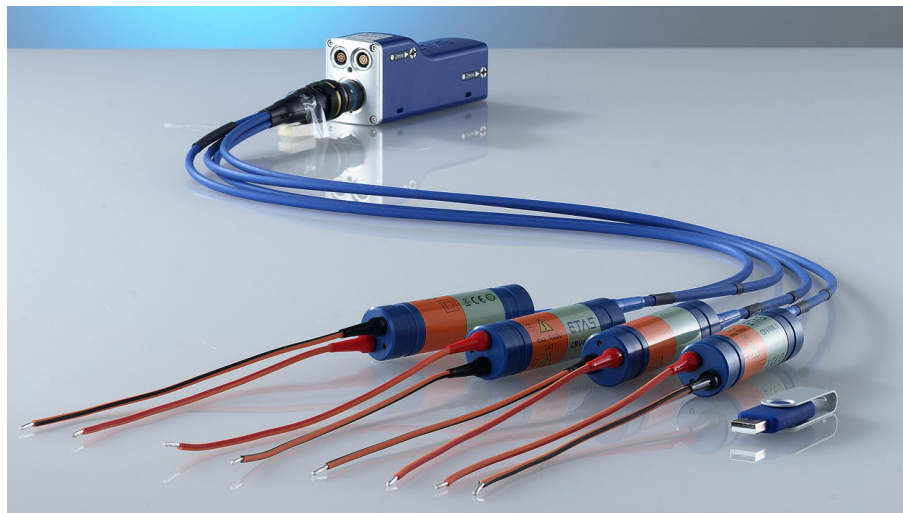
Abb. 2-1 CBN401.1 mit ES411.1 A/D-Modul
