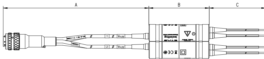
Abb. 3-1 Abmessungen
