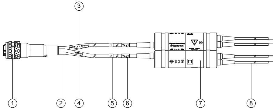
Abb. 2-2 Aufbau der Isolierenden Messsonde
