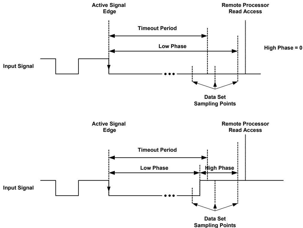
Abb. 17-48 Frequenz- und Zykluszeitmessungen: Messwert im Timeout-Fall beim Modus „Intvl InpDep“ zur Timeout-Überwachung
