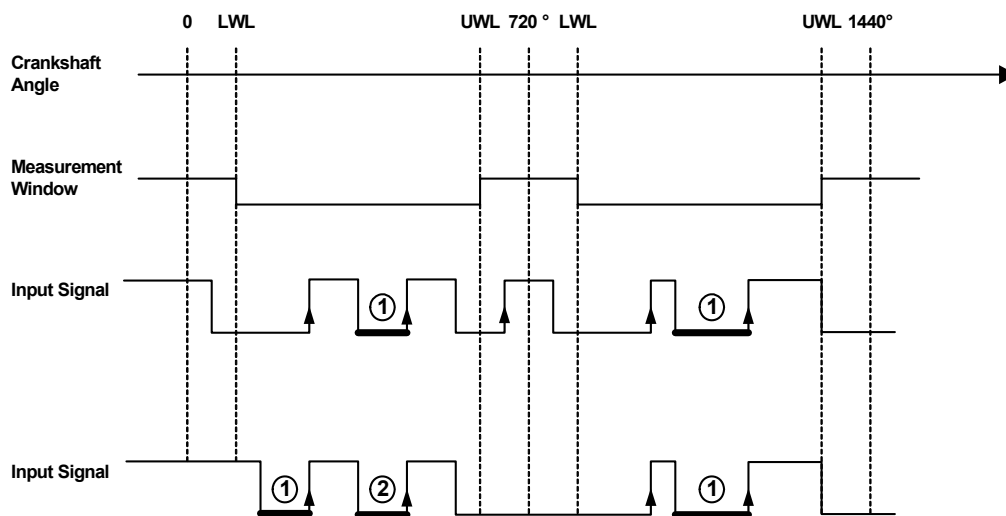
Abb. 12-20 Darstellung der Funktionsweise einer puls-qualifizierten, low-aktiven Pulsweitenmessung (Messverfahren Angular: L-Time n-th Pulse (Pu Qual.) [ \mu s]). Vermessene Pulse bzw. Pulse die gezählt werden sind mit erhöhter Linienstärke hervorgehoben.
