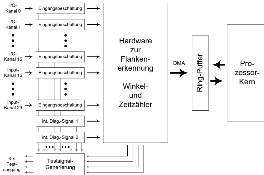
Abb. 33-22 Blockschaltbild TMIO-Karte
