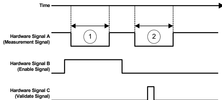
Abb. 12-21 Pulsweitenmessungen mit Enable- und Validierungssignal
