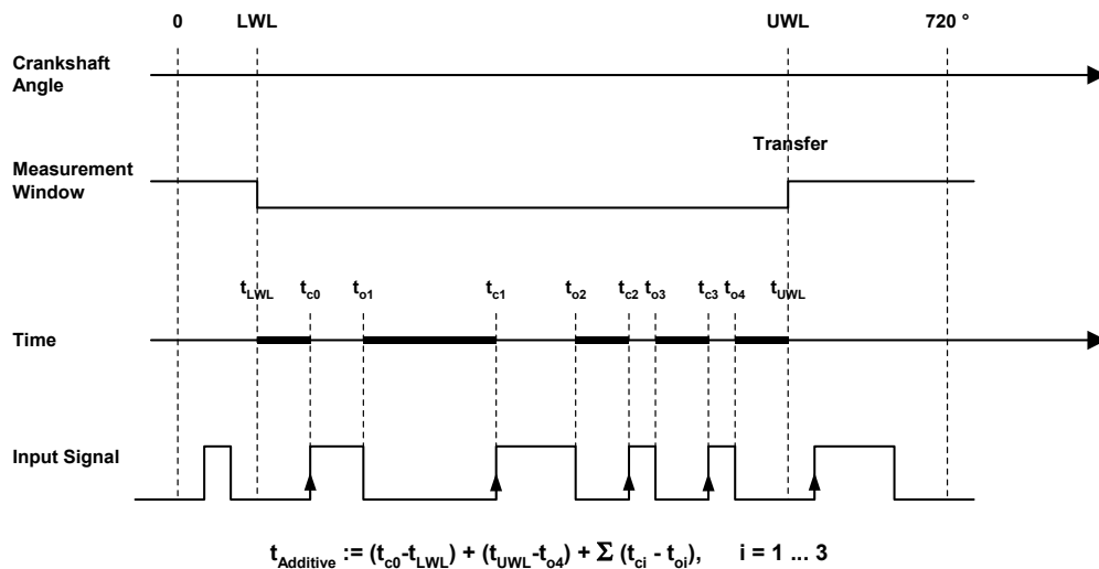
Abb. 9-17 Darstellung der Funktionsweise einer drehzahlsynchronen additiven Lowzeit-Messung (Messverfahren „Additive Lowtime [µs]“). Die additive Zeit setzt sich aus der Summe der fett markierten Linien-segmente zusammen.
