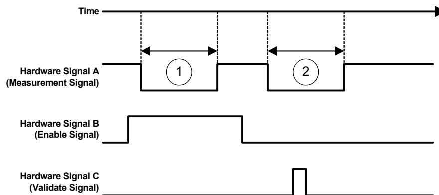
Abb. 18-46 Validierte Zeitmessungen mit der ES4330-Karte
