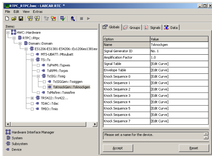
Abb. 33-17 Die Registerkarte „Globals“ des TsKnockGen Devices
