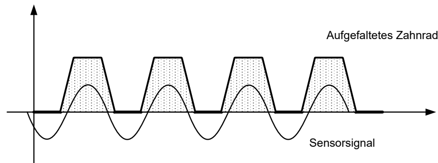
Abb. 7-2 Das Sensorsignal eines passiven Drehzahlfühlern
