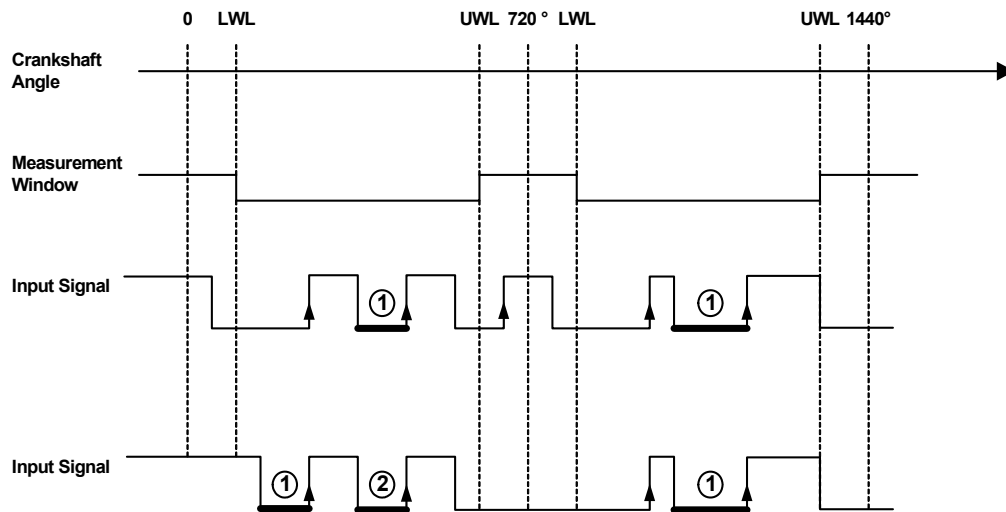
Abb. 24-29 Darstellung der Funktionsweise einer puls-qualifizierten, low-aktiven Pulsweitenmessung (Messverfahren Angular: L-Time n-th Pulse (Pu Qual.) [ \mu s]). Vermessene Pulse bzw. Pulse die gezählt werden sind mit erhöhter Linienstärke hervorgehoben.
