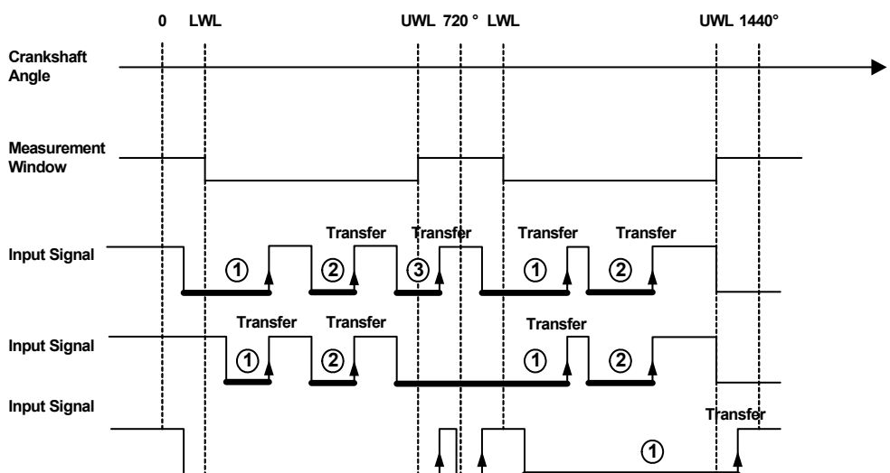
Abb. 10-16 Darstellung der Funktionsweise einer flanken-qualifizierten, low-aktiven Pulsweitenmessung (Messverfahren „Lowtime (Edge Qual.) [µs]“). Vermessene Pulse sind mit erhöhter Linienstärke hervorgehoben. Die Zuordnung der Pulse zu den Winkelfenstern und die Zählung der Pulse innerhalb eines Winkelfensters ist ebenfalls dargestellt.
