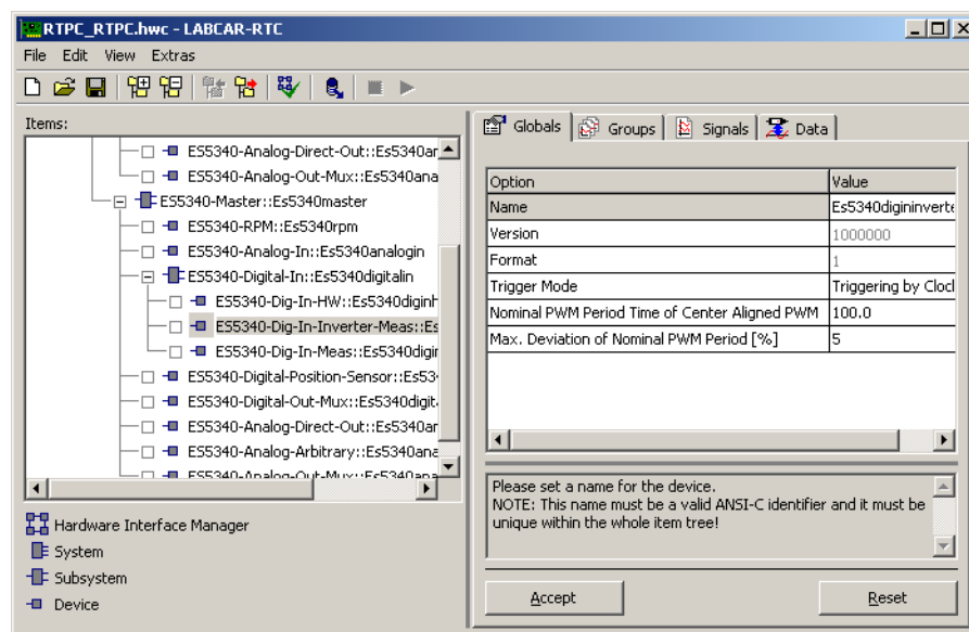
Abb. 23-20 Die Registerkarte „Globals“ des ES5340-Dig-In-Inverter-Meas Device (Ansichtsoption „Show All“)
