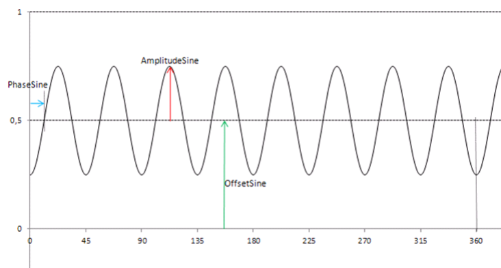
Abb. 23-40 Sine-Encoder: Sinuskanal
