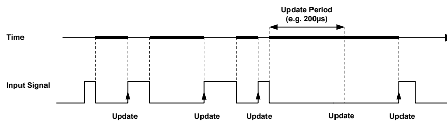
Abb. 18-45 Darstellung der Funktionsweise einer asynchronen additiven Lowzeit-Messung (Messverfahren „Additive Lowtime [ \mu\text{s} ]“). Die additive Zeit setzt sich aus den fett markierten Zeitsegmenten zusammen. Die Zeitpunkte an denen die Summe im DPRAM aktualisiert wird, sind ebenfalls dargestellt.
