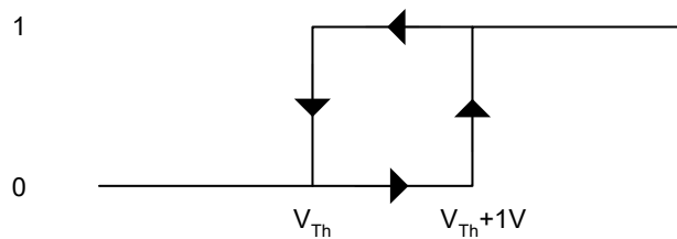
Abb. 9-3 Komparator-Hysterese. V_{Th} bezeichnet den eingestellten Schwellwert.
