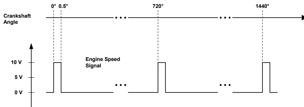
Abb. 9-9 Synchronisationssignal auf den Nulldurchgang des Nockenwellenwinkels.
