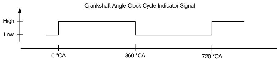
Abb. 12-14 Winkeltakt-Phasen-Indikator-Signal
