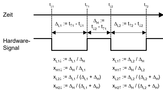
Abb. 33-28 Tastverhältnis-Bestimmung mit TMIO-Karte.
