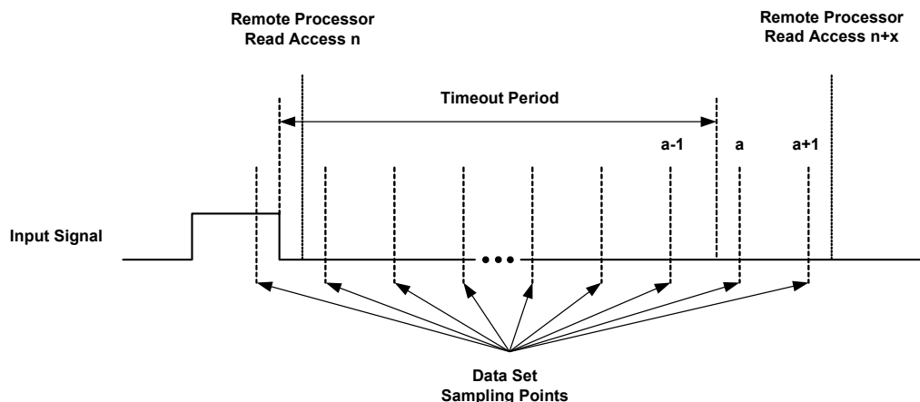
Abb. 17-44 Timeouts bei additiven Pulsweitenmessungen
