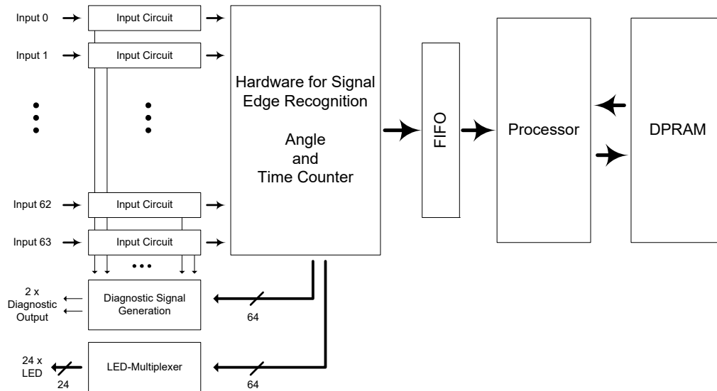
Abb. 18-31 Blockschaltbild der ES4330-Karte
