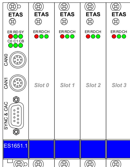
Abb. 17-33 Nummerierung der Modul-Steckplätze eines ES1651.1 Carrier Board
