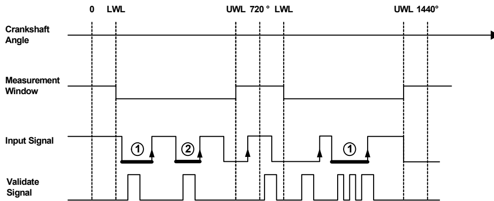
Abb. 12-23 Darstellung der Funktionsweise einer winkelsynchronen Pulsweitenmessung mit Validierungssignal (Messverfahren „Angular: L-Time n-th Pulse (H-Valid.) [µs]“). Validierte Pulse sind mit erhöhter Linienstärke hervorgehoben.
