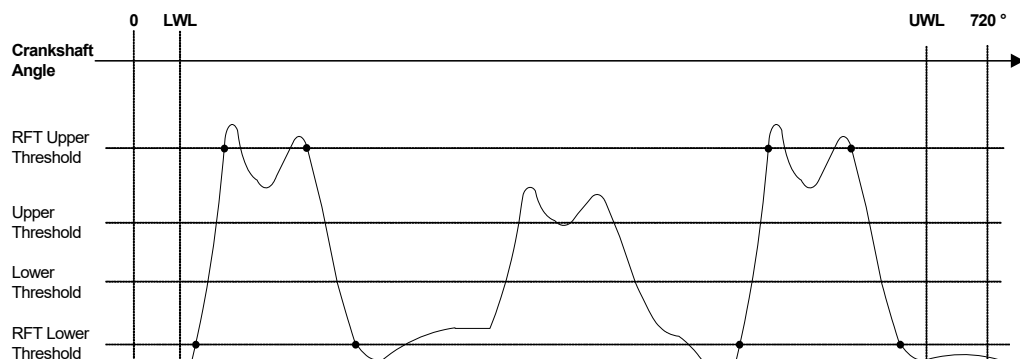
Abb. 12-26 Flankenmessung bei Vermessung von Anstiegs- und Abfallzeiten
