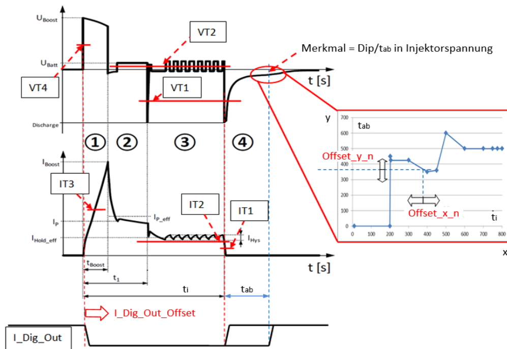
Abb. 26-4 Typischer HDEV5 CVO-Injektorstrom-/Injektorspannungsverlauf mit Merkmal und „I_Dig_Out“ Signal
