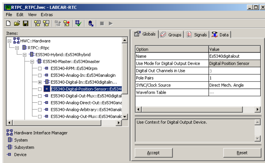
Abb. 23-26 Die Registerkarte „Globals“ des ES5340-Digital-Position-Sensor RTIO-Elements
