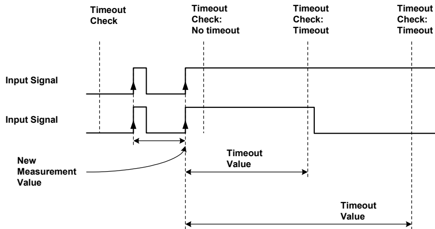
Abb. 18-50 Frequenz- und Zykluszeitmessungen an ansteigenden Flanken: Darstellung der Messwertberechnung im Timeout-Fall (der Messwert ist in der Darstellung als „Timeout Value“ bezeichnet) bei den „... InpDep“-Verfahren zur Timeout-Überwachung
