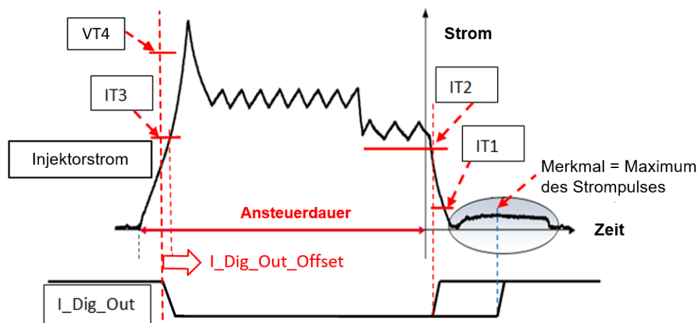
Abb. 31-2 Typischer CRI2X Injektorstromverlauf mit Merkmal (graue Ellipse) und „I_Dig_Out“ Signal
