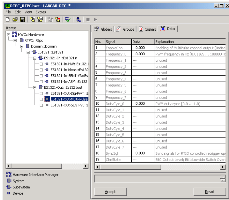
Abb. 5-28 Die Registerkarte „Data“ des ES1321-Multi-Pulse Devices
