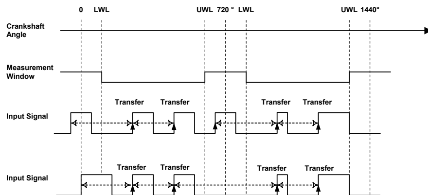
Abb. 18-49 Darstellung der Messwertberechnung bei einer winkelsegmentierten Frequenz- oder Zykluszeitmessung an steigenden Signalfanken
