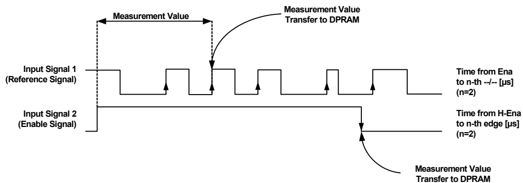
Abb. 10-24 Funktionsweise der Messverfahren zur Vermessung von Ereignissen (Flanken) auf unterschiedlichen Signalen bzw. Hardwarekanälen relativ zueinander. Dargestellt ist eine Messung mit high-aktivem Enable-Signal. Der RTIO-Parameter zur Flankenselektion („(Max) Pulse (Count)“ in der Registerkarte „Signals“) ist größer als 0.
