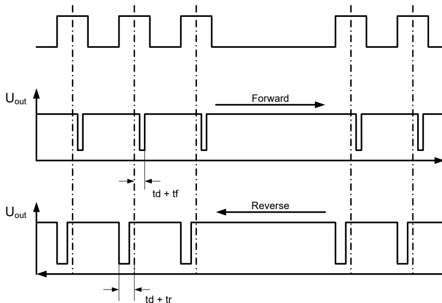
Abb. 24-48 Kurbelwellenzähne und Sensorsignale bei einem MSA-Sensor
