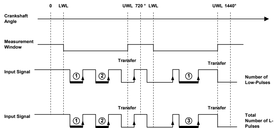
Abb. 18-55 Darstellung der Funktionsweise drehzahlsynchroner Messverfahren zur Pulszählung (Messverfahren „Number of Low-Pulses“ und „Total Number of L-Pulses“). Pulse die gezählt wurden sind durch erhöhte Linienstärke hervorgehoben. Die Summe wird jeweils an der oberen Winkelfenstergrenze in das DPRAM transferiert.
