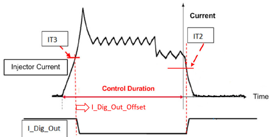
Abb. 26-6 Typischer Injektor-Stromverlauf für ES4455.2-Generic-Load-Carrier-(Legacy-Mode) und I_Dig_Out-Signal.
