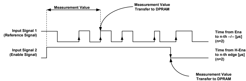
Abb. 18-51 Funktionsweise der Messverfahren zur Vermessung von Ereignissen (Flanken) auf unterschiedlichen Signalen bzw. Hardwarekanälen relativ zueinander. Dargestellt ist eine Messung mit high-aktivem Enable-Signal. Der RTIO-Parameter zur Flanken-Selektion („(Max) Pulse (Count)“ in der Registerkarte „Signals“) ist größer als 0.
