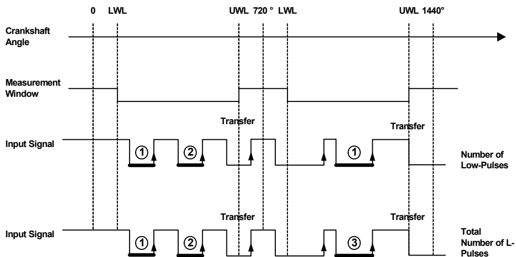
Abb. 10-28 Darstellung der Funktionsweise winkelsynchroner Messverfahren zur Pulszählung (Messverfahren „Number of Low-Pulses“ und „Total Number of L-Pulses“). Pulse, die gezählt werden, sind durch erhöhte Linienstärke hervorgehoben. Die Summe wird jeweils an der oberen Winkelfenstergrenze in das DPRAM transferiert.
