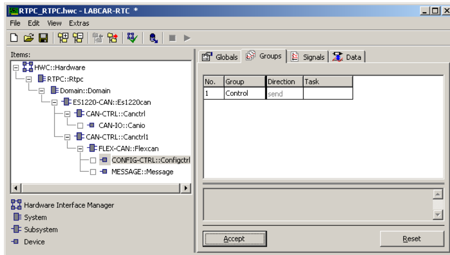
Abb. 3-4 Die Registerkarte „Groups“ des CONFIG-CTRL Devices
