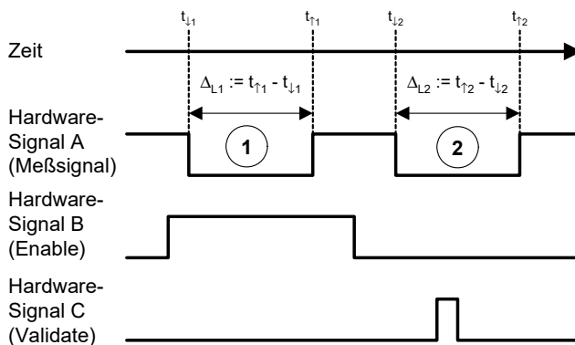
Abb. 33-29 Validierte Zeitmessungen mit TMIO-Karte
