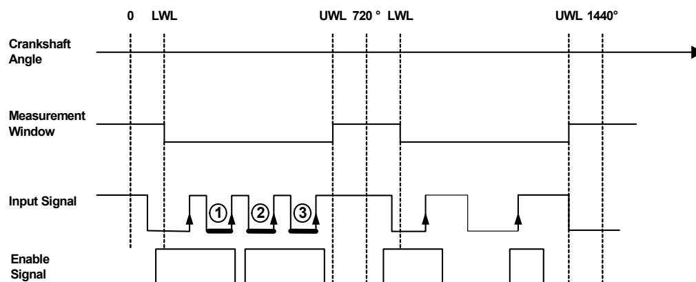
Abb. 12-22 Darstellung der Funktionsweise einer winkelsynchronen Pulsweitenmessung mit Enable-Signal (Messverfahren „Angular: L-Time n-th Pulse (H-Enable) [µs]“). Aktivierte Pulse sind mit erhöhter Linienstärke hervorgehoben.
