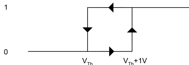
Abb. 10-3 Komparator-Hysterese. V_{Th} bezeichnet den eingestellten Schwellwert
