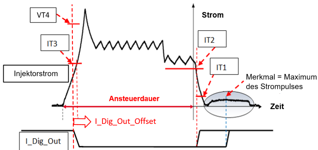
Abb. 19-20 Typischer CRI2-x Injektorstromverlauf mit Merkmal (graue Ellipse) und „I_Dig_Out“ Signal
