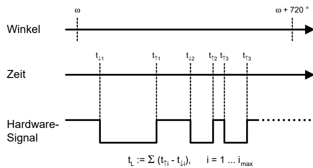
Abb. 33-25 Additive Zeitmessungen mit TMIO-Karte
