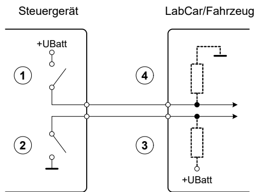
Abb. 18-33 Notwendigkeit von Pull-Up- / Pull-Down-Beschaltungen
