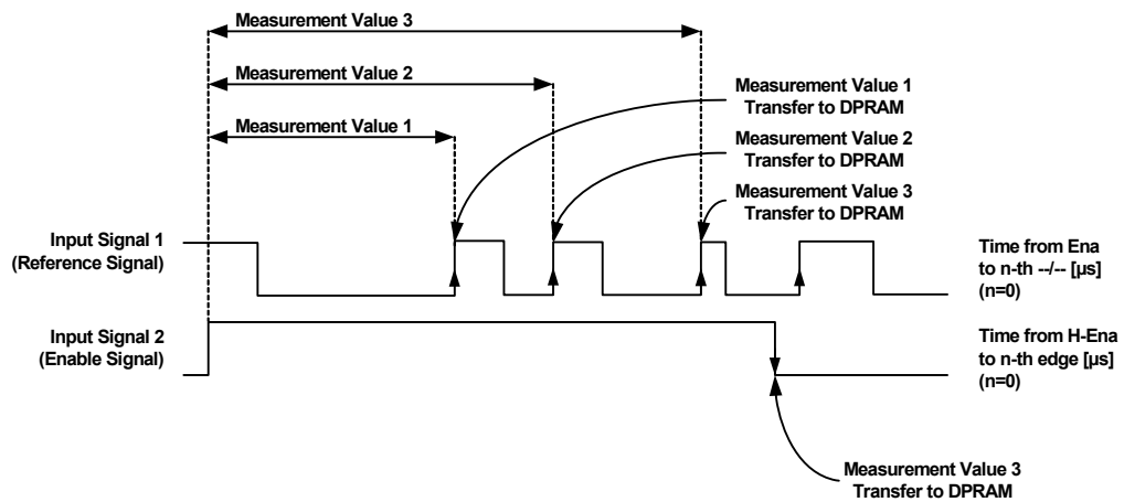
Abb. 10-26 Funktionsweise der Messverfahren zur Vermessung von Ereignissen (Flanken) auf unterschiedlichen Signalen bzw. Hardwarekanälen relativ zueinander. Dargestellt ist eine Messung mit high-aktivem Enable-Signal. Der RTIO-Parameter zur Flanken-Selektion („(Max) Pulse (Count)“ in der Registerkarte „Signals“) ist gleich 0.
