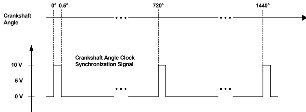
Abb. 10-9 Synchronisationssignal auf den Nulldurchgang des Nockenwellenwinkels
