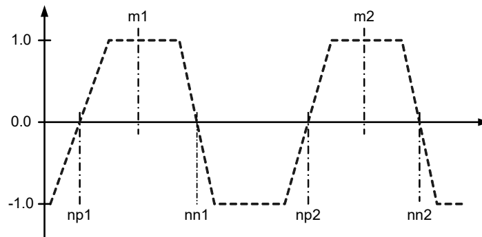
Abb. 24-49 Mittenpositionsberechnung (bei nicht ganz symmetrischem Zahnverlauf und positiver Logik)
