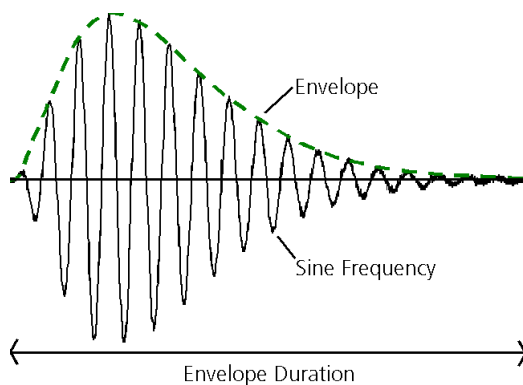
Abb. 33-16 Klopfsignal (durchgezogen) und Einhüllende (gestrichelt)
