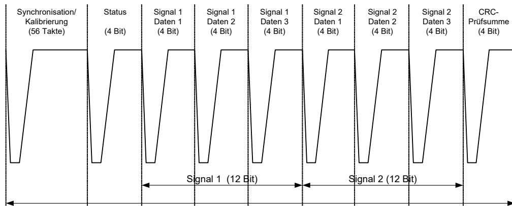
Abb. 5-14 Format eines Signals gemäß SENT-Datenprotokoll
