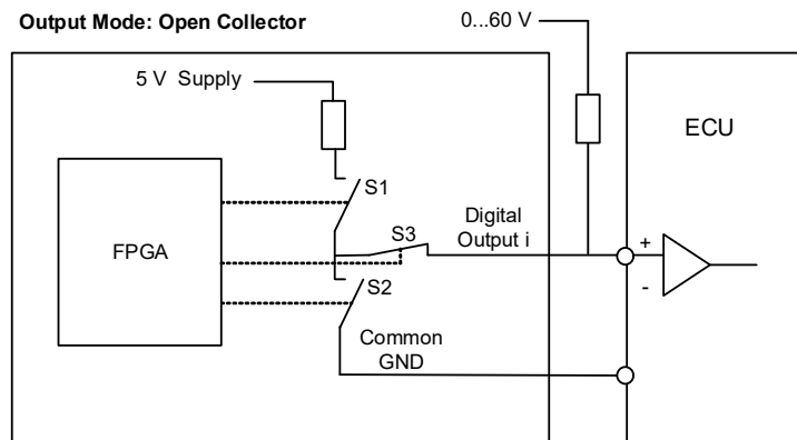
Abb. 23-34 Prinzipschaltbild für die beiden Einstellungen „Pull-Up to +5 V“ und „Open Collector“ in der Registerkarte „Signals“
