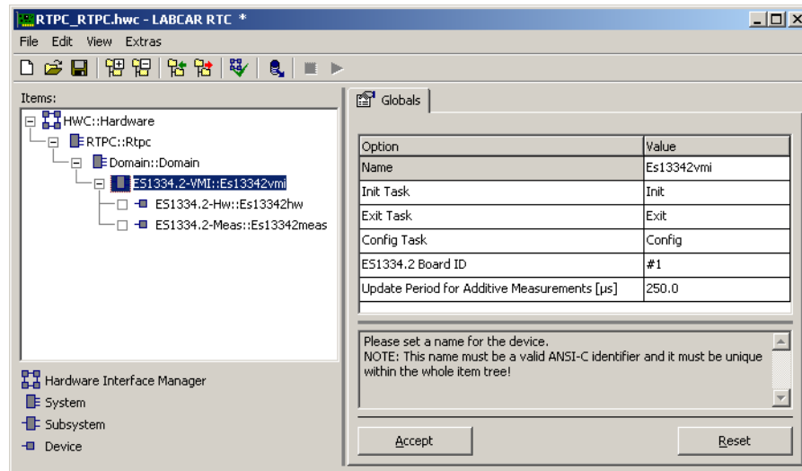
Abb. 10-6 Die Registerkarte „Globals“ des ES1334.2-VMI-Subsystems
