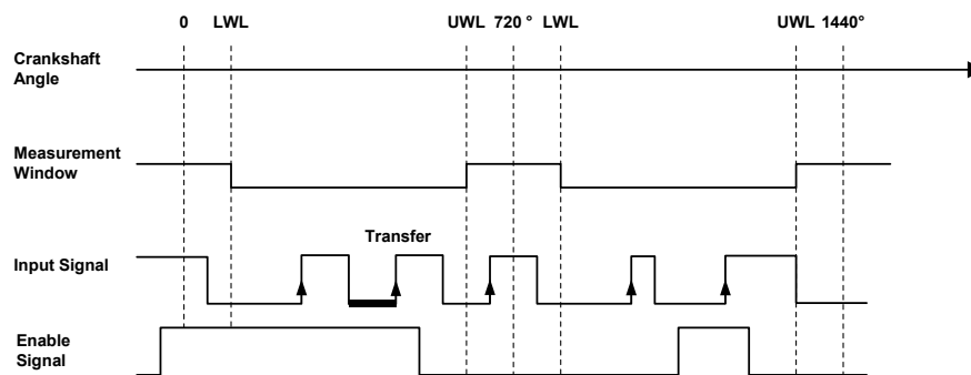
Abb. 18-47 Darstellung der Funktionsweise einer drehzahlsynchronen Pulsweitenmessung mit Enable-Signal (Messverfahren „Lowtime using H-Enable [μs]“). Vermessene Pulse sind mit erhöhter Linienstärke hervorgehoben.
