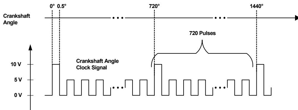
Abb. 10-8 Winkeltaktsignal zur Synchronisation auf den Nulldurchgang des Nockenwellenwinkels und Berechnung der Winkelstellung des Motors
