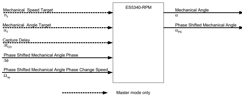
Abb. 23-7 Steuer- und Statussignale der Drehzahleinheit bei der Simulation von Elektromotoren im Master-Betrieb mit Winkeladaption
