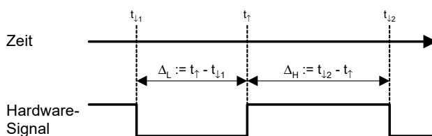
Abb. 33-24 Zeitmessungen mit TMIO-Karte
