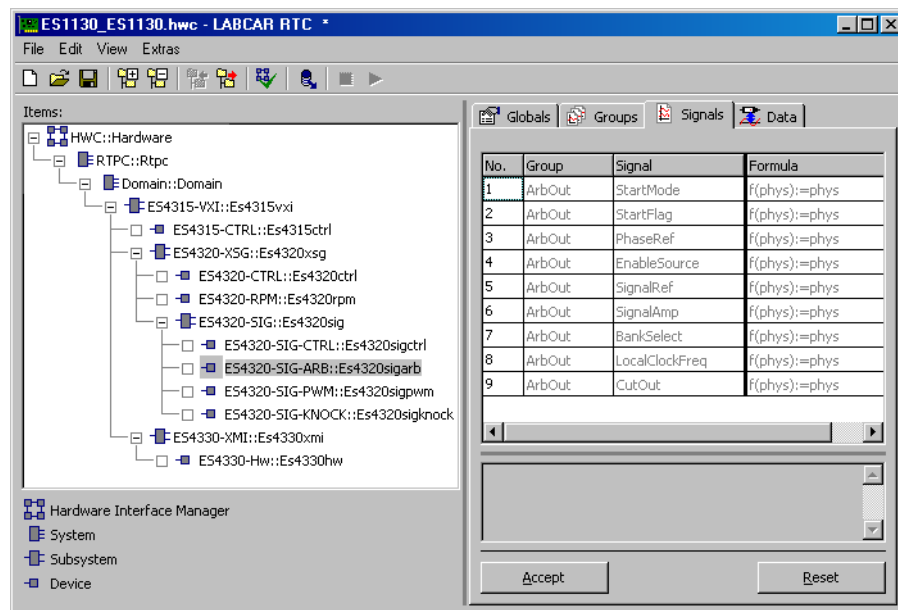
Abb. 18-19 Die Registerkarte „Signals“ des ES4320-SIG-ARB Devices
