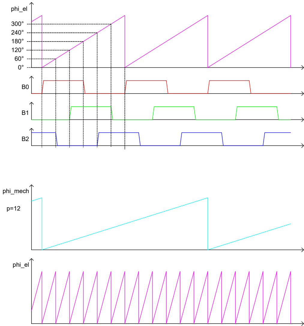
Abb. 23-25 Digital Position Sensor – Signalverläufe
