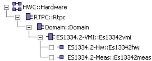
Abb. 10-5 RTIO-Hardwarebeschreibung mit eingebundener ES1334.2
