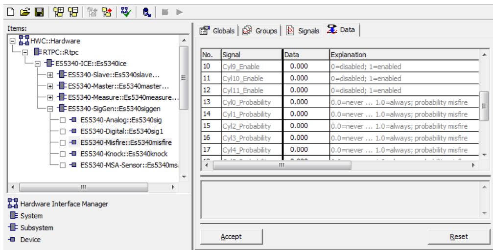
Abb. 24-44 Die Registerkarte „Data“ des ES5340-Misfire Device
