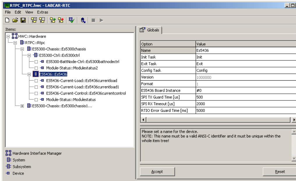
Abb. 30-3 Die Registerkarte "Globals" des ES5436 Subsystems (alle Optionen sichtbar)
