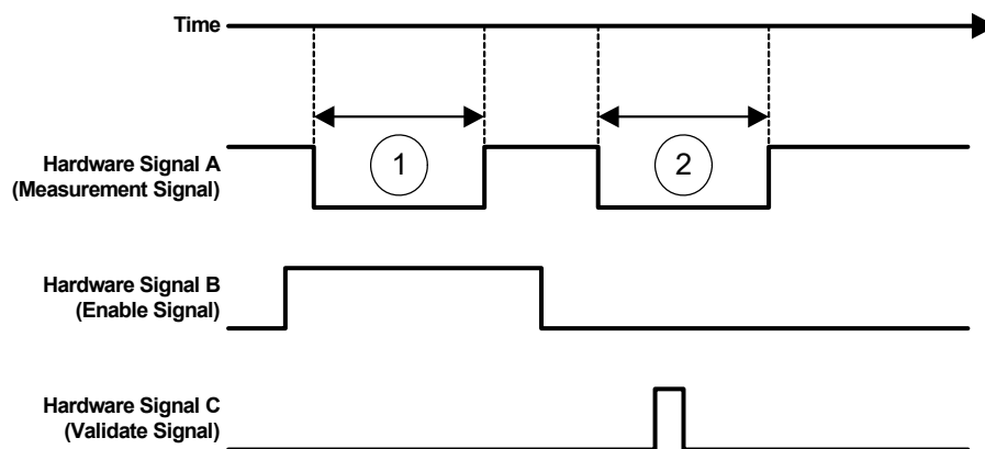
Abb. 10-19 Validierte Zeitmessungen mit der ES1334.2
