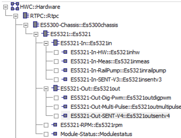
Abb. 21-1 Vollständiger RTIO-Baum für das ES5321.1 PWM I/O Board
