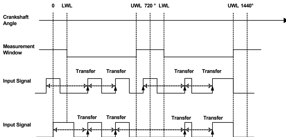
Abb. 10-22 Darstellung der Messwertberechnung bei einer winkelsegmentierten Frequenz- oder Zykluszeitmessung an steigenden Signalfanken
