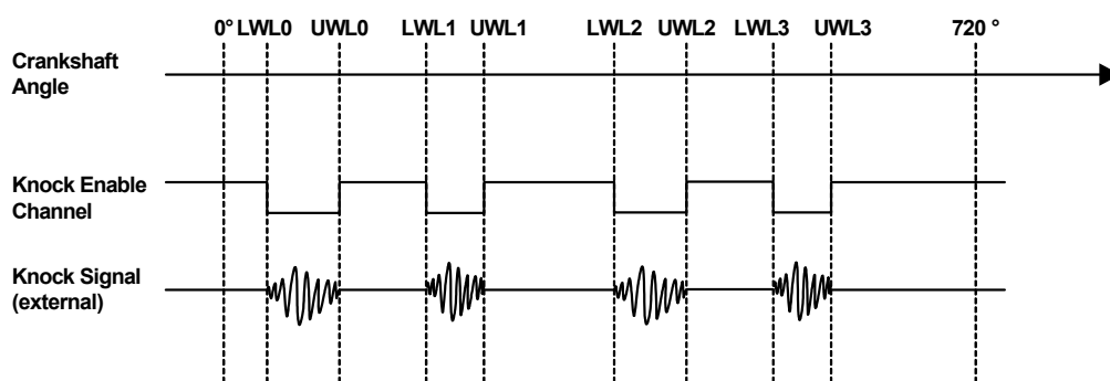
Abb. 10-4 Low-aktives Klopf-Enable-Signal zur Aktivierung und Deaktivierung eines externen Klopf-Generators
