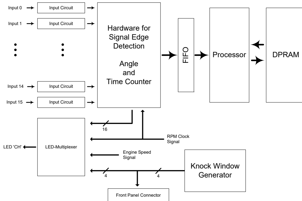
Abb. 10-1 Blockschaltbild des ES1334.2 Measurement Board
