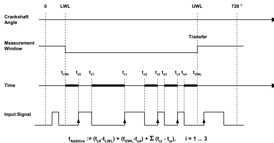
Abb. 18-44 Darstellung der Funktionsweise einer drehzahlsynchronen additiven Lowzeit-Messung (Messverfahren „Additive Lowtime [µs]“). Die additive Zeit setzt sich aus der Summe der fett markierten Linien-segmente zusammen.
