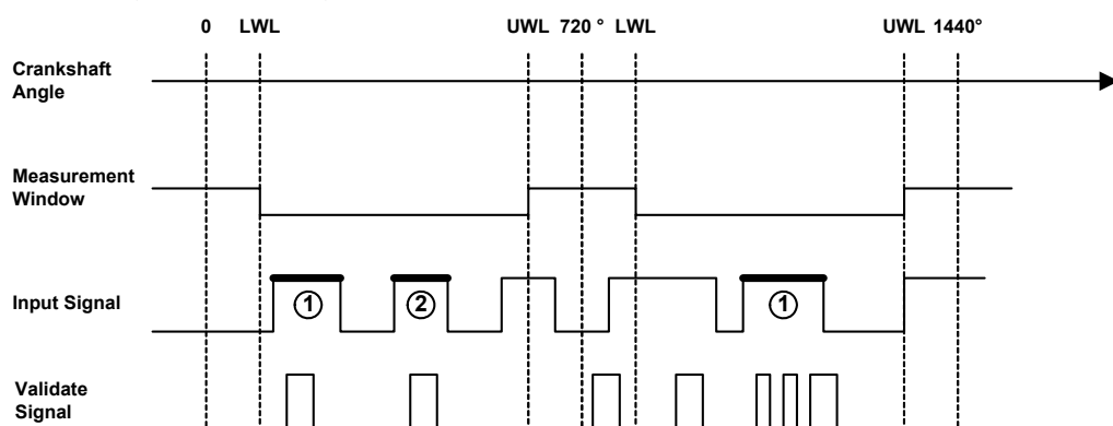
Abb. 24-30 Darstellung der Funktionsweise einer winkelsynchronen Pulsweitenmessung mit Validierungssignal (Messverfahren „Angular: H-Time n-th Pulse (H-Valid.) [µs]“). Validierte Pulse sind mit erhöhter Linienstärke hervorgehoben.
