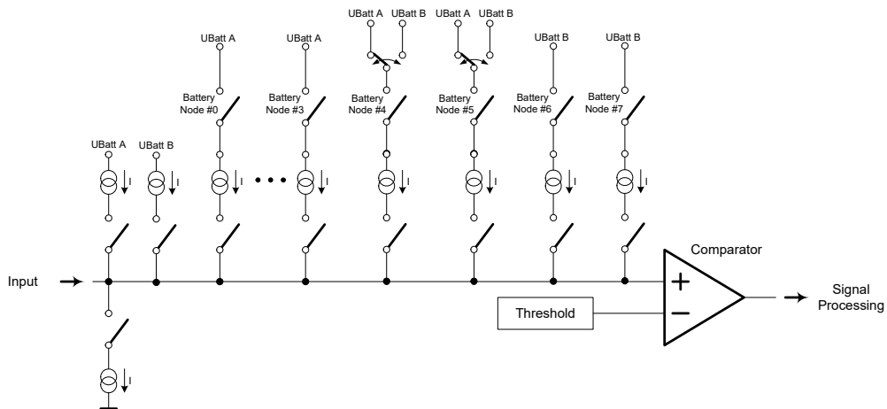
Abb. 18-32 Vereinfachte Darstellung der Eingangsbeschaltung eines ES4330 Hardwarekanals
