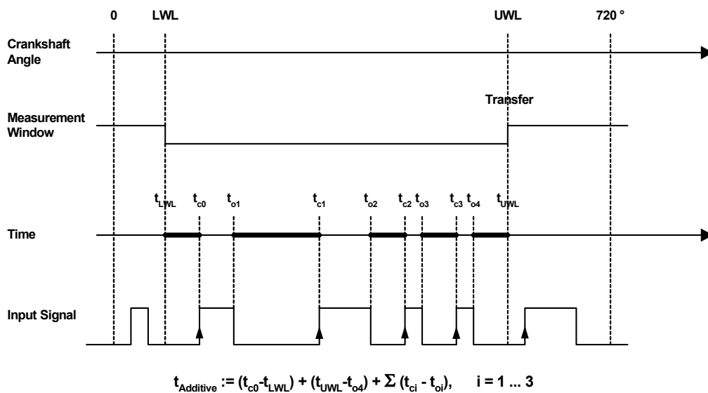
Abb. 12-24 Darstellung der Funktionsweise einer winkelsynchronen additiven Lowzeit-Messung (Messverfahren Angular: Additive Lowtime [µs]). Die additive Zeit setzt sich aus der Summe der fett markierten Liniensegmente zusammen.
