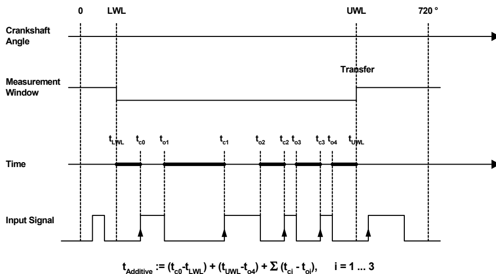
Abb. 24-31 Darstellung der Funktionsweise einer winkelsynchronen additiven Lowzeit-Messung (Messverfahren Angular: Additive Lowtime [µs]). Die additive Zeit setzt sich aus der Summe der fett markierten Liniensegmente zusammen.
