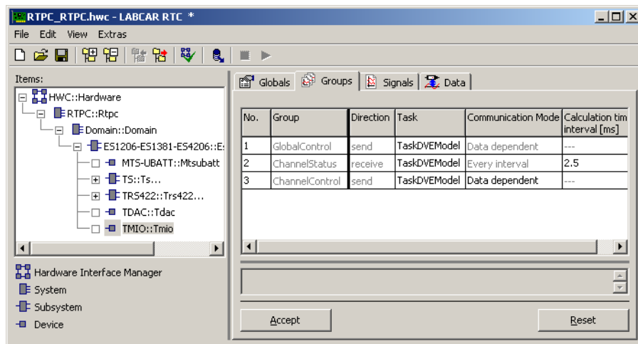
Abb. 33-32 Die Registerkarte „Groups“ des TMIO Devices
