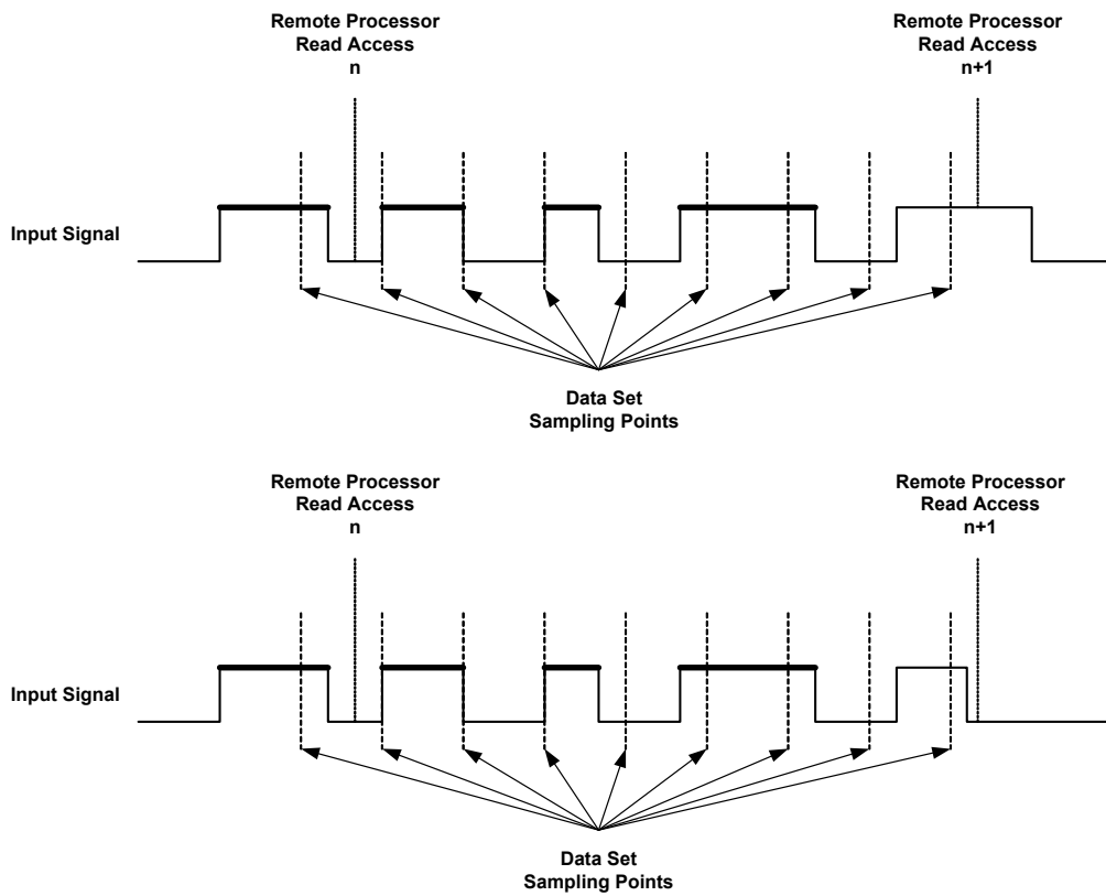
Abb. 5-10 High-Puls-Zählung: Die Anzahl der mit fetter Strichstärke markierten Pulse wird beim (n+1)-ten Lesevorgang als Messwert zurückgegeben
