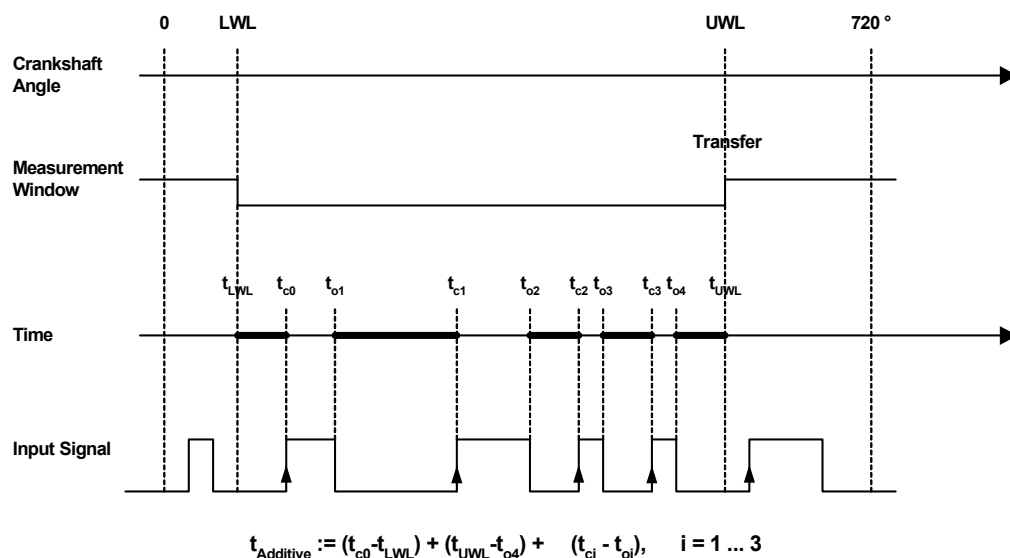
Abb. 10-17 Darstellung der Funktionsweise einer winkelsynchronen additiven Lowzeit-Messung (Messverfahren „Additive Lowtime [µs]“). Die additive Zeit setzt sich aus der Summe der fett markierten Linien-segmente zusammen.
