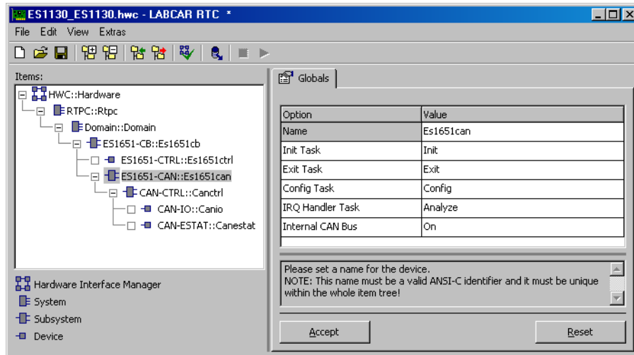
Abb. 17-9 Die Registerkarte „Globals“ des ES1651-CAN Subsystems
