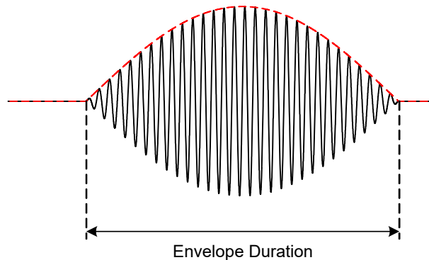
Abb. 24-38 Ein Klopfpaket
