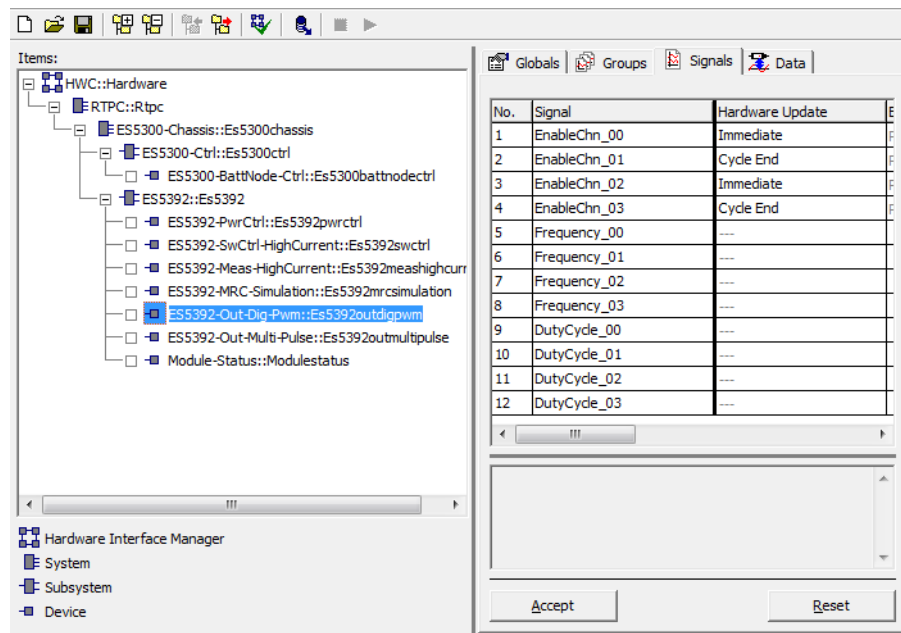
Abb. 28-14 Die Registerkarte „Signals“ des ES5392-Out-Dig-Pwm Device
