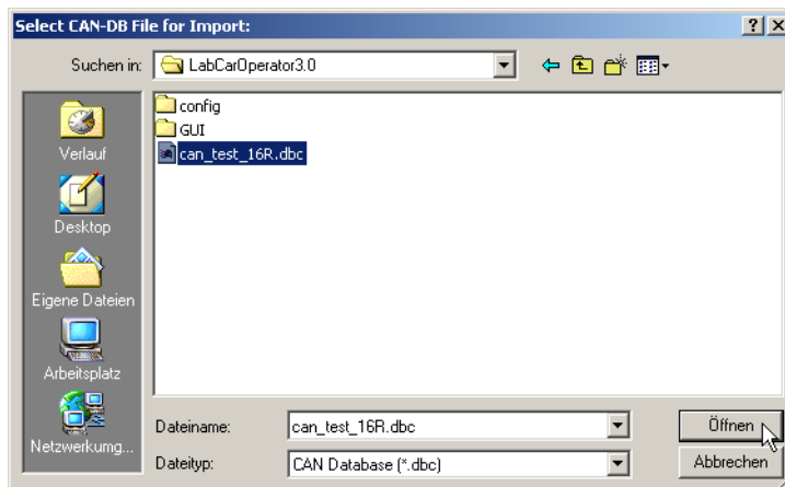
Abb. 32-6 CANdb Auswahl
