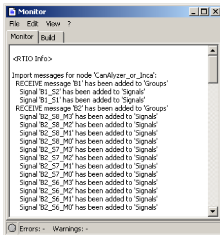
Abb. 32-9 CANdb Importprotokoll
