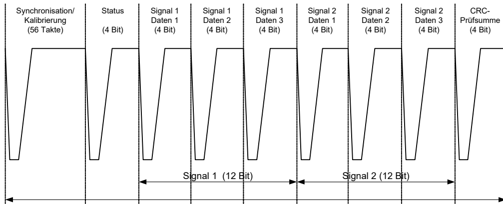
Abb. 21-15 Format eines Signals gemäß SENT-Datenprotokoll
