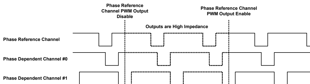
Abb. 17-52 Aktivierung und Deaktivierung der PWM-Ausgabe von Kanälen, die in einem definierten Phasenbezug zueinander stehen
