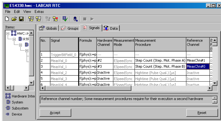
Abb. 18-56 Konfiguration einer Messung zur Positionsverfolgung an zwei-phasigen Schrittmotoren
