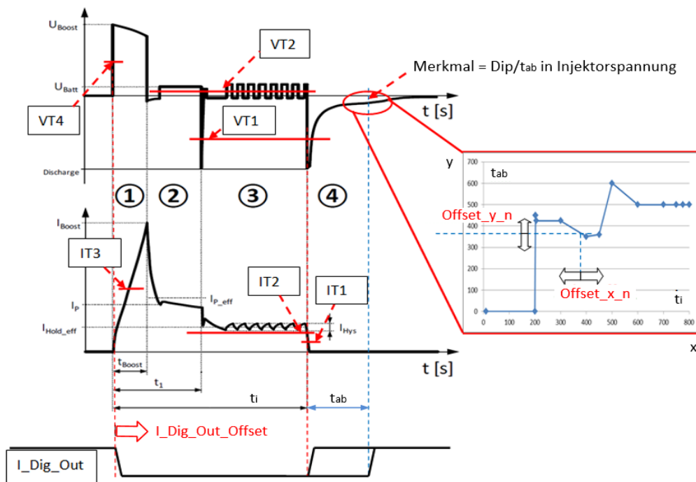
Abb. 31-1 Typischer HDEV5/HDEV6 CVO-Injektorstrom-/Injektorspannungsverlauf mit Merkmal und I_Dig_Out-Signal Rot umrandetes Insert: Interpolierter Graph aus Valve-Closing-Delay-Table t_{ab} : Schließ-Verzögerungszeit nach Ansteuerende = Verzögerungszeit nach Ansteuerende für das Auftreten des Merkmals t_i : Ansteuerdauer des Injektors
