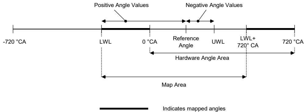
Abb. 9-21 Funktionsweise einer Winkelmessung im drehzahlsynchronen Messmodus
