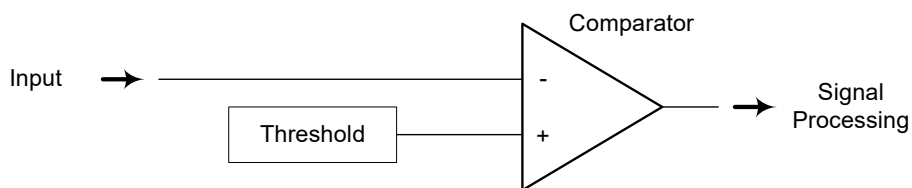
Abb. 9-2 Vereinfachte Darstellung der Eingangsbeschaltung eines ES1334.1-Hardwarekanals.
