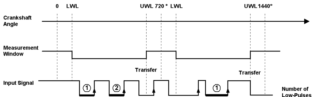
Abb. 9-22 Darstellung der Funktionsweise drehzahlsynchroner Messverfahren zur Pulszählung (Messverfahren „Number of Low-Pulses“). Pulse, die gezählt werden, sind durch erhöhte Linienstärke hervorgehoben. Die Summe wird jeweils an der oberen Winkelfenstergrenze in das DPRAM transferiert.
