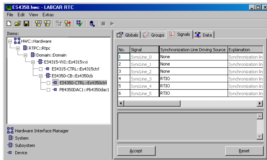
Abb. 18-64 Die Registerkarte „Signals“ des ES4350-CTRL Devices
