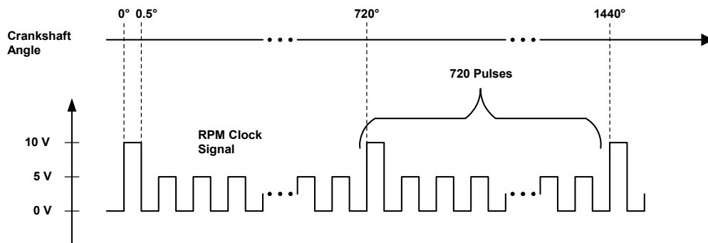
Abb. 9-8 Winkeltaktsignal zur Synchronisation auf den Nulldurchgang des Nockenwellenwinkels und Berechnung der Winkelstellung des Motors
