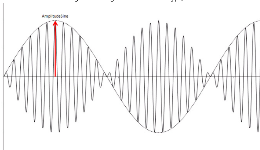
Abb. 23-44 Resolver: Sinuskanal
