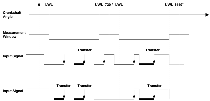
Abb. 18-42 Darstellung der Funktionsweise einer puls-qualifizierten low-aktiven Pulsweitenmessung (Messverfahren „Lowtime (Pulse Qual.) [µs]“). Vermessene Pulse sind mit erhöhter Linienstärke hervorgehoben.
