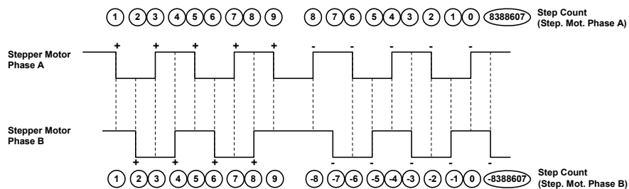
Abb. 18-57 Darstellung der Arbeitsweise der Positionsverfolgung an zwei-phasigen Schrittmotoren
