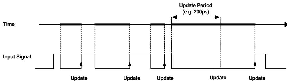
Abb. 10-18 Darstellung der Funktionsweise einer asynchronen additiven Lowzeit-Messung (Messverfahren „Additive Lowtime [ \mu\text{s} ]“). Die additive Zeit setzt sich aus den fett markierten Zeitsegmenten zusammen. Die Zeitpunkte an denen die Summe im DPRAM aktualisiert wird, sind ebenfalls dargestellt.
