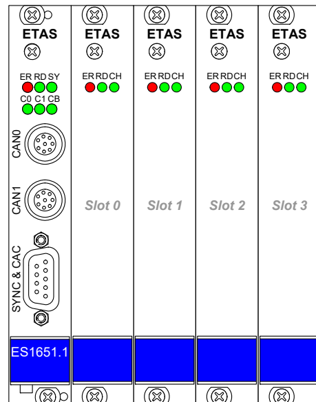
Abb. 17-25 Nummerierung der Modulsteckplätze eines ES1651.1 Carrier Board
