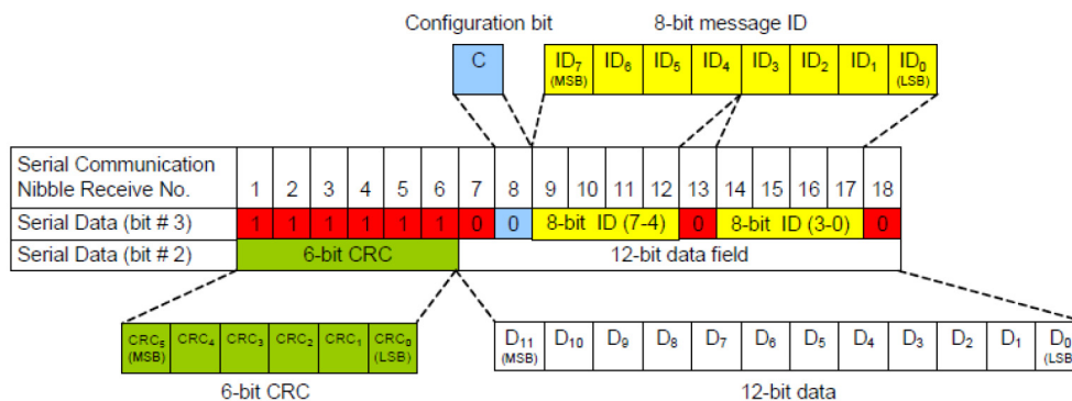
Abb. 21-16 Enhanced Serial Message Format mit 12-Bit Data Field und 8-Bit Message ID
