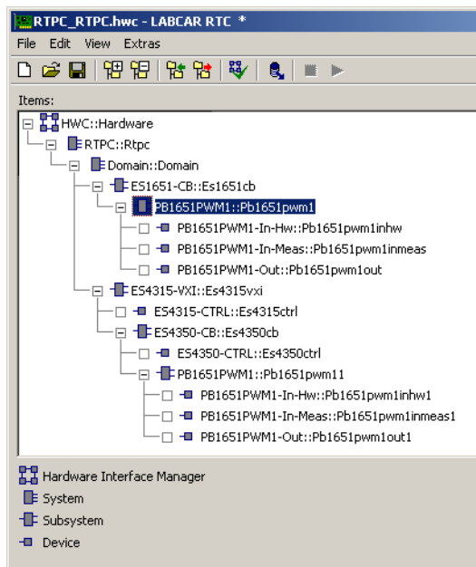
Abb. 17-31 RTIO-Hardwarebeschreibung mit eingebundenen PB1651PWM1-Modulen
