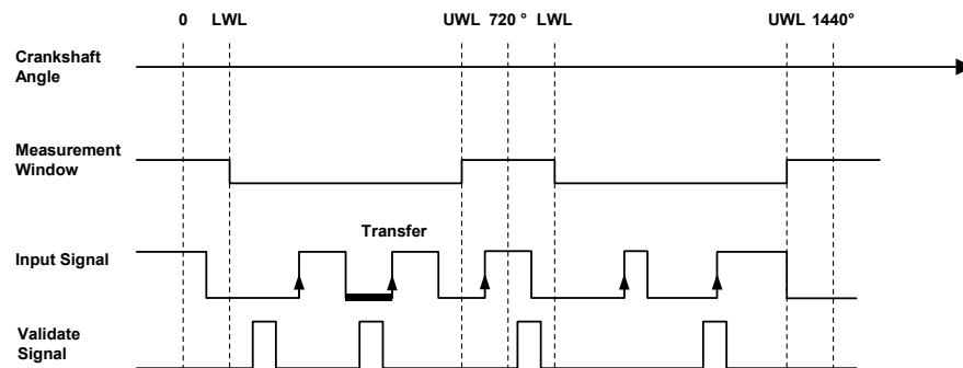
Abb. 18-48 Darstellung der Funktionsweise einer drehzahlsynchronen Pulsweitenmessung mit Validate-Signal (Messverfahren „Lowtime using H-Validate [ \mu\text{s} ]“). Vermessene Pulse sind mit erhöhter Linienstärke hervorgehoben.
