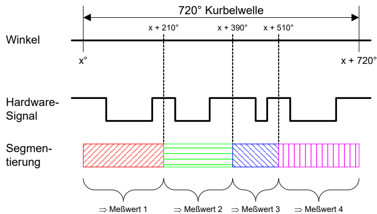
Abb. 33-30 Winkelsegmentierung mit TMIO-Karte
