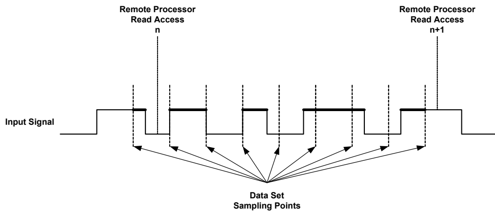
Abb. 5-9 Additive High-Zeit-Messung: Illustration der Messwertberechnung Eine Timeout-Bedingung liegt dann vor, wenn mindestens eine der vier Flanken älter ist als der aktuelle Zeitstempel abzüglich der Timeout-Zeit.
