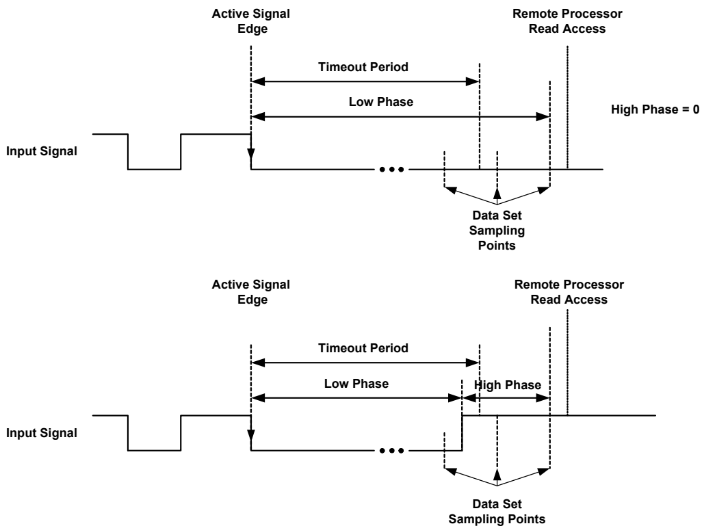
Abb. 17-49 Tastverhältnismessungen an fallenden Flanken: Bestimmung der High-Phase und Low-Phase des Signals im Timeout-Fall
