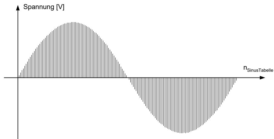
Abb. 7-3 Darstellung der Sinuswelle im Datenspeicher des DSP-Prozessors
