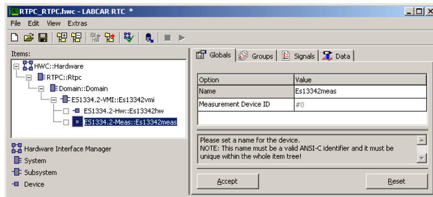
Abb. 10-12 Die Registerkarte „Globals“ des ES1334.2-Meas Device
