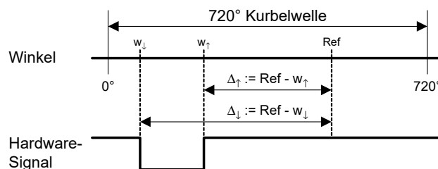
Abb. 33-23 Winkelmessungen mit der TMIO-Karte
