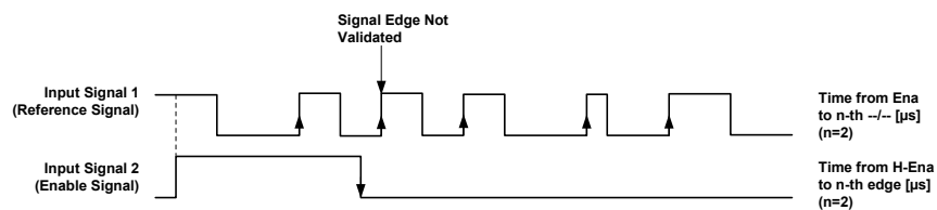
Abb. 18-52 Vermessung von Flanken auf unterschiedlichen Hardwarekanälen: Signalverlauf mit high-aktivem Enable-Signal und nicht validierter aktiver Signalfanke des Referenz-Signals.
