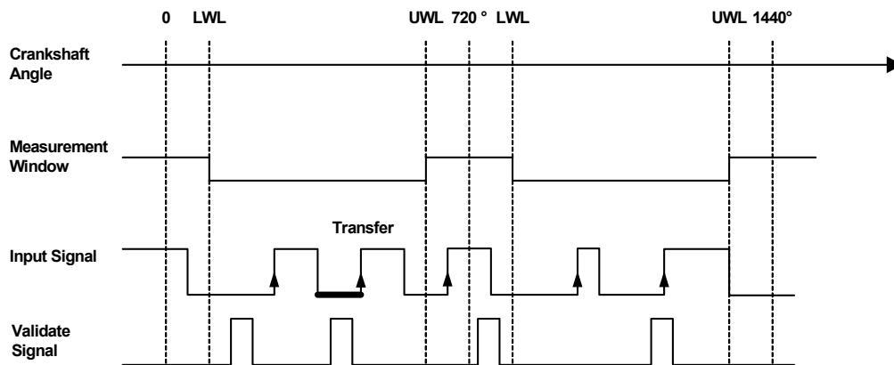
Abb. 10-21 Darstellung der Funktionsweise einer winkelsynchronen Pulsweitenmessung mit Validate-Signal (Messverfahren „Lowtime using H-Validate [ \mu\text{s} ]“). Vermessene Pulse sind mit erhöhter Linienstärke hervorgehoben.
