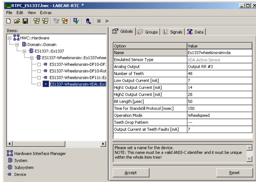
Abb. 13-15 Die Registerkarte „Globals“ des ES1337-Wheelsnsrsim-VDA Device
