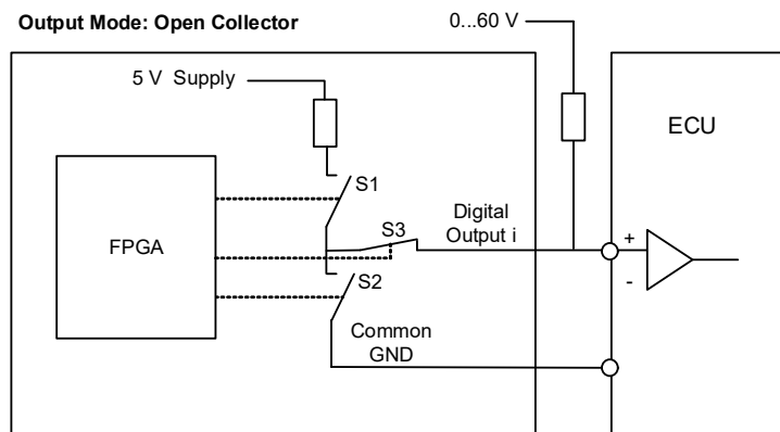
Abb. 24-13 Prinzipschaltbild für die beiden Einstellungen „Pull-Up to +5 V“ und „Open Collector“ in der Registerkarte „Signals“
