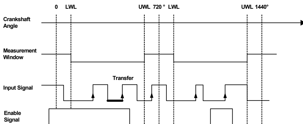
Abb. 10-20 Darstellung der Funktionsweise einer winkelsynchronen Pulsweitenmessung mit Enable-Signal (Messverfahren „Lowtime using H-Enable [ \mu\text{s} ]“). Vermessene Pulse sind mit erhöhter Linienstärke hervorgehoben.
