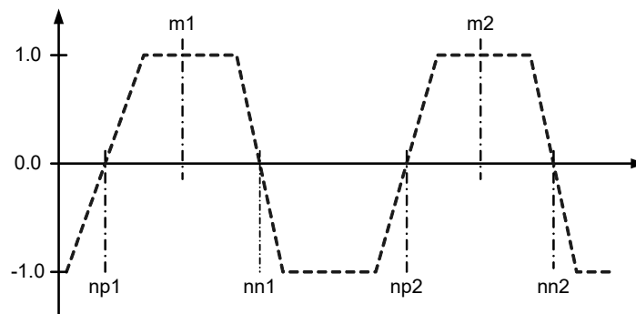
Abb. 11-18 Mittenpositionsberechnung (bei nicht ganz symmetrischem Zahnverlauf und positiver Logik)
