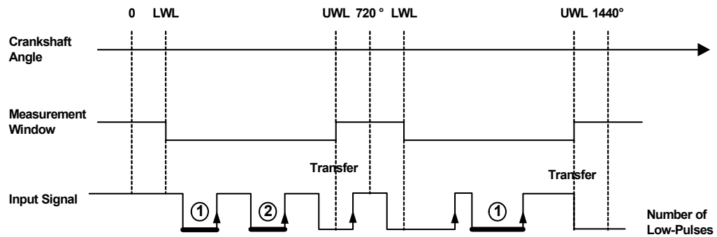
Abb. 12-27 Darstellung der Funktionsweise winkelsynchroner Messverfahren zur Pulszählung (Messverfahren Angular: Number of Low-Pulses). Pulse, die gezählt werden, sind durch erhöhte Linienstärke hervorgehoben.
