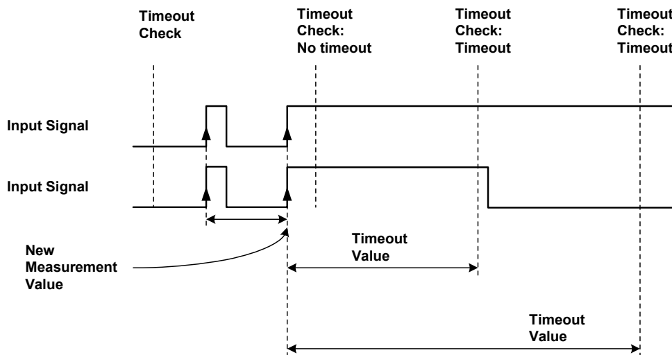
Abb. 9-20 Frequenz- und Zykluszeitmessungen an ansteigenden Flanken: Darstellung der Messwertberechnung im Timeout-Fall (der Messwert ist in der Darstellung als „Timeout Value“ bezeichnet) bei den „... InpDep“-Verfahren zur Timeout-Überwachung
