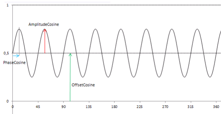
Abb. 23-41 Sine-Encoder: Kosinuskanal
