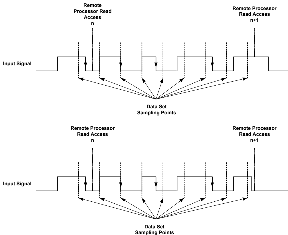
Abb. 17-46 Zählung fallender Flanken: Die Zahl der markierten fallenden Flanken wird beim (n+1)-ten Lesezugriff als Messwert zurückgegeben
