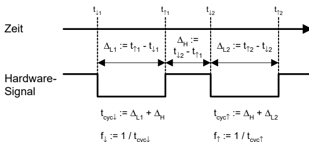
Abb. 33-27 Frequenzmessungen mit TMIO-Karte.
