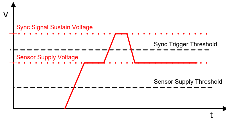
Abb. 22-13 Typischer Signalverlauf mit Schwellenspannungen
