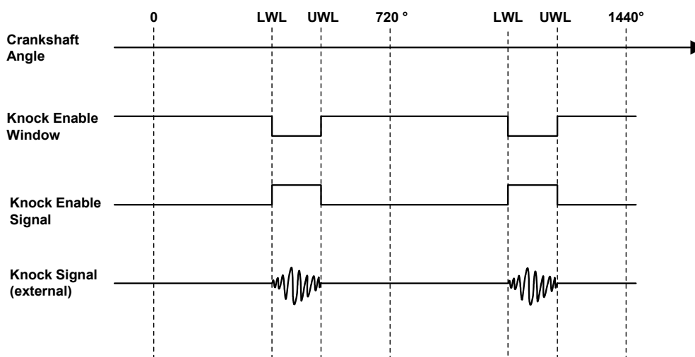
Abb. 9-4 High-aktives Klopf-Enable-Signal zur Aktivierung und Deaktivierung eines externen Klopfgenerators.
