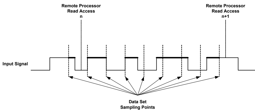
Abb. 17-43 Additive High-Zeit-Messung: Illustration der Messwertberechnung
