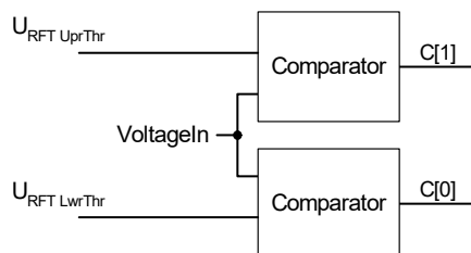
Abb. 12-3 Komparatorstufe für die Messung der Signalanstiegs- und -abfallzeiten
