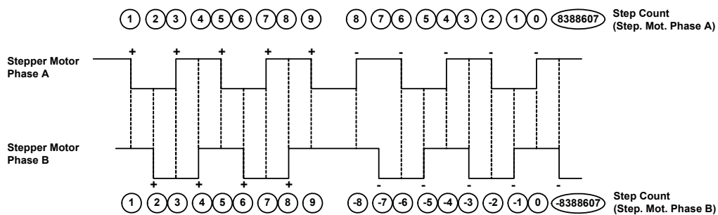
Abb. 5-13 Darstellung der Arbeitsweise der Positionsverfolgung an zwei-phasigen Schrittmotoren
