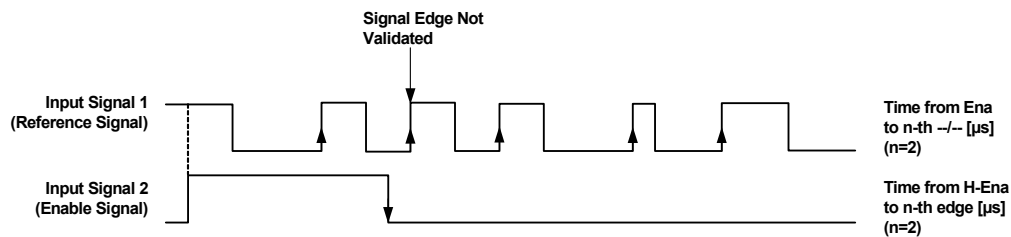
Abb. 10-25 Vermessung von Flanken auf unterschiedlichen Hardwarekanälen: Signalverlauf mit high-aktivem Enable-Signal und nicht validierter n-ter aktiver Signalfanke des Referenz-Signals
