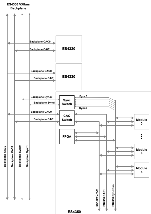
Abb. 18-60 ES4350 Winkelтакт-Bus und Synchronisationsbus
