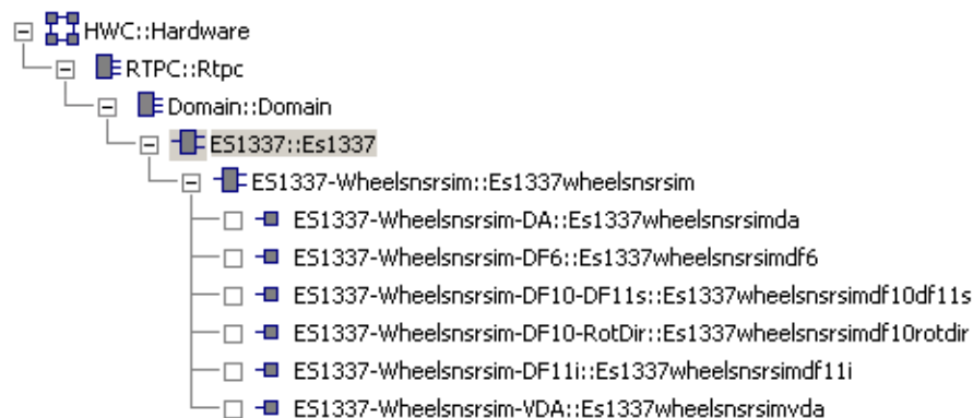
Abb. 13-1 RTIO-Hardwarebeschreibung mit eingebundener ES1337.1
