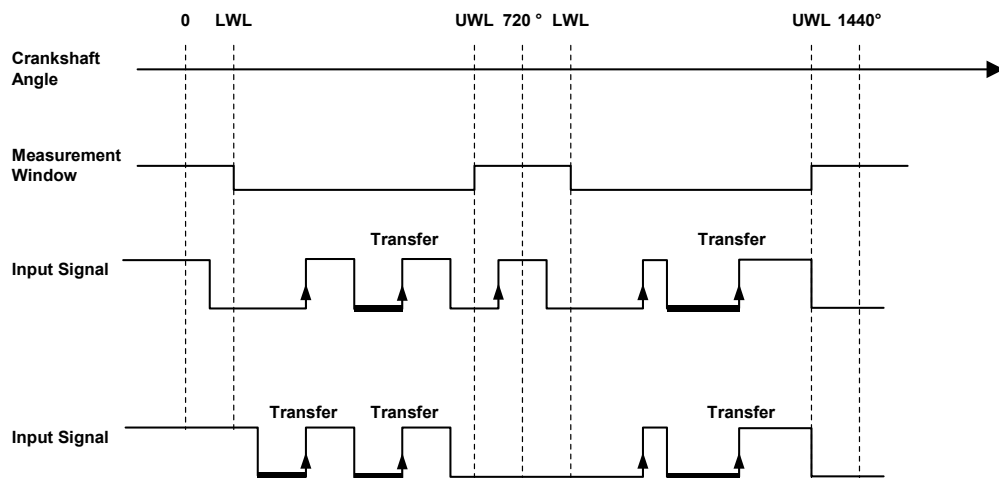
Abb. 9-15 Darstellung der Funktionsweise einer puls-qualifizierten, low-aktiven Pulsweitenmessung (Messverfahren „Lowtime (Pulse Qual.) [µs]“). Vermessene Pulse sind mit erhöhter Linienstärke hervorgehoben.
