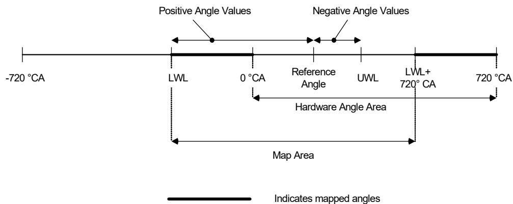
Abb. 12-25 Funktionsweise einer Winkelmessung.
