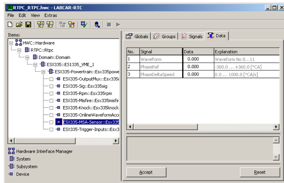
Abb. 11-20 Die Registerkarte „Data“ des ESX335-MSA-Sensor Device
