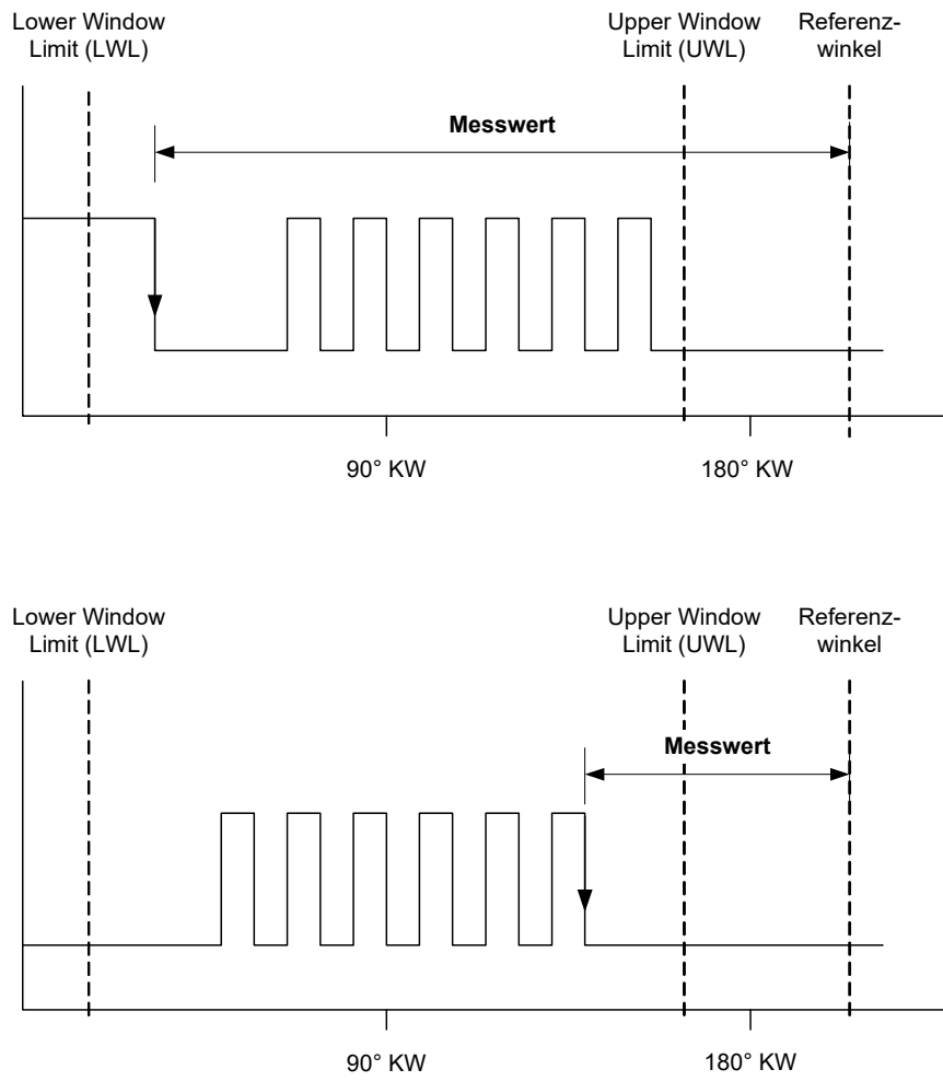
Abb. 5-21 Messwerte bei „Angle of First Falling Edge of Pulse Sequence“ (oben) und „Angle of Last Falling Edge of Pulse Sequence“ (unten)
