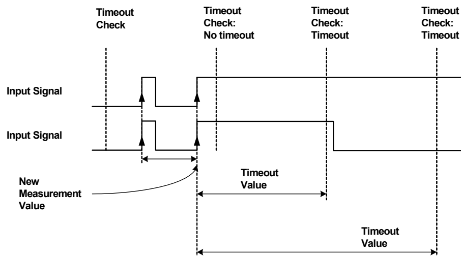
Abb. 10-23 Frequenz- und Zykluszeitmessungen an ansteigenden Flanken: Darstellung der Messwertberechnung im Timeout-Fall (der Messwert ist als „Timeout Value“ bezeichnet) bei den „... InpDep“-Verfahren zur Timeout-Überwachung.
