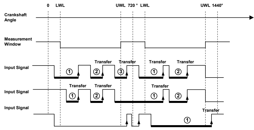
Abb. 18-43 Darstellung der Funktionsweise einer flanken-qualifizierten low-aktiven Pulsweitenmessung (Messverfahren „Lowtime (Edge Qual.) [µs]“). Vermessene Pulse sind mit erhöhter Linienstärke hervorgehoben. Die Zuordnung der Pulse zu den Winkelfenstern und die Zählung der Pulse innerhalb eines Winkelfensters ist ebenfalls dargestellt.
