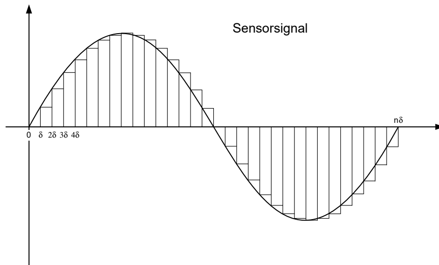
Abb. 7-4 Erzeugung einer variablen Sinusfrequenz (siehe Text)
