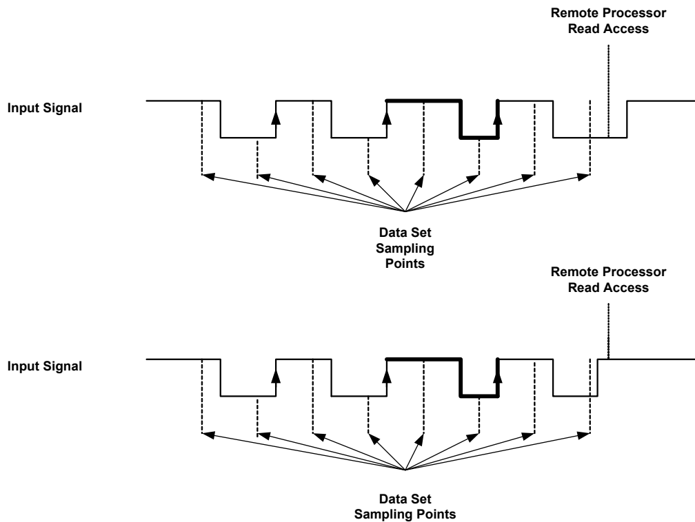
Abb. 21-14 Ausgewertete Periode (fett gezeichnet) bei einer Frequenz- oder Zykluszeitmessung an ansteigenden Flanken
