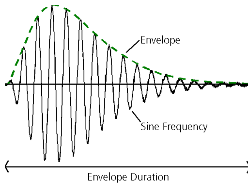
Abb. 18-20 Klopfsignal (durchgezogen) und Einhüllende (gestrichelt)
