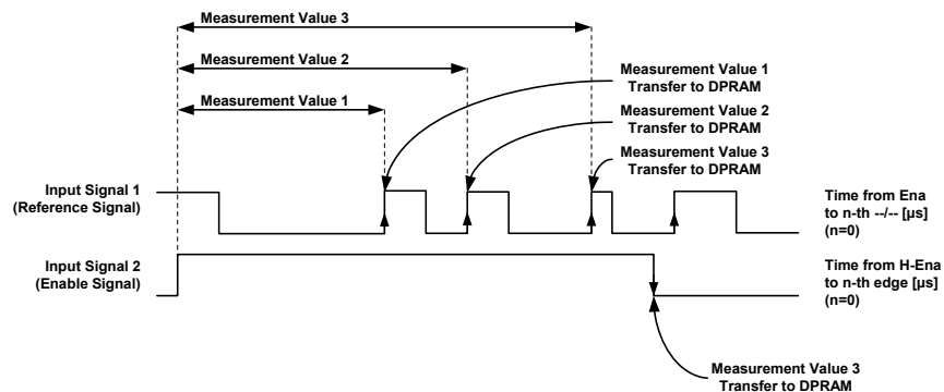
Abb. 18-53 Funktionsweise der Messverfahren zur Vermessung von Ereignissen (Flanken) auf unterschiedlichen Signalen bzw. Hardwarekanälen relativ zueinander. Dargestellt ist eine Messung mit high-aktivem Enable-Signal. Der RTIO-Parameter zur Flanken-Selektion („(Max) Pulse (Count)“ in der Registerkarte „Signals“) ist gleich 0.
