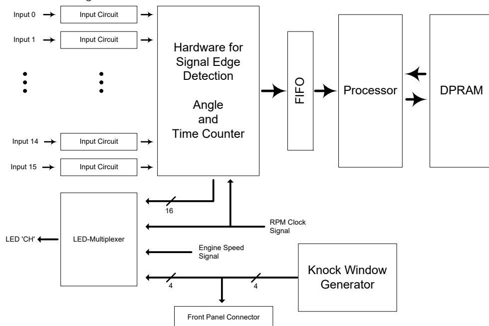
Abb. 9-1 Blockschaltbild des ES1334.1 Measurement Board
