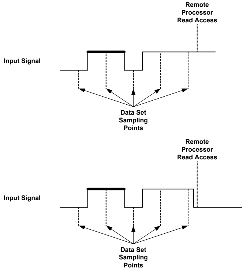
Abb. 5-8 High-Zeit-Messung (der gemessene Puls ist mit fetter Strichstärke hervorgehoben)
