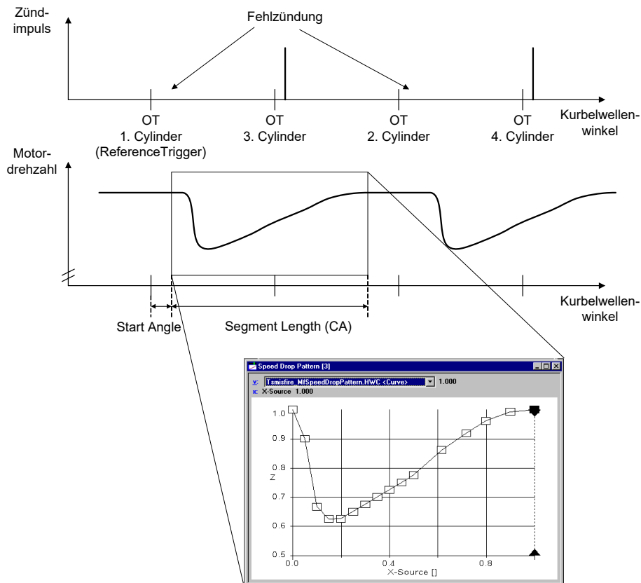
Abb. 33-19 Fehlzündung und Abfall der Motordrehzahl
