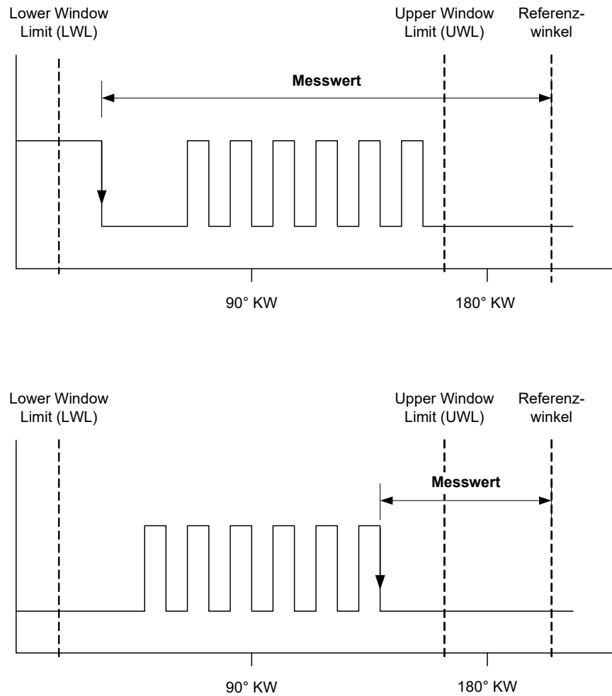
Abb. 24-36 Messwerte bei „Angle of First Falling Edge of Pulse Sequence“ (oben) und „Angle of Last Falling Edge of Pulse Sequence“ (unten)
