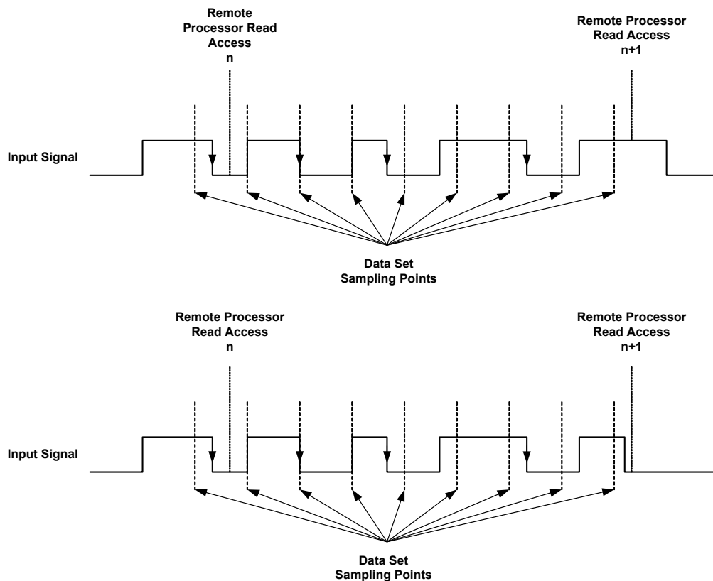
Abb. 5-11 Zählung fallender Flanken: Die Zahl der markierten fallenden Flanken wird beim (n+1)-ten Lesezugriff als Messwert zurückgegeben
