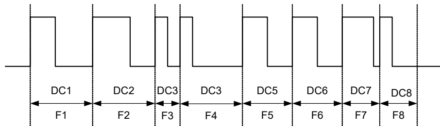
Abb. 5-26 Eine Abfolge von acht Pulsen ( F_x = Frequenz von Puls x , DC_x = Tasterhältnis von Puls x )
