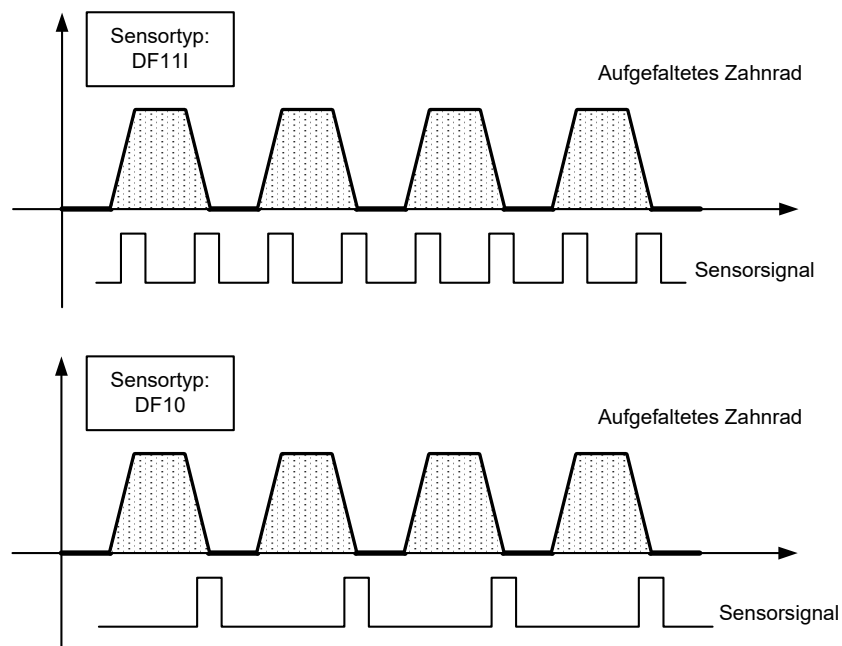
Abb. 7-5 Sensorsignal eines DF11I und eines DF10 Drehzahlfühlers
