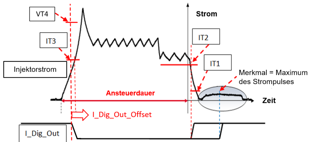
Abb. 26-5 Typischer CRI2-x Injektorstromverlauf mit Merkmal (graue Ellipse) und „I_Dig_Out“ Signal
