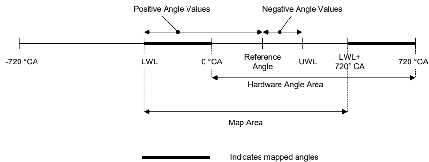
Abb. 18-54 Funktionsweise einer Winkelmessung im drehzahlsynchronen Messmodus
