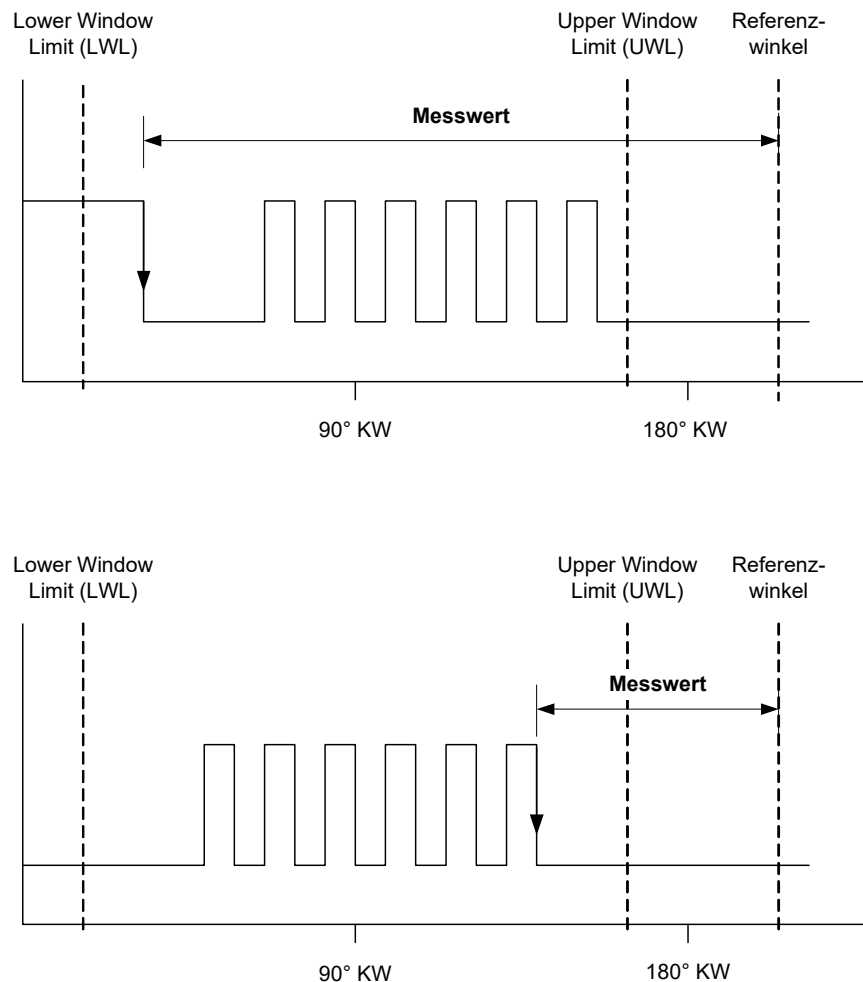
Abb. 21-22 Messwerte bei „Angle of First Falling Edge of Pulse Sequence“ (oben) und „Angle of Last Falling Edge of Pulse Sequence“ (unten)
