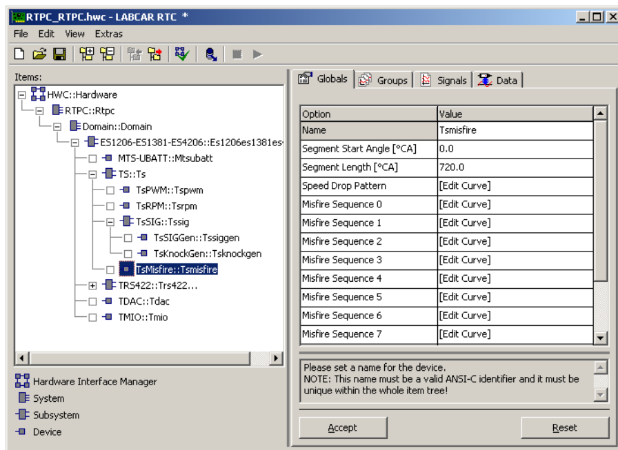
Abb. 33-20 Die Registerkarte „Globals“ des TsMisfire Devices
