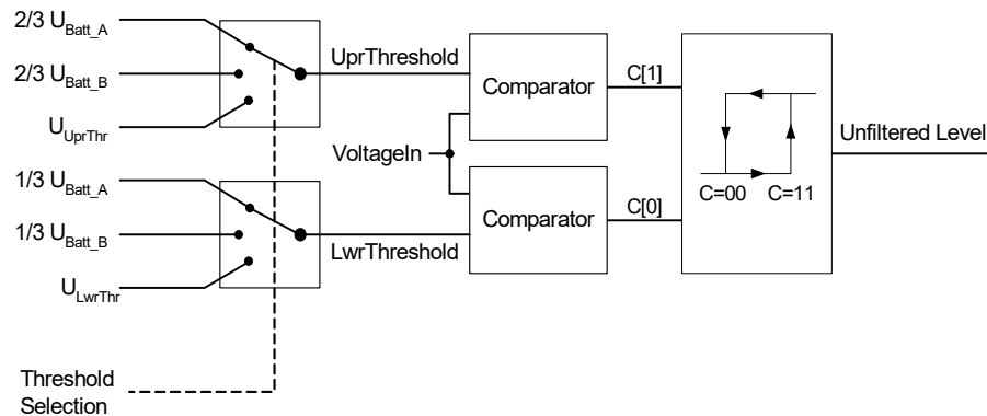
Abb. 12-2 Komparatorstufe
