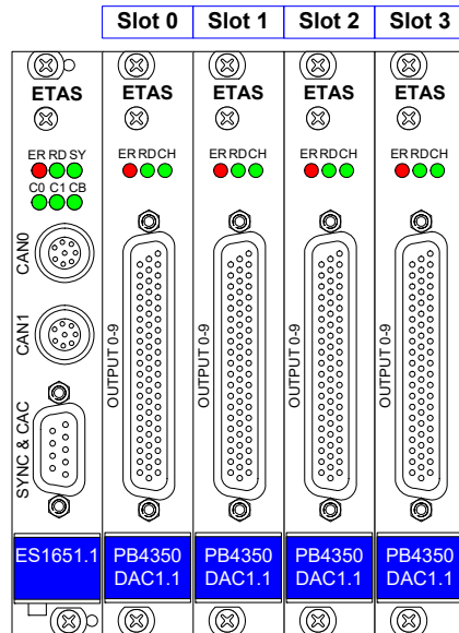
Abb. 18-67 Nummerierung der Modul-Steckplätze einer ES1651-Trägerkarte
