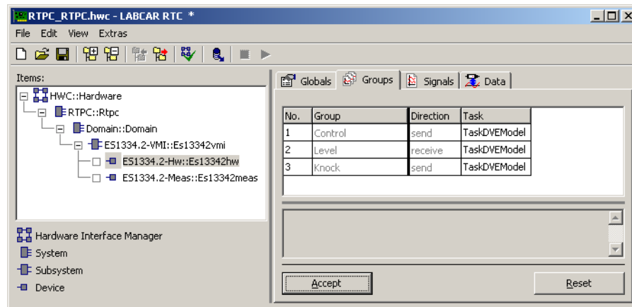
Abb. 10-10 Die Registerkarte „Groups“ des ES1334.2-Hw-Device
