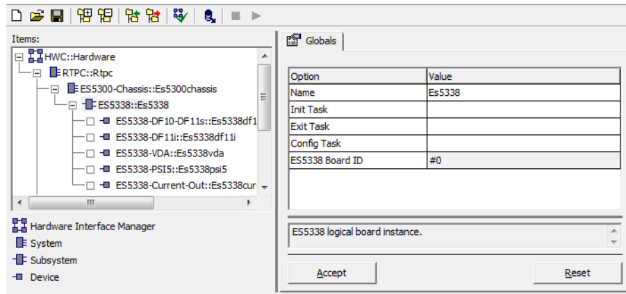
Abb. 22-2 Die Registerkarte „Globals“ des ES5338 Subsystems
