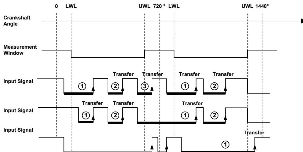
Abb. 9-16 Darstellung der Funktionsweise einer flanken-qualifizierten, low-aktiven Pulsweitenmessung (Messverfahren „Lowtime (Edge Qual.) [µs]“). Vermessene Pulse sind mit erhöhter Linienstärke hervorgehoben. Die Zuordnung der Pulse zu den Winkelfenstern und die Zählung der Pulse innerhalb eines Winkelfensters ist ebenfalls dargestellt.
