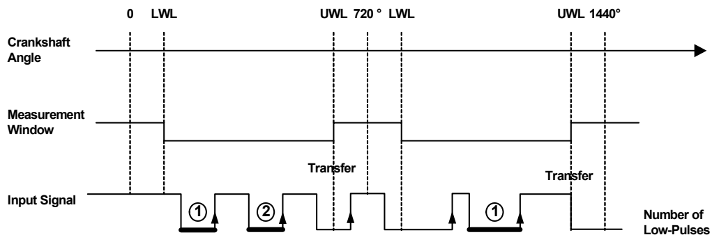
Abb. 24-33 Darstellung der Funktionsweise winkelsynchroner Messverfahren zur Pulszählung (Messverfahren Angular: Number of Low-Pulses). Pulse, die gezählt werden, sind durch erhöhte Linienstärke hervorgehoben.
