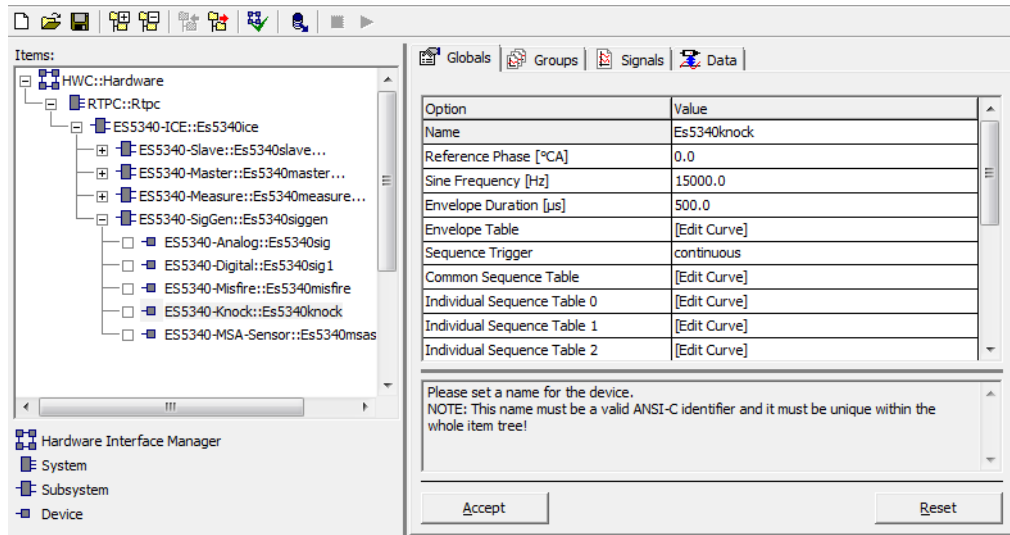
Abb. 24-45 Die Registerkarte „Globals“ des ES5340-Knock Device
