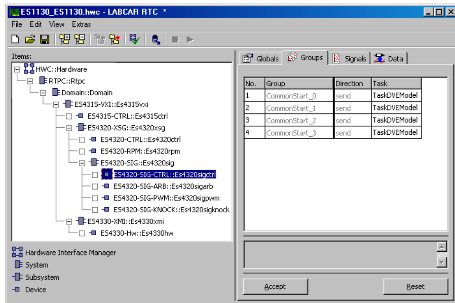
Abb. 18-12 Die Registerkarte „Groups“ des ES4320-SIG-CTRL Devices
