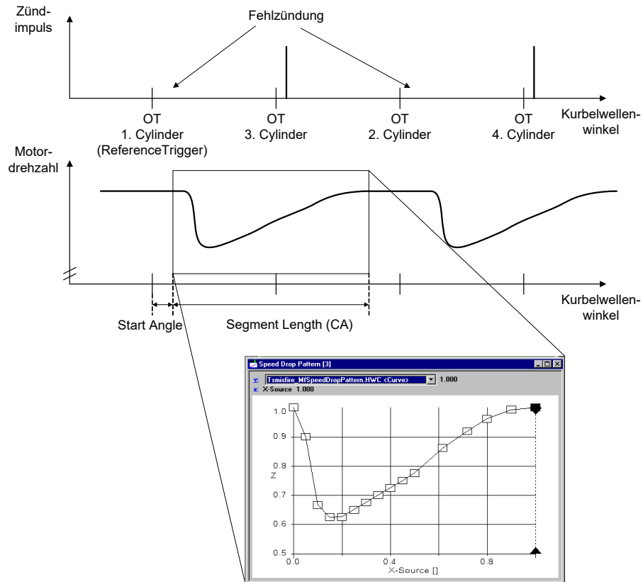
Abb. 18-27 Fehlzündung und Abfall der Motordrehzahl
