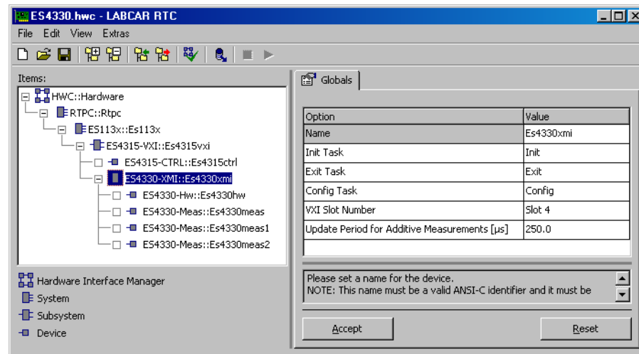
Abb. 18-34 RTIO Hardwarebeschreibung mit ES4315 VMEbus/VXIbus-Adapter und ES4330-Karte
