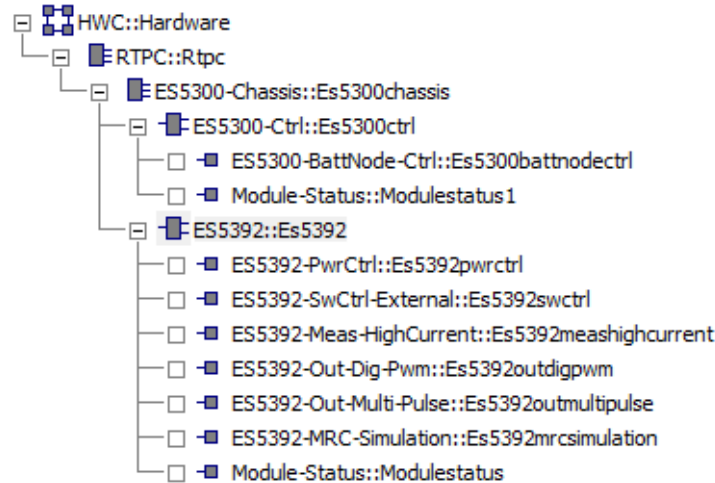
Abb. 28-1 RTIO-Hardwarebeschreibung mit ES5392.1 High Current Switch Board
