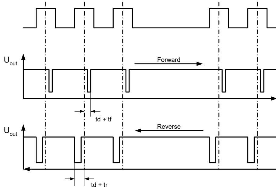
Abb. 11-17 Kurbelwellenzähne und Sensorsignale bei einem MSA-Sensor
