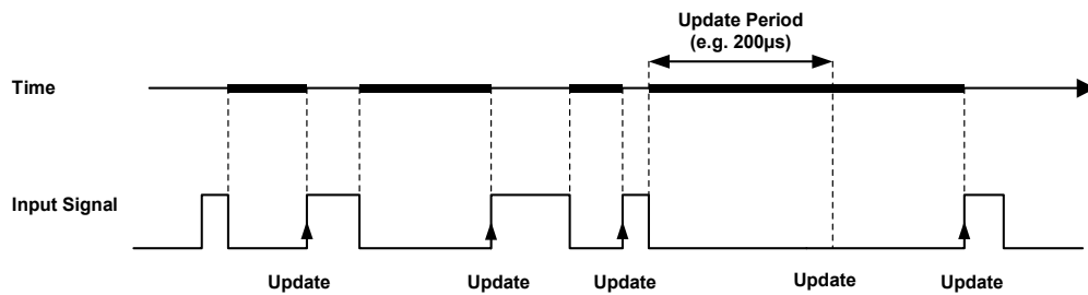
Abb. 9-18 Darstellung der Funktionsweise einer asynchronen additiven Lowzeit-Messung (Messverfahren „Additive Lowtime [µs]“). Die additive Zeit setzt sich aus den fett markierten Zeitsegmenten zusammen. Die Zeitpunkte, an denen die Summe im DPRAM aktualisiert wird, sind ebenfalls dargestellt.
