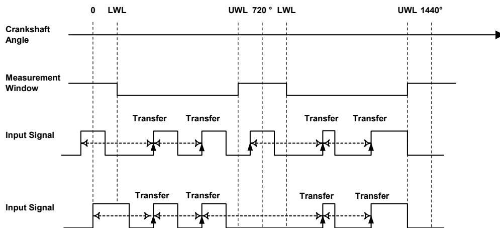
Abb. 9-19 Darstellung der Messwertberechnung bei einer winkelsegmentierten Frequenz- oder Zykluszeitmessung an steigenden Signalflanken
