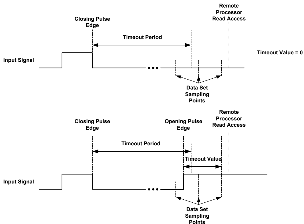
Abb. 17-42 Pulsweitenmessungen: Messwert im Timeout-Fall im „Intvl InpDep“-Modus am Beispiel einer High-Zeit-Messung
