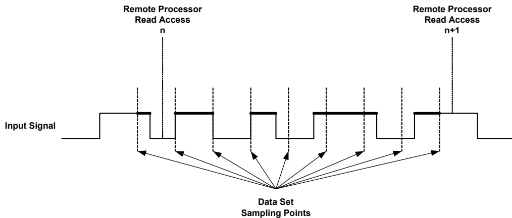
Abb. 21-13 Additive High-Zeit-Messung: Illustration der Messwertberechnung
