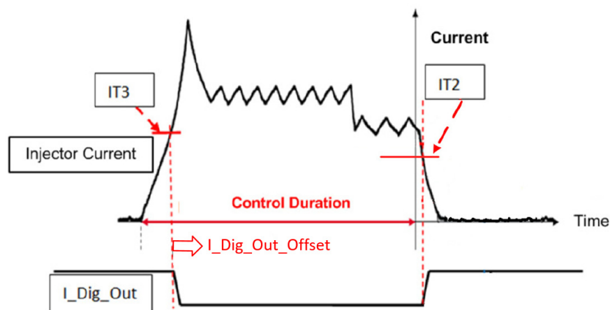
Abb. 31-3 Typischer Injektor-Stromverlauf für passive Injektorsimulation und I_Dig_Out-Signal.
