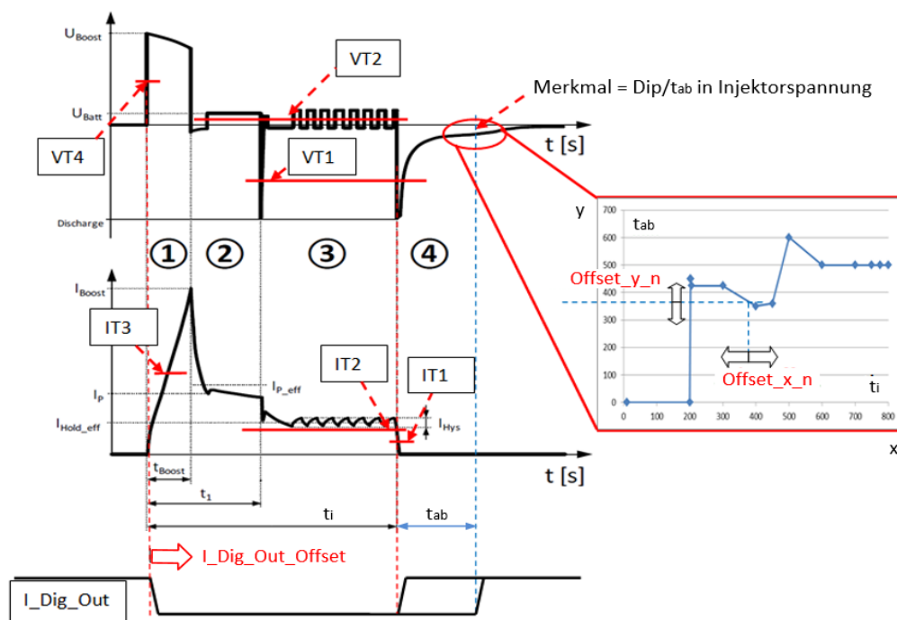
Abb. 19-19 Typischer HDEV5 CVO-Injektorstrom-/Injektorspannungsverlauf mit Merkmal und „I_Dig_Out“ Signal
