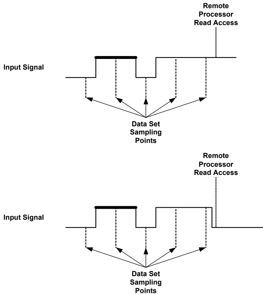
Abb. 21-12 High-Zeit-Messung (der gemessene Puls ist mit fetter Strichstärke hervorgehoben)
