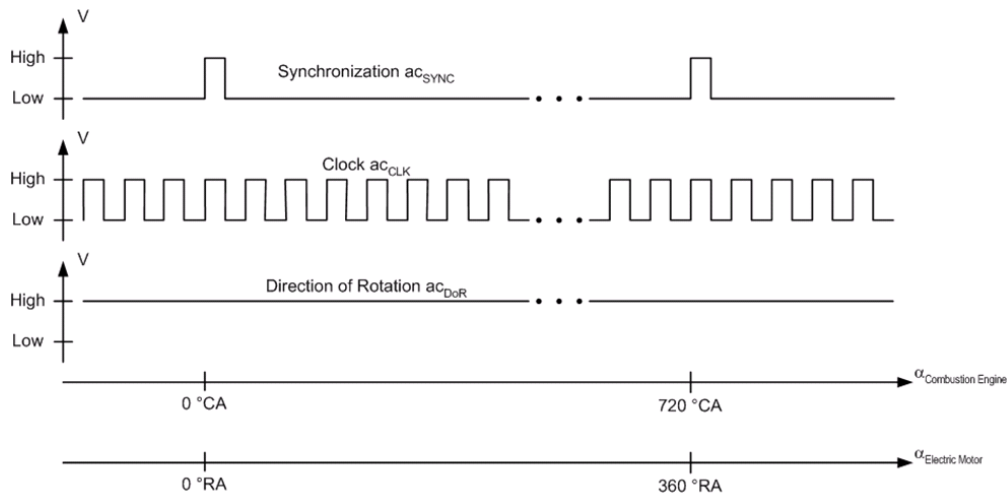
Abb. 23-3 Die drei Komponenten des Winkeltaktsignals
