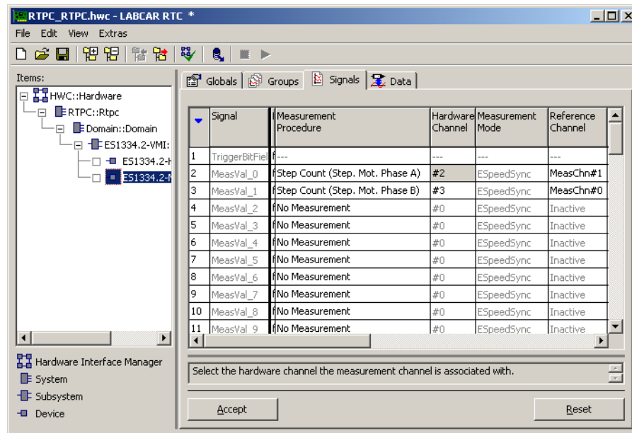
Abb. 10-29 Konfiguration einer Messung zur Positionsverfolgung an zwei-phasigen Schrittmotoren
