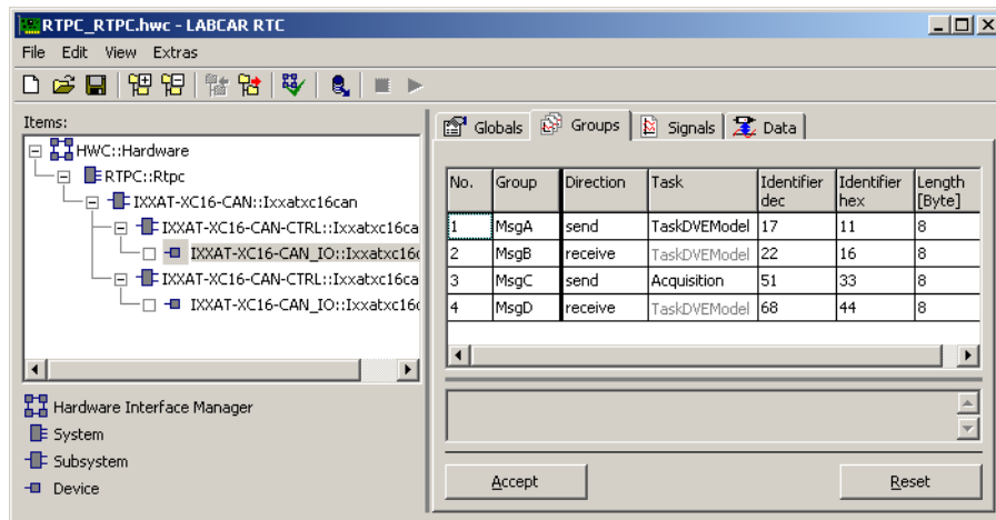
Abb. 32-10 Die Registerkarte „Groups“ des IXXAT-XC16-CAN_IO Devices
