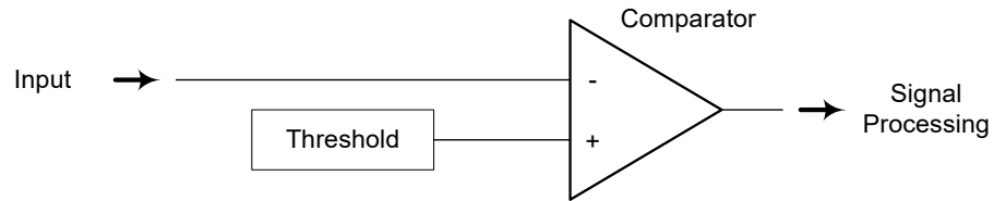
Abb. 10-2 Vereinfachte Darstellung der Eingangsbeschaltung eines Hardwarekanals
