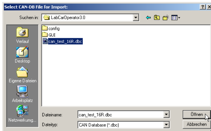
Abb. 17-12 CANdb Auswahl
