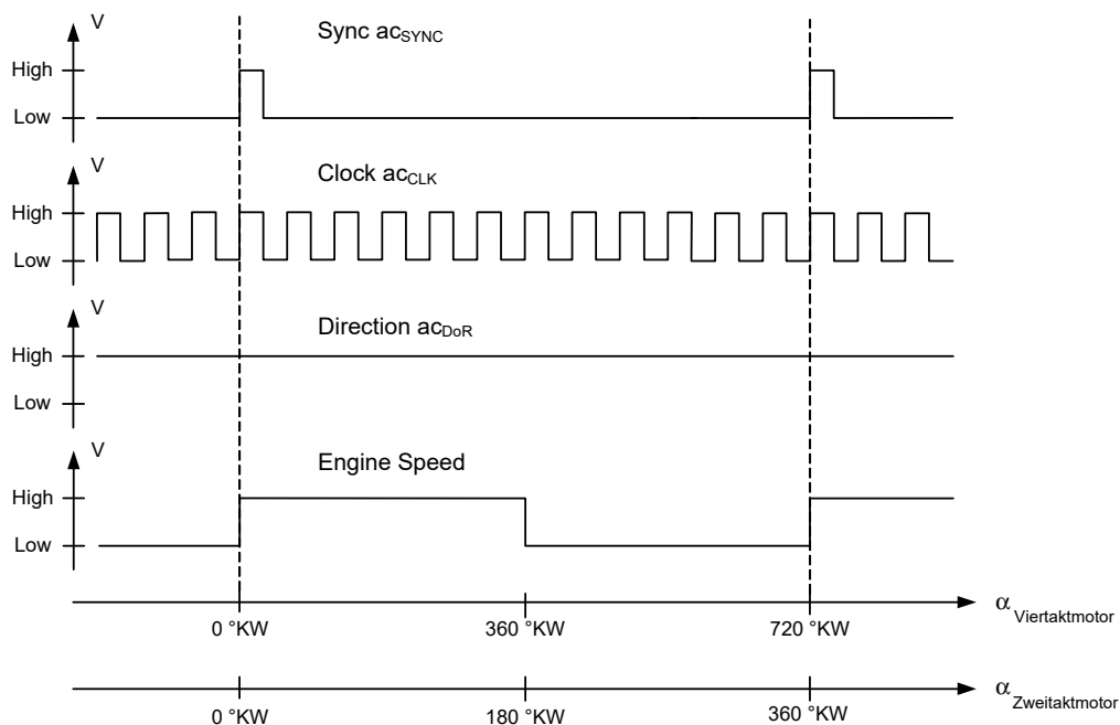
Abb. 24-3 Die drei Komponenten des Winkeltaktsignals
