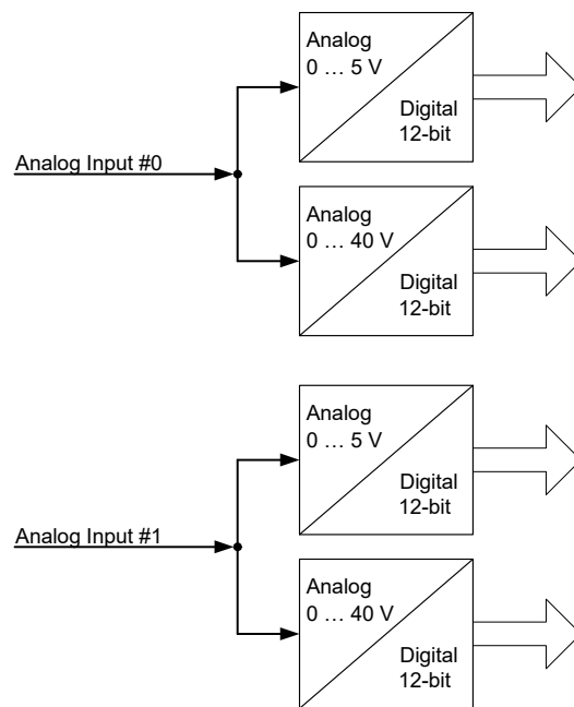
Abb. 23-12 Schematische Darstellung der Analog-Einheit.
