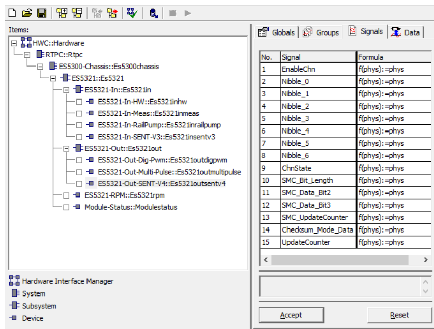
Abb. 21-31 Die Registerkarte „Signals“ des ES5321-Out-SENT Devices
