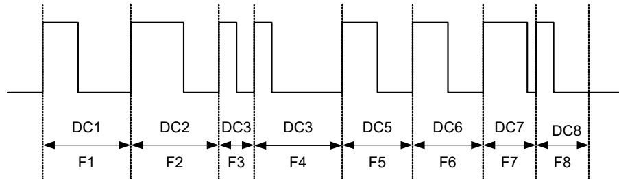
Abb. 21-27 Eine Abfolge von acht Pulsen (Fx = Frequenz von Puls x, DCx = Tastverhältnis von Puls x)
