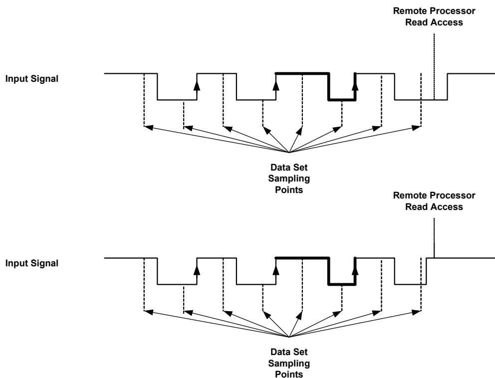
Abb. 17-47 Ausgewertete Periode (fett gezeichnet) bei einer Frequenz- oder Zykluszeitmessung an ansteigenden Flanken
