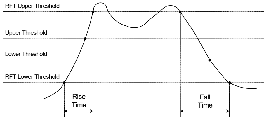
Abb. 12-5 Vermessung von Anstiegs- und Abfallzeiten
