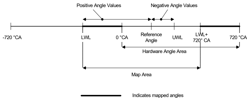
Abb. 24-32 Funktionsweise einer Winkelmessung.
