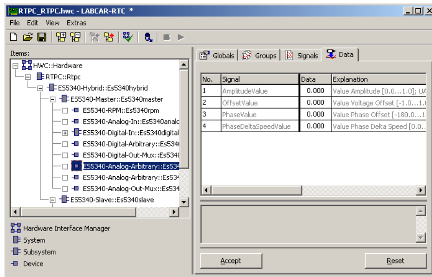
Abb. 23-49 Die Registerkarte „Data“ des ES5340-Analog-Arbitrary RTIO-Elements
