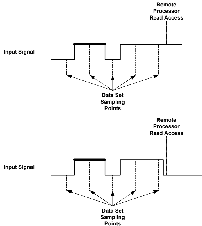
Abb. 17-41 High-Zeit-Messung (der gemessene Puls ist mit fetter Strichstärke hervorgehoben)
