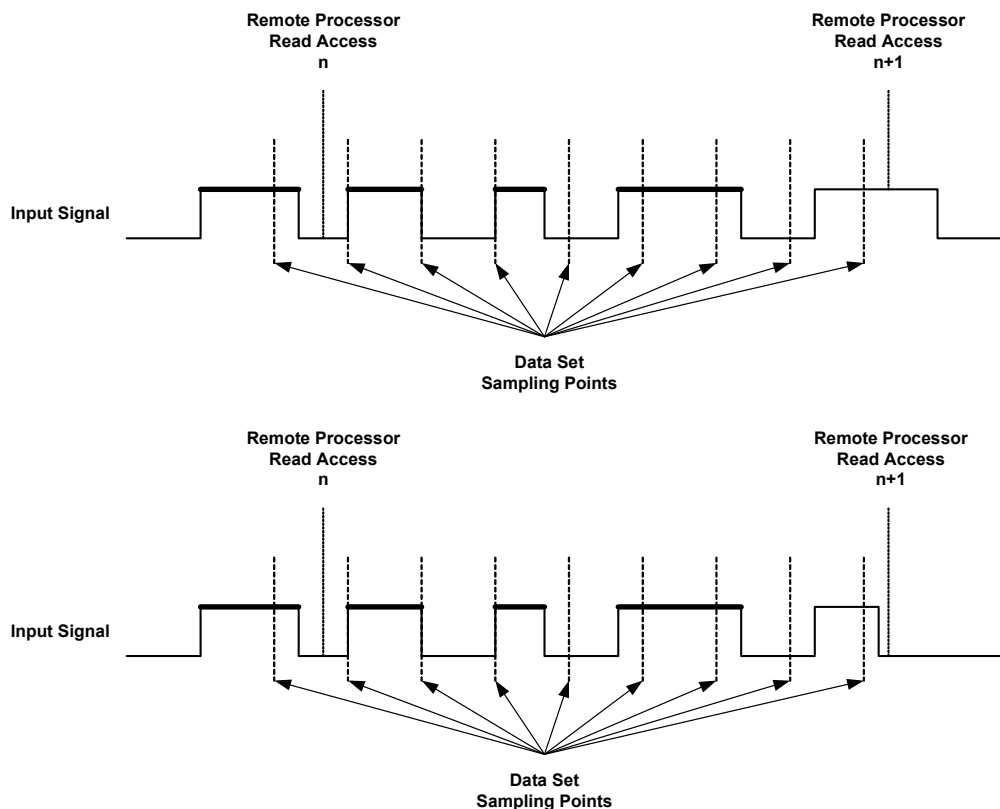
Abb. 17-45 High-Puls-Zählung: Die Anzahl der mit fetter Strichstärke markierten Pulse wird beim (n+1)-ten Lesevorgang als Messwert zurückgegeben
