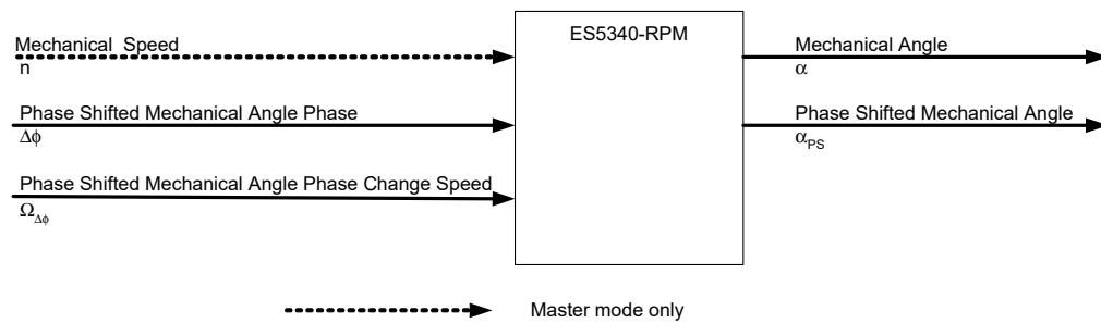
Abb. 23-5 Steuer- und Statussignale der Drehzahleinheit bei der Simulation von Elektromotoren im einfachen Master-Betrieb
