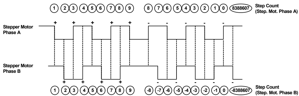
Abb. 10-30 Darstellung der Arbeitsweise der Positionsverfolgung an zwei-phasigen Schrittmotoren
