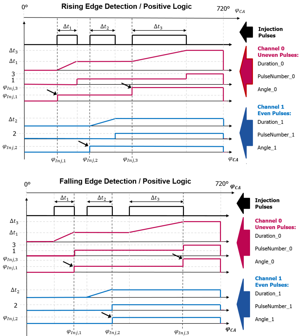
Abb. 24-22 Erfassung der steigenden Flanke und Erfassung der fallenden Flanke für positive Logik
