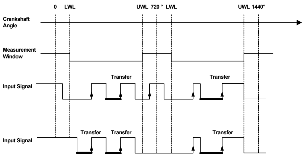
Abb. 10-15 Darstellung der Funktionsweise einer puls-qualifizierten, low-aktiven Pulsweitenmessung (Messverfahren „Lowtime (Pulse Qual.) [µs]“). Vermessene Pulse sind mit erhöhter Linienstärke hervorgehoben.
