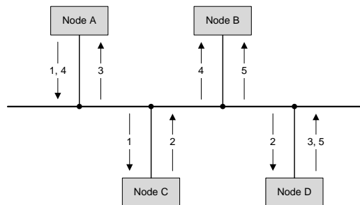
Abb. 3-9 CAN-Netzwerk mit vier Knoten und fünf Messages
