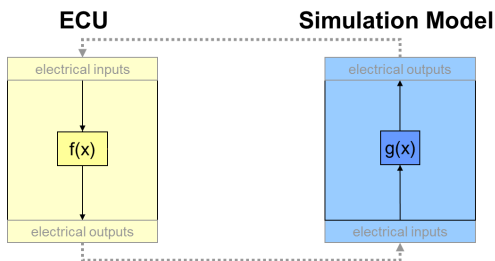
Abb. 3-33 Aufbau eines HiL-Systems
