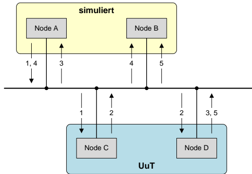
Abb. 3-10 Physikalisch vorhandene (UuT) und simulierte Knoten
