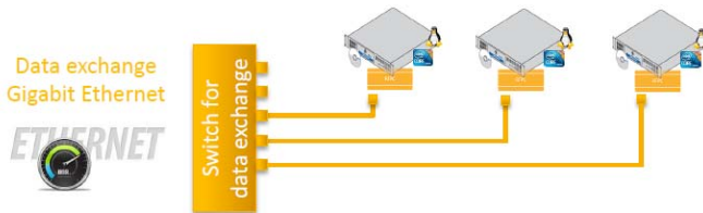
Abb. 3-57 Datenaustausch zwischen den Real-Time PCs
