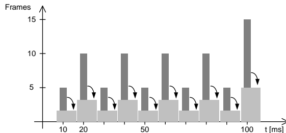
Abb. 3-14 Wirkungsweise der Option „Spread Send Frames“ (siehe Text)
