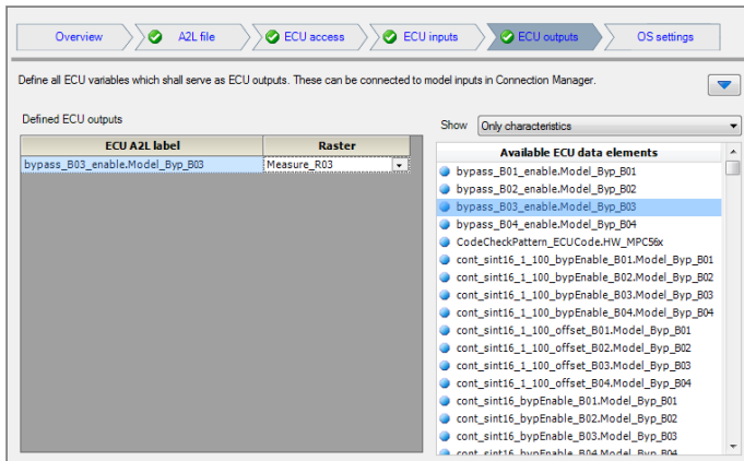
Abb. 3-37 Steuergeräteausgänge zur Verbindung mit Modelleingängen bereitstellen
