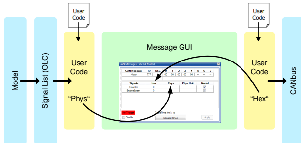
Abb. 3-15 Signalfluss bei Send-Message (siehe Text)
