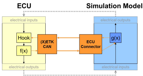
Abb. 3-34 FiL-System
