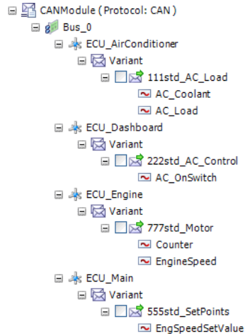
Abb. 3-13 Das CAN-Netzwerk
