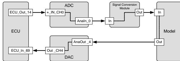
Abb. 3-45 Signale, Pins und virtuelle Verbindungen (gestrichelt)
