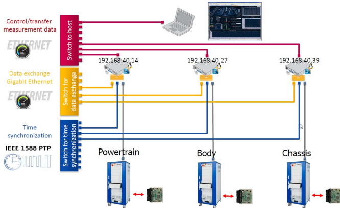
Abb. 3-55 Architektur eines Multi-RTPC-Systems
