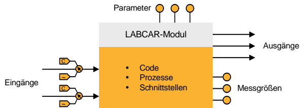
Abb. 3-1 Ein LABCAR-Modul
