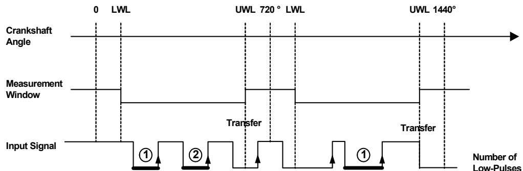
Abb. 23-33 Darstellung der Funktionsweise winkelsynchroner Messverfahren zur Pulszählung (Messverfahren Angular: Number of Low-Pulses). Pulse, die gezählt werden, sind durch erhöhte Linienstärke hervorgehoben.
