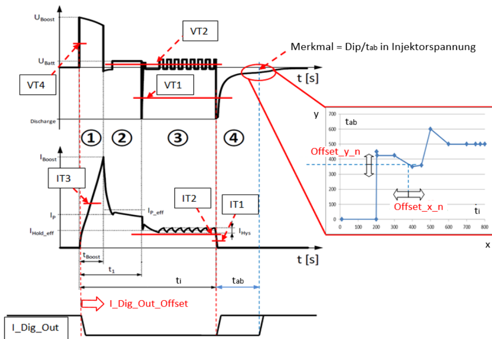
Abb. 25-4 Typischer HDEV5 CVO-Injektorstrom-/Injektorspannungsverlauf mit Merkmal und „I_Dig_Out“ Signal
