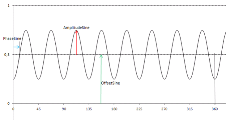
Abb. 22-40 Sine-Encoder: Sinuskanal
