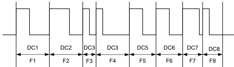
Abb. 20-27 Eine Abfolge von acht Pulsen ( F_x = Frequenz von Puls x , DC_x = Tastverhältnis von Puls x )
