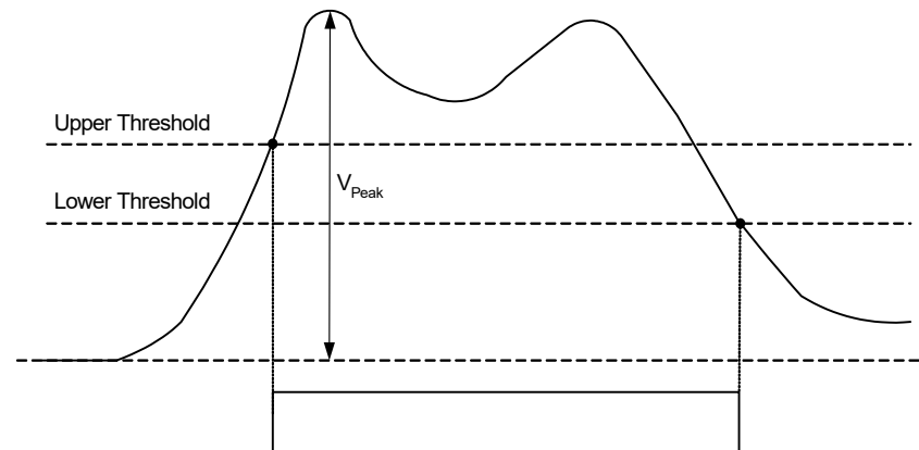
Abb. 11-6 Spitzenwertvermessung
