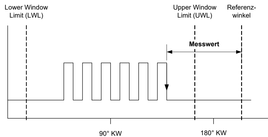
Abb. 23-36 Messwerte bei „Angle of First Falling Edge of Pulse Sequence“ (oben) und „Angle of Last Falling Edge of Pulse Sequence“ (unten)
