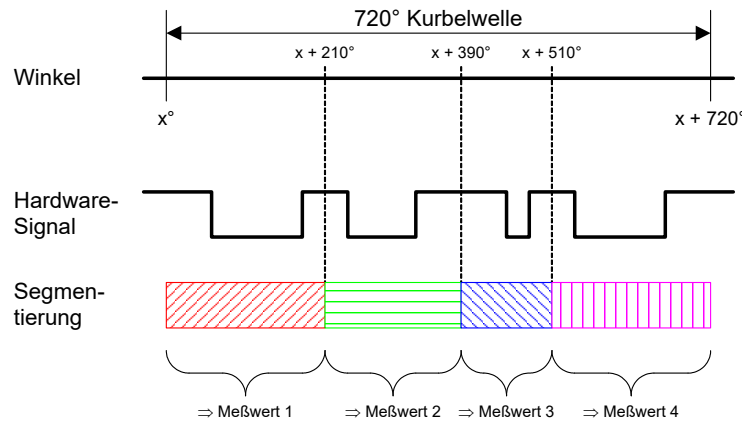
Abb. 32-30 Winkelsegmentierung mit TMIO-Karte
