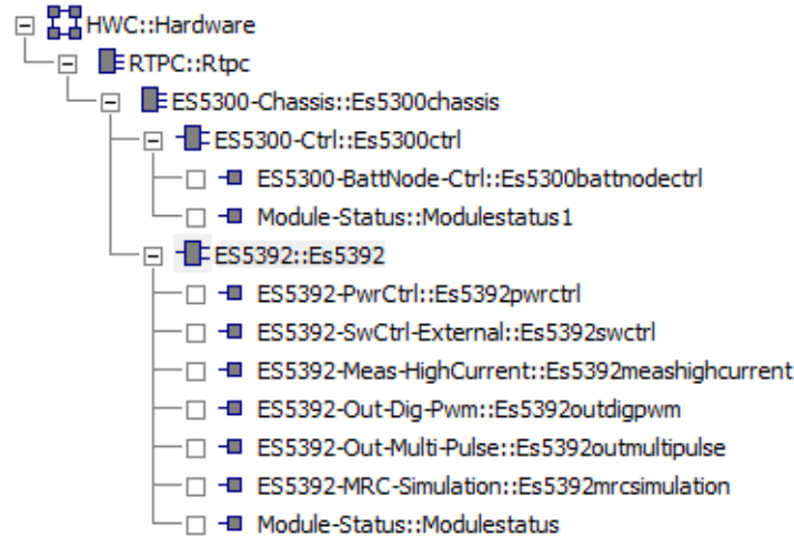
Abb. 27-1 RTIO-Hardwarebeschreibung mit ES5392.1 High Current Switch Board
