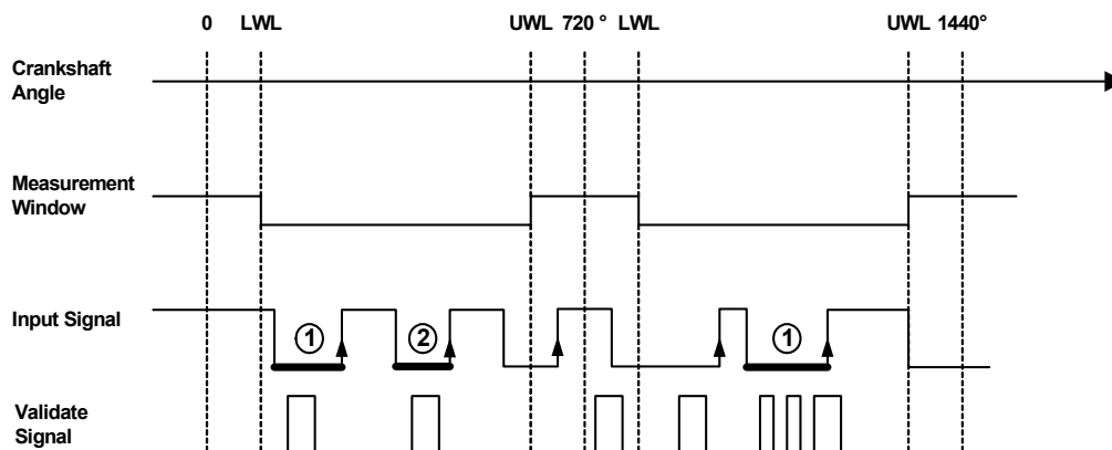
Abb. 11-23 Darstellung der Funktionsweise einer winkelsynchronen Pulsweitenmessung mit Validierungssignal (Messverfahren „Angular: L-Time n-th Pulse (H-Valid.) [ \mu\text{s} ]“). Validierte Pulse sind mit erhöhter Linienstärke hervorgehoben.
