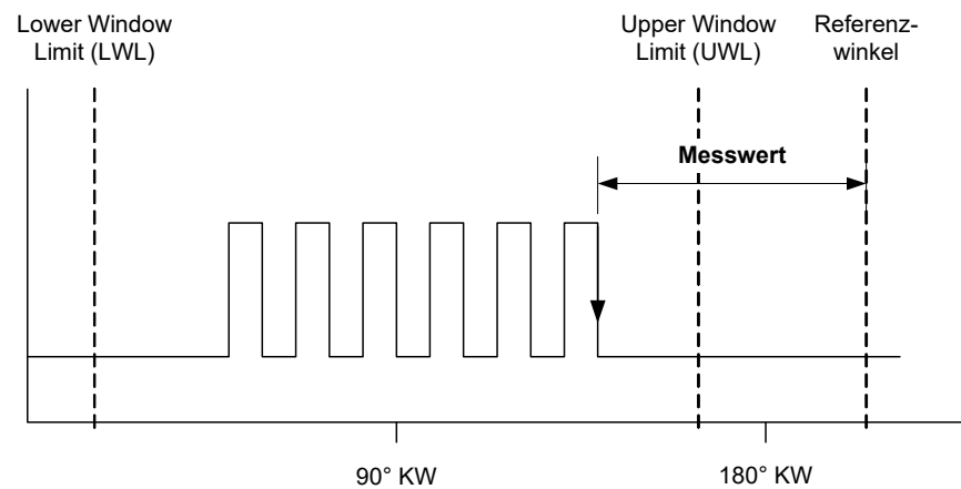
Abb. 20-22 Messwerte bei „Angle of First Falling Edge of Pulse Sequence“ (oben) und „Angle of Last Falling Edge of Pulse Sequence“ (unten)
