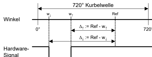
Abb. 32-23 Winkelmessungen mit der TMIO-Karte
