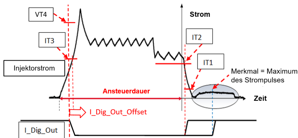
Abb. 30-2 Typischer CR12X Injektorstromverlauf mit Merkmal (graue Ellipse) und „I_Dig_Out“ Signal
