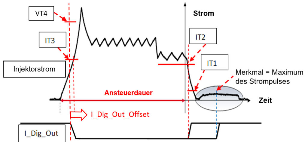
Abb. 18-20 Typischer CR12-x Injektorstromverlauf mit Merkmal (graue Ellipse) und „I_Dig_Out“ Signal
