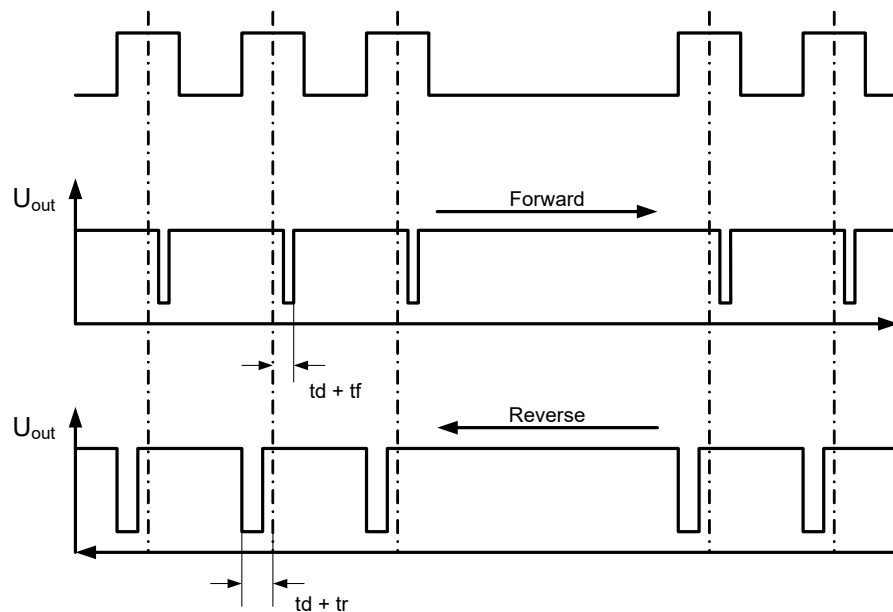
Abb. 23-48 Kurbelwellenzähne und Sensorsignale bei einem MSA-Sensor
