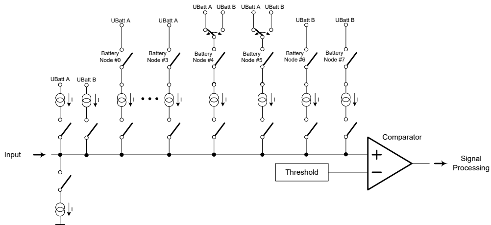
Abb. 17-32 Vereinfachte Darstellung der Eingangsbeschaltung eines ES4330 Hardwarekanals
