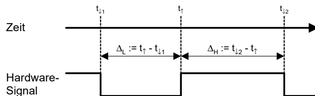
Abb. 32-24 Zeitmessungen mit TMIO-Karte
