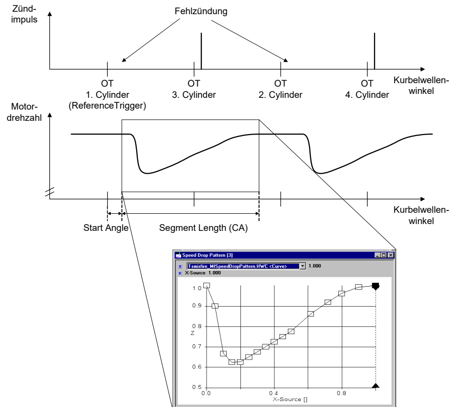
Abb. 32-19 Fehlzündung und Abfall der Motordrehzahl
