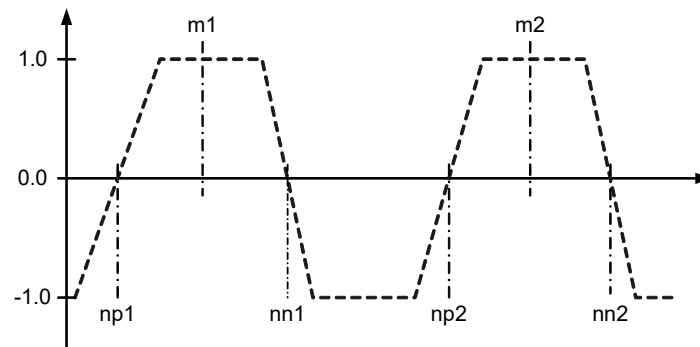
Abb. 23-49 Mittenpositionsberechnung (bei nicht ganz symmetrischem Zahnverlauf und positiver Logik)
