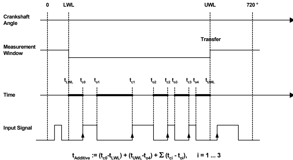
Abb. 23-31 Darstellung der Funktionsweise einer winkelsynchronen additiven Lowzeit-Messung (Messverfahren Angular: Additive Lowtime [µs]). Die additive Zeit setzt sich aus der Summe der fett markierten Liniensegmente zusammen.
