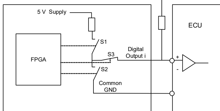
Abb. 22-34 Prinzipschaltbild für die beiden Einstellungen „Pull-Up to +5 V“ und „Open Collector“ in der Registerkarte „Signals“
