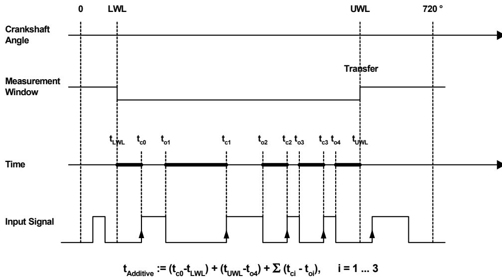
Abb. 11-24 Darstellung der Funktionsweise einer winkelsynchronen additiven Lowzeit-Messung (Messverfahren Angular: Additive Lowtime [µs]). Die additive Zeit setzt sich aus der Summe der fett markierten Liniensegmente zusammen.
