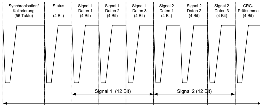
Abb. 4-14 Format eines Signals gemäß SENT-Datenprotokoll
