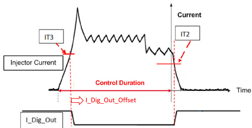
Abb. 30-3 Typischer Injektor-Stromverlauf für passive Injektorsimulation und I_Dig_Out-Signal.
