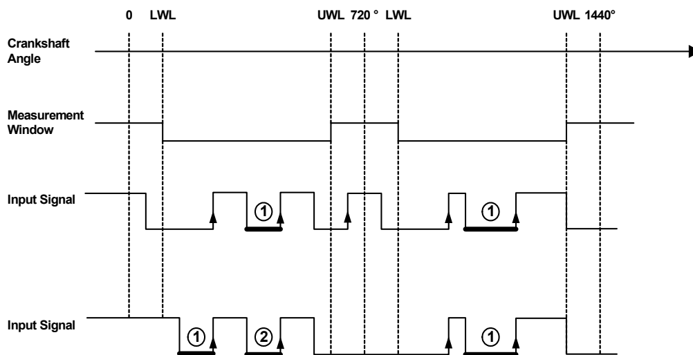
Abb. 23-29 Darstellung der Funktionsweise einer puls-qualifizierten, low-aktiven Pulsweitenmessung (Messverfahren Angular: L-Time n-th Pulse (Pu Qual.) [ \mu s]). Vermessene Pulse bzw. Pulse die gezählt werden sind mit erhöhter Linienstärke hervorgehoben.
