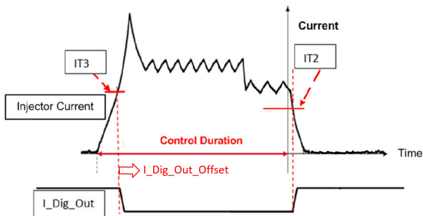
Abb. 25-6 Typischer Injektor-Stromverlauf für ES4455.2-Generic-Load-Carrier-(Legacy-Mode) und I_Dig_Out-Signal.
