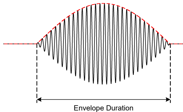
Abb. 23-38 Ein Klopfpaket
