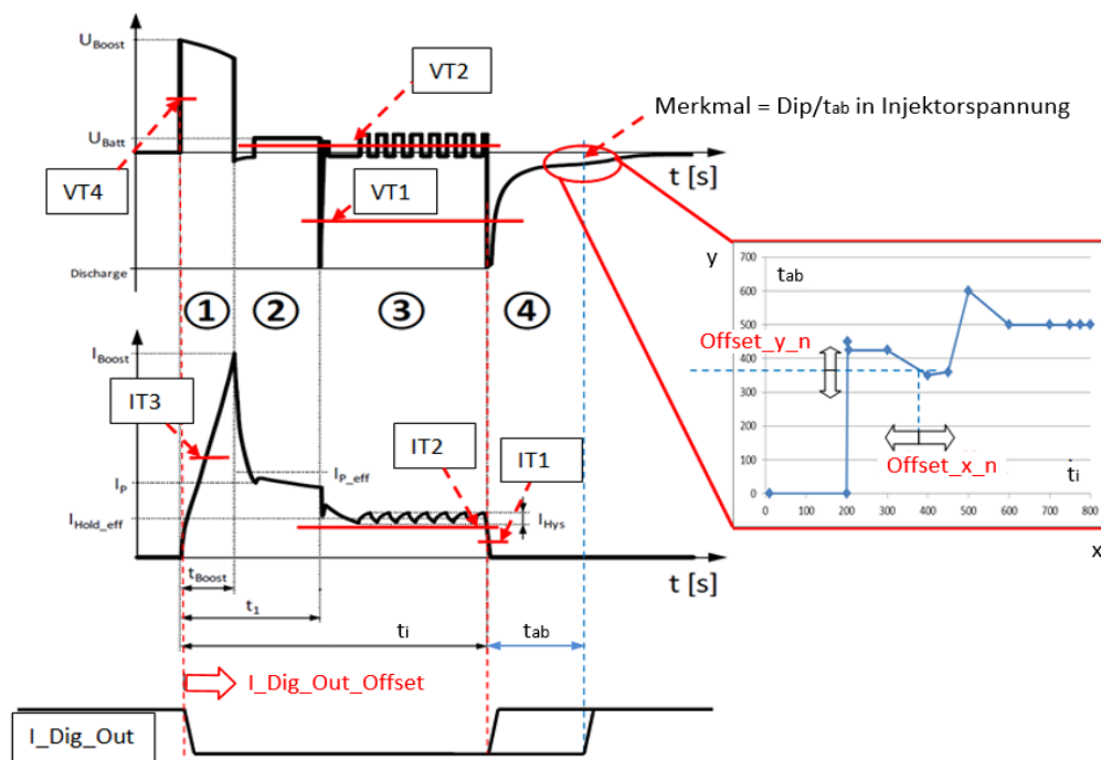
Abb. 30-1 Typischer HDEV5/HDEV6 CVO-Injektorstrom-/Injektorspannungsverlauf mit Merkmal und I_Dig_Out-Signal Rot umrandetes Insert: Interpolierter Graph aus Valve-Closing-Delay-Table t_{tab} : Schließ-Verzögerungszeit nach Ansteuerende = Verzögerungszeit nach Ansteuerende für das Auftreten des Merkmals t_i : Ansteuerdauer des Injektors
