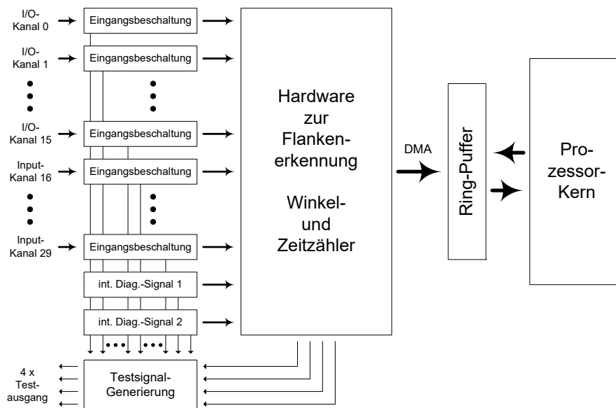
Abb. 32-22 Blockschaltbild TMIO-Karte
