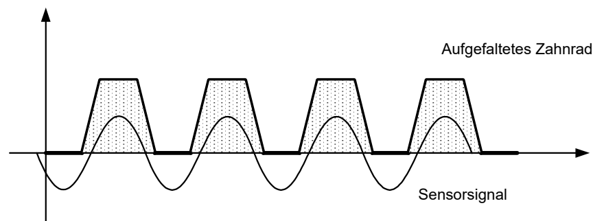
Abb. 6-2 Das Sensorsignal eines passiven Drehzahlfühlern
