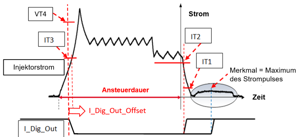
Abb. 25-5 Typischer CRI2-x Injektorstromverlauf mit Merkmal (graue Ellipse) und „I_Dig_Out“ Signal
