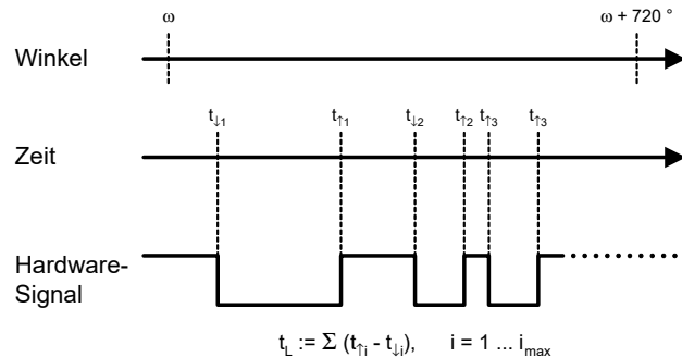
Abb. 32-25 Additive Zeitmessungen mit TMIO-Karte
