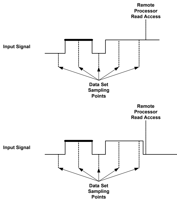
Abb. 16-41 High-Zeit-Messung (der gemessene Puls ist mit fatter Strichstärke hervorgehoben)
