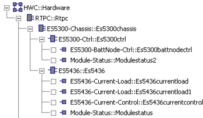
Abb. 29-1 RTIO Hierarchie mit ES5436.1 Current Source Load Board
