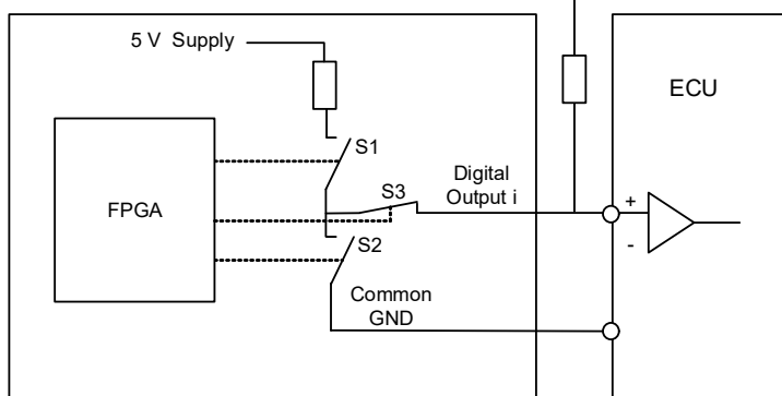
Abb. 23-13 Prinzipschaltbild für die beiden Einstellungen „Pull-Up to +5 V“ und „Open Collector“ in der Registerkarte „Signals“
