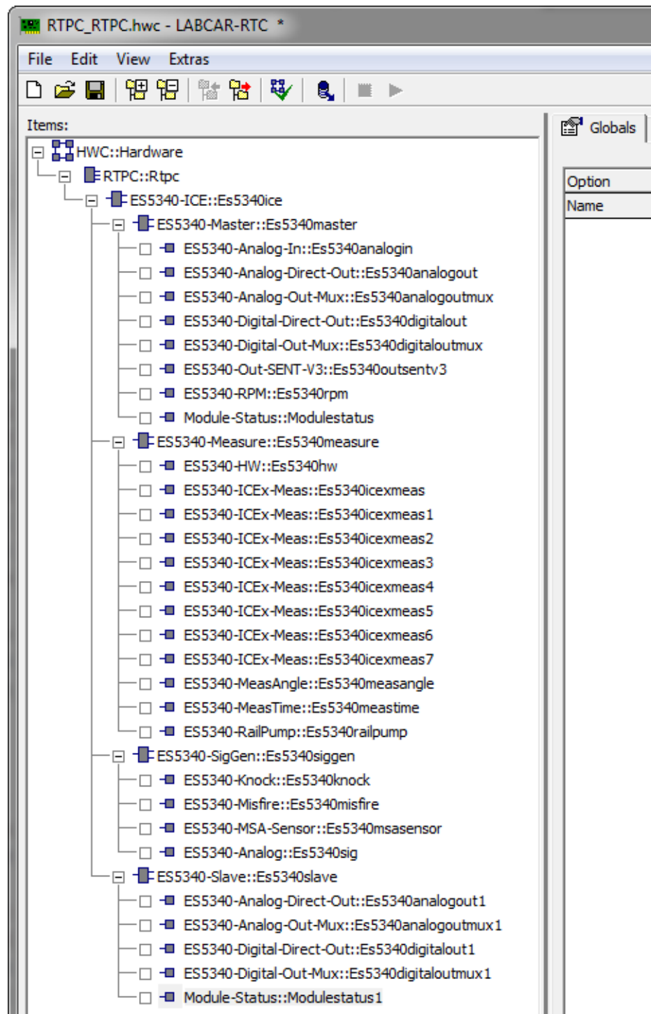
Abb. 23-1 Vollständiger ES5340-ICE RTIO-Baum
