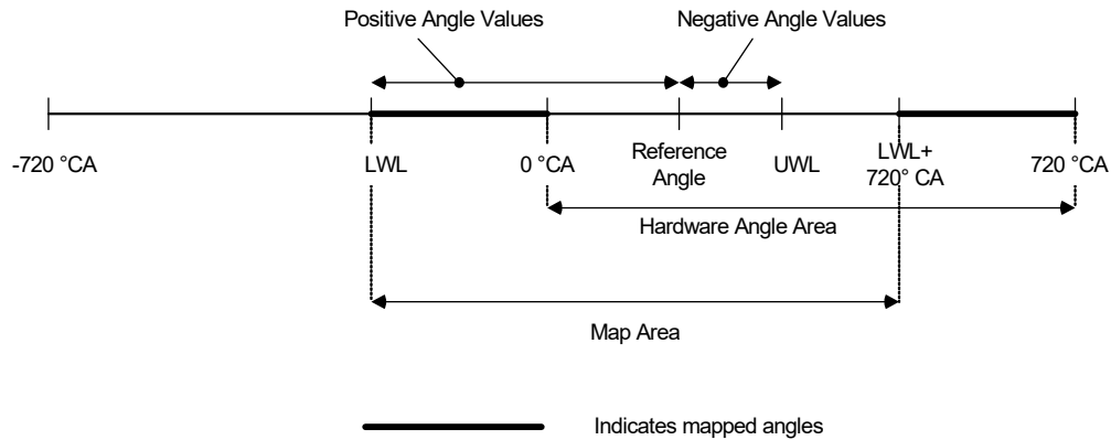
Abb. 23-32 Funktionsweise einer Winkelmessung.
