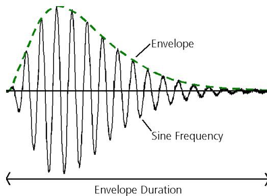
Abb. 32-16 Klopfsignal (durchgezogen) und Einhüllende (gestrichelt)
