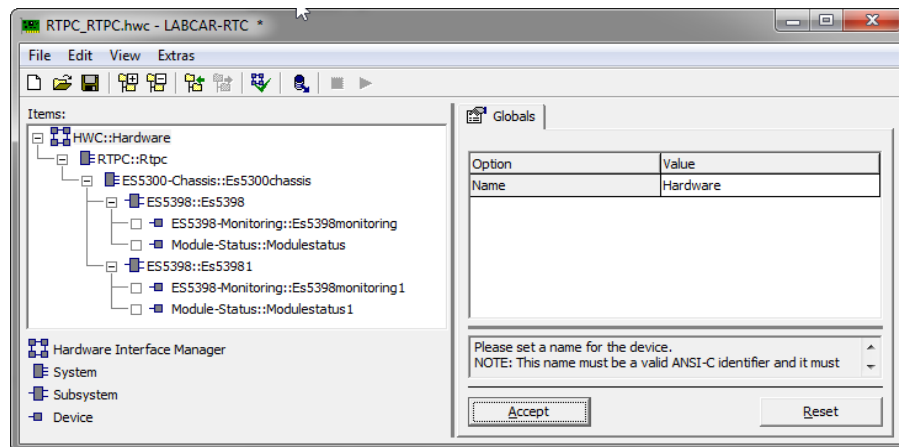
Abb. 28-1 RTIO Hierarchie mit ES5398.1 Fault Insertion Board
