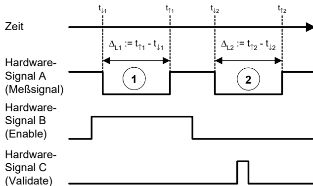
Abb. 32-29 Validierte Zeitmessungen mit TMIO-Karte
