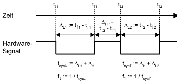
Abb. 32-27 Frequenzmessungen mit TMIO-Karte.
