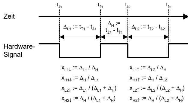
Abb. 32-28 Tastverhältnis-Bestimmung mit TMIO-Karte.
