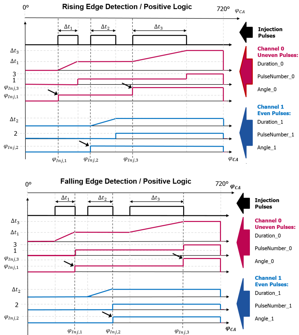
Abb. 23-22 Erfassung der steigenden Flanke und Erfassung der fallenden Flanke für positive Logik
