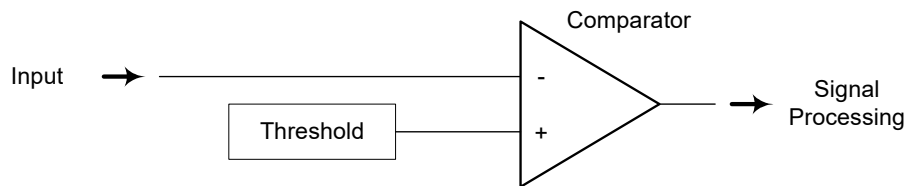
Abb. 9-2 Vereinfachte Darstellung der Eingangsbeschaltung eines -Hardwarekanals
