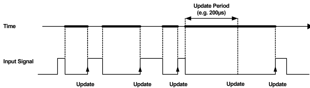
Abb. 9-18 Darstellung der Funktionsweise einer asynchronen additiven Lowzeit-Messung (Messverfahren „Additive Lowtime [µs]“). Die additive Zeit setzt sich aus den fett markierten Zeitsegmenten zusammen. Die Zeitpunkte an denen die Summe im DPRAM aktualisiert wird, sind ebenfalls dargestellt.
