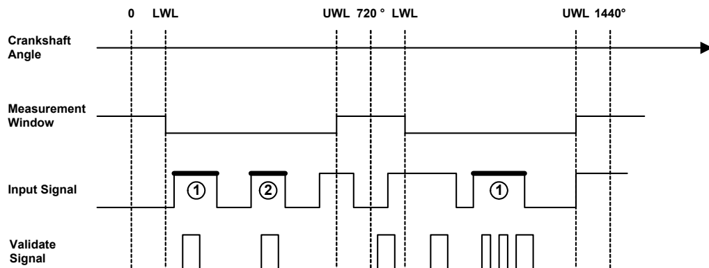
Abb. 23-30 Darstellung der Funktionsweise einer winkelsynchronen Pulsweitenmessung mit Validierungssignal (Messverfahren „Angular: H-Time n-th Pulse (H-Valid.) [μs]“). Validierte Pulse sind mit erhöhter Linienstärke hervorgehoben.
