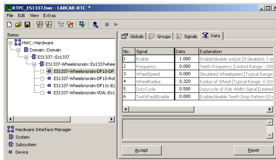
Abb. 12-10 Die Registerkarte „Data“ des ES1337-Wheelsnrsim-DF10-DF11s Device
