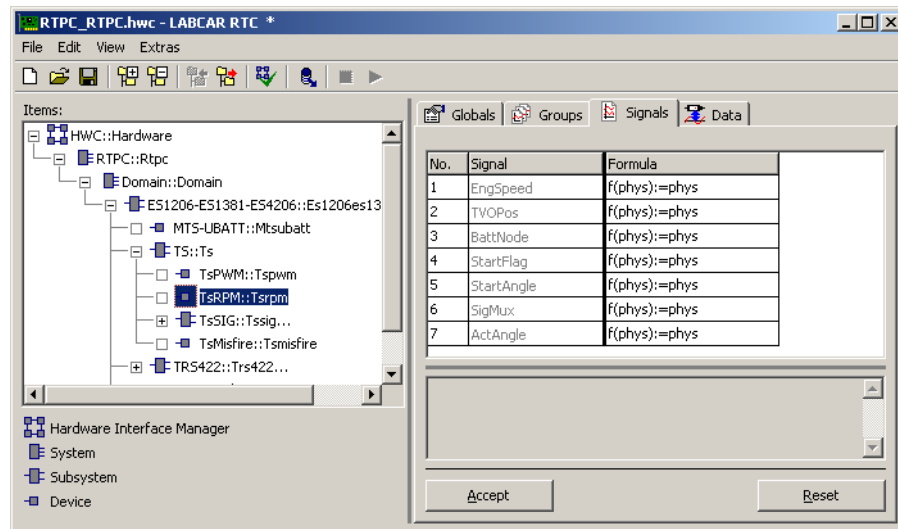
Abb. 29-11 Die Registerkarte „Signals“ des TsRPM Devices
