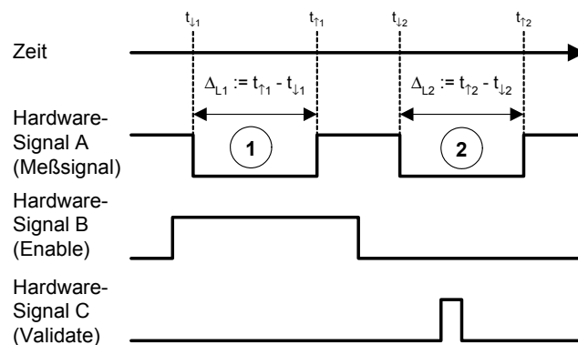
Abb. 29-29 Validierte Zeitmessungen mit TMIO-Karte
