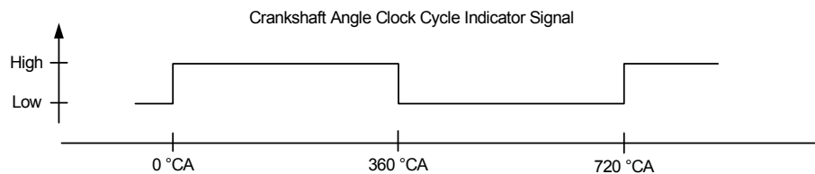
Abb. 11-14 Winkeltakt-Phasen-Indikator-Signal
