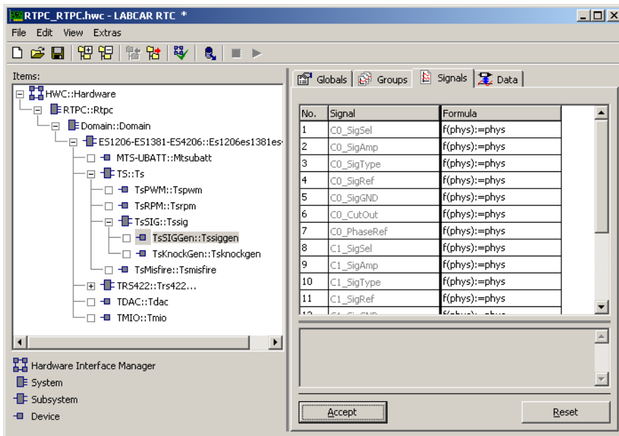
Abb. 29-15 Die Registerkarte „Signals“ des TsSIGGEN Devices
