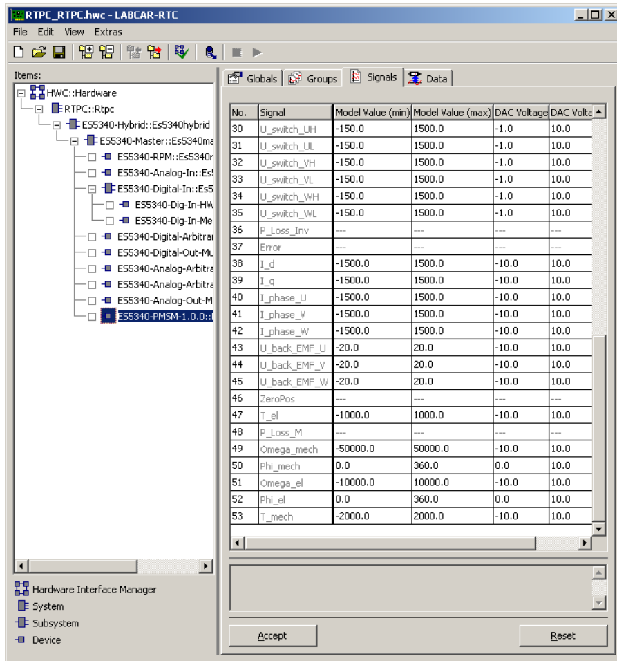
Abb. 22-56 Die Registerkarte „Signals“ des ES5340-PMSM-1.0.0 RTIO-Elements (Teil 2)
