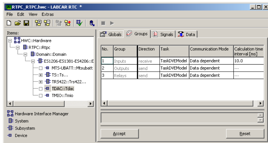
Abb. 29-35 Die Registerkarte „Groups“ des TDAC Devices
