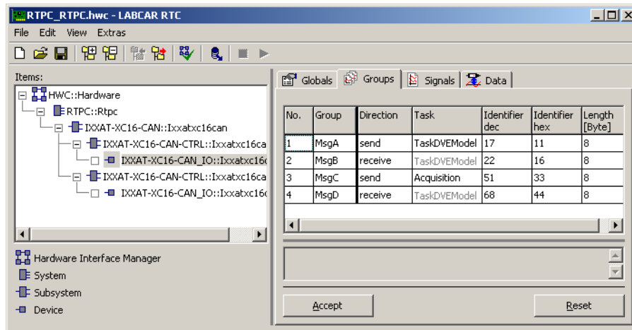
Abb. 28-10 Die Registerkarte „Groups“ des IXXAT-XC16-CAN_IO Devices
