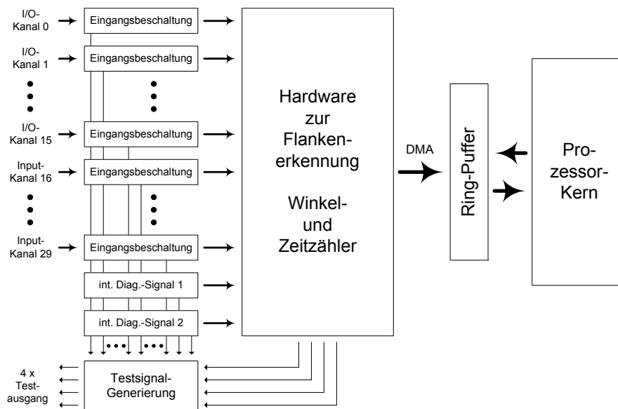
Abb. 29-22 Blockschaltbild TMIO-Karte
