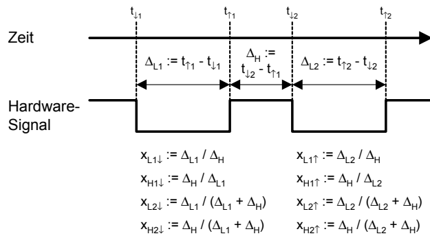
Abb. 29-28 Tastverhältnis-Bestimmung mit TMIO-Karte.
