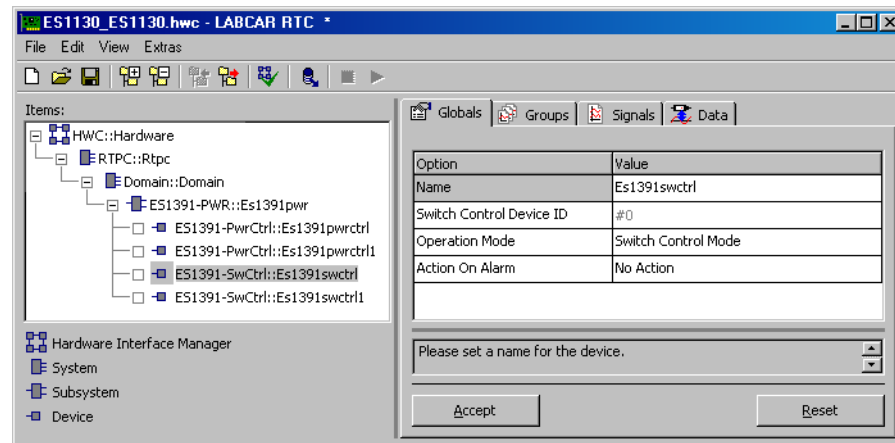
Abb. 14-7 Die Registerkarte „Globals“ des ES1391-SwCtrl Device
