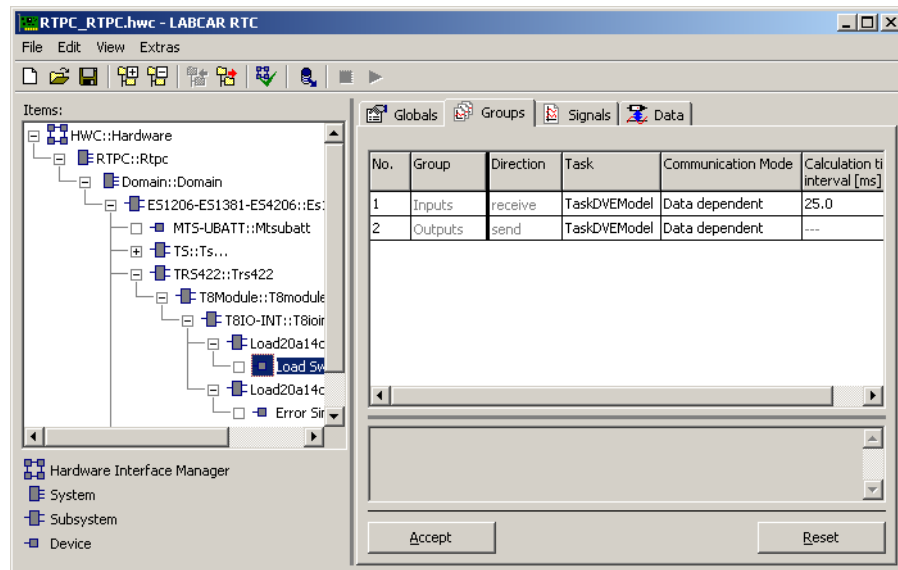
Abb. 29-45 Die Registerkarte „Groups“ des LoadSwitch Devices
