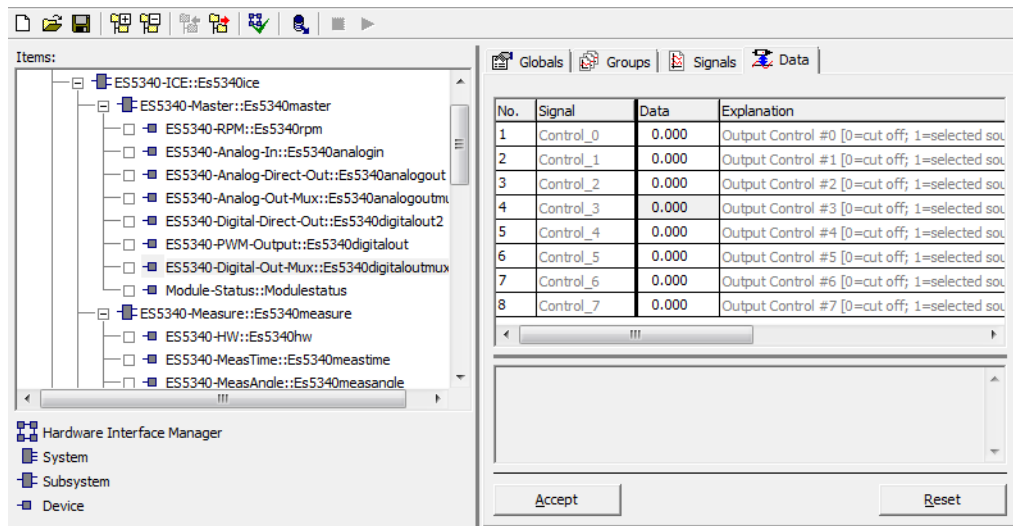
Abb. 23-13 Die Registerkarte „Data“ des ES5340-Digital-Out-Mux RTIO-Elements
