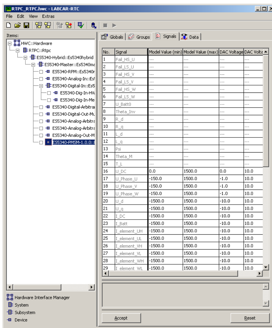
Abb. 22-55 Die Registerkarte „Signals“ des ES5340-PMSM-1.0.0 RTIO-Elements (Teil 1)
