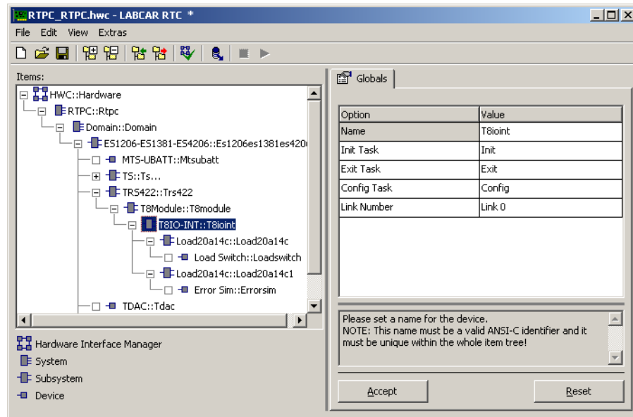
Abb. 29-39 Die Registerkarte „Globals“ des T8IO Subsystems
