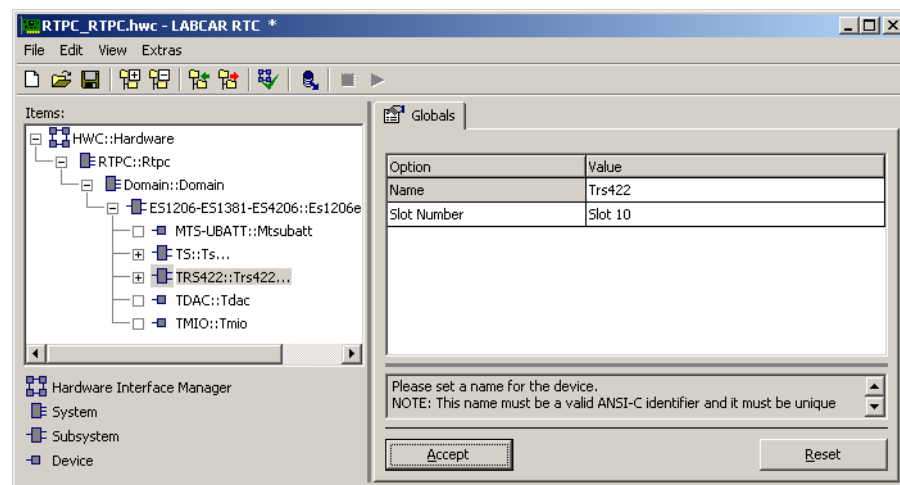
Abb. 29-37 Die Registerkarte „Globals“ des TRS422 Subsystems
