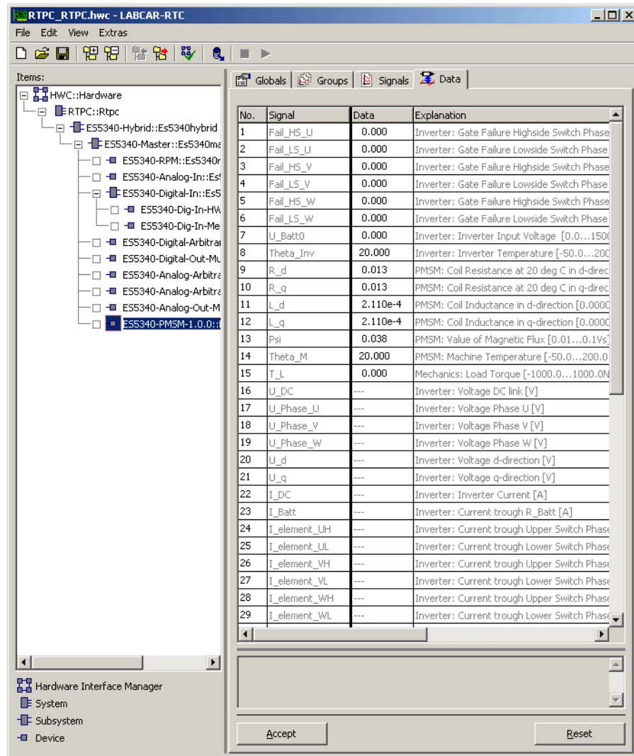
Abb. 22-57 Die Registerkarte „Data“ des ES5340-PMSM-1.0.0 RTIO-Elements (Teil 1)
