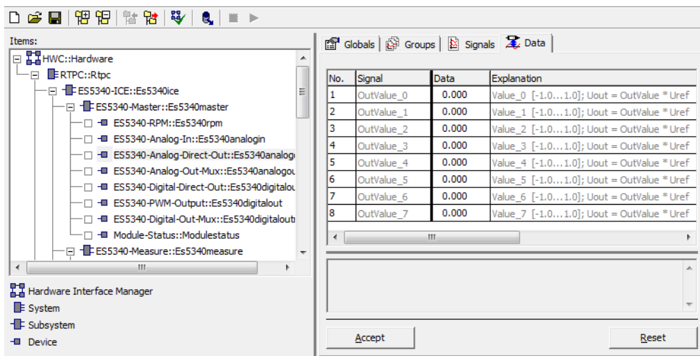
Abb. 23-15 Die Registerkarte „Data“ des ES5340-Analog-Direct-Out RTIO-Elements
