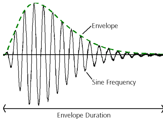
Abb. 29-16 Klopfsignal (durchgezogen) und Einhüllende (gestrichelt)
