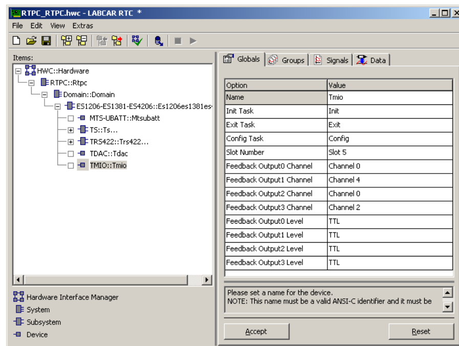
Abb. 29-31 Die Registerkarte „Globals“ des TMIO Devices
