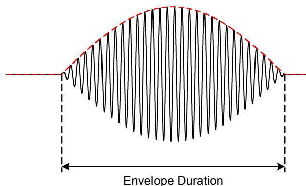
Abb. 23-32 Ein Klopfpaket
