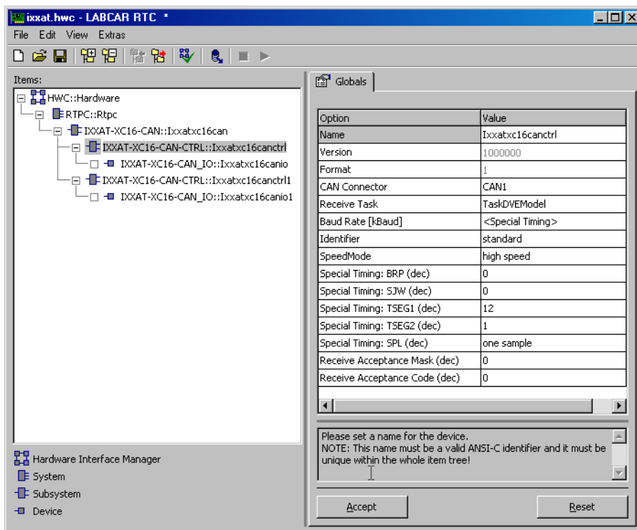
Abb. 28-4 Die Registerkarte „Globals“ eines IXXAT-XC16-CAN-CTRL Subsystems
