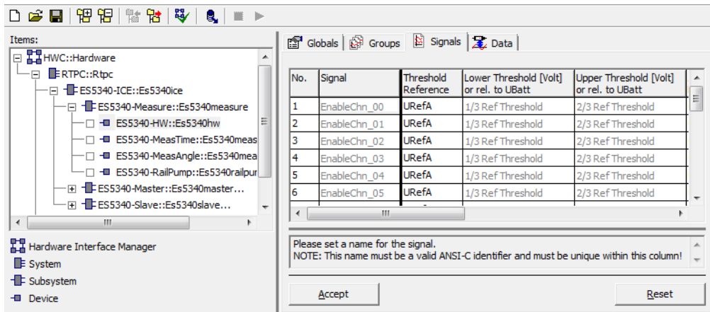
Abb. 23-20 Die Registerkarte „Signals“ des ES5340-HW Device Tab. 23-11 fasst die Eigenschaften der RTIO-Signale zusammen.
