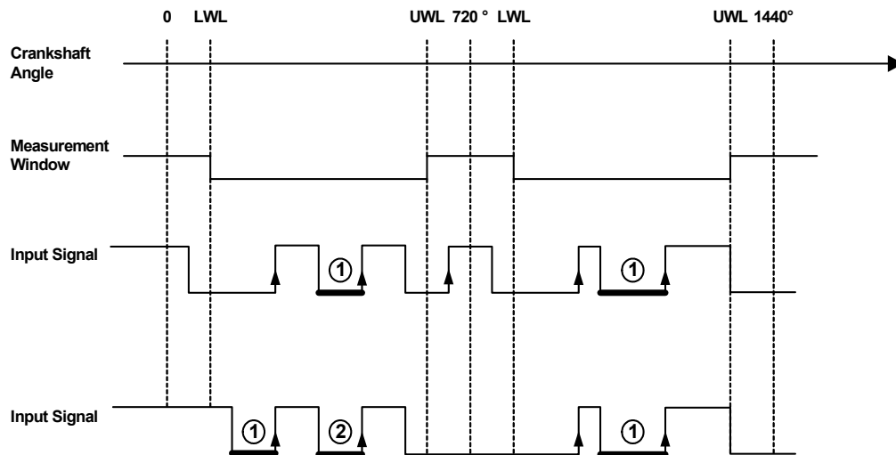
Abb. 23-23 Darstellung der Funktionsweise einer puls-qualifizierten, low-aktiven Pulsweitenmessung (Messverfahren Angular: L-Time n-th Pulse (Pu Qual.) [ \mu s]). Vermessene Pulse bzw. Pulse die gezählt werden sind mit erhöhter Linienstärke hervorgehoben.
