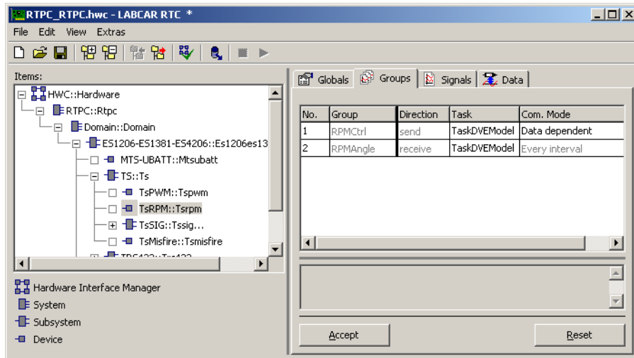
Abb. 29-10 Die Registerkarte „Groups“ des TsRPM Devices
