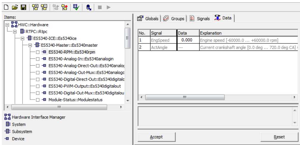
Abb. 23-5 Die Registerkarte „Data“ des ES5340-RPM Device (Viertaktmotor)
