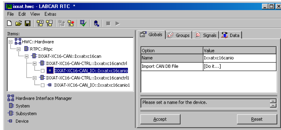
Abb. 28-5 Die Registerkarte „Globals“ des IXXAT-XC16-CAN_IO Devices Import CAN DB File
