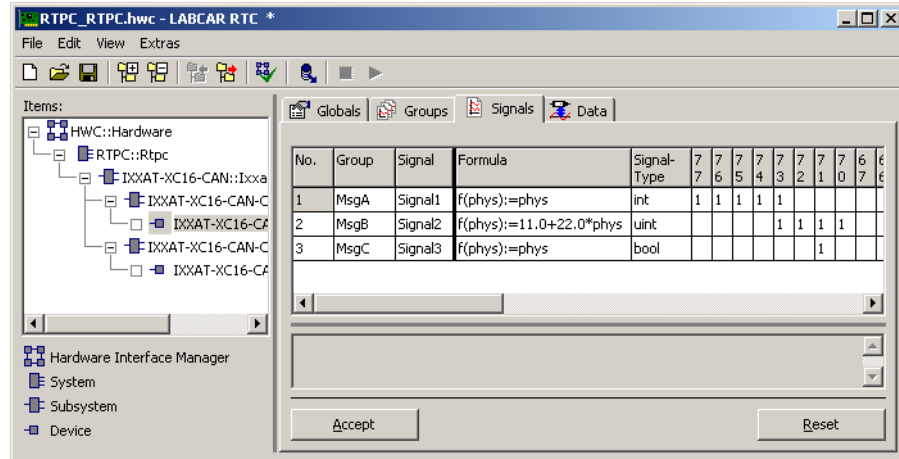
Abb. 28-11 Die Registerkarte „Signals“ des IXXAT-XC16-CAN_IO Devices
