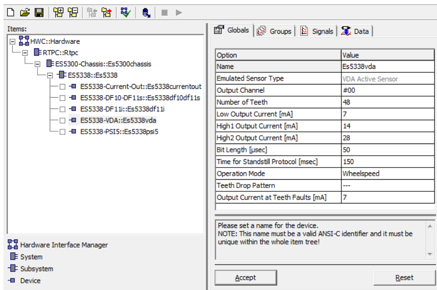
Abb. 21-10 Die Registerkarte „Globals“ des ES5338-VDA Device
