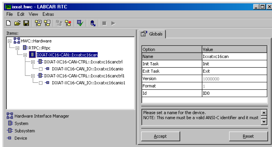
Abb. 28-3 Die Registerkarte „Globals“ des IXXAT-XC16-CAN Subsystems mit versteckten Optionen
