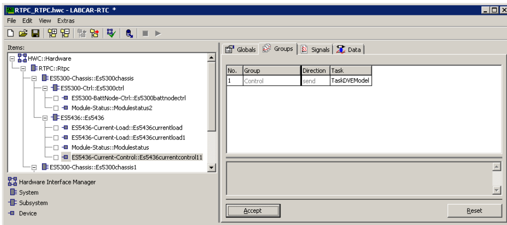
Abb. 27-9 Die Registerkarte "Groups" des ES5436-Current-Control-Device Das ES5436-Current-Control-Item implementiert eine Send-Signalgruppe zum schnellen Verändern der Stromwerte einzelner Lastkanäle.
