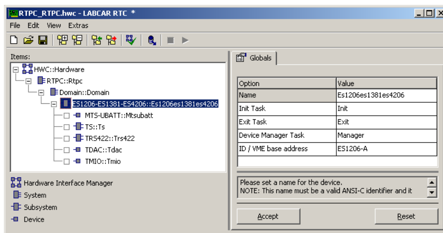
Abb. 29-1 Die Registerkarte „Globals“ des ES4205 / ES1206-ES1381-ES4206 Subsystems
