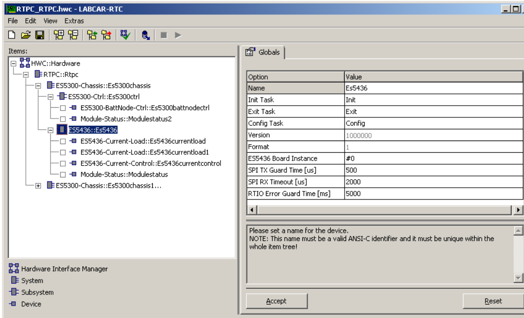
Abb. 27-3 Die Registerkarte "Globals" des ES5436 Subsystems (alle Optionen sichtbar)
