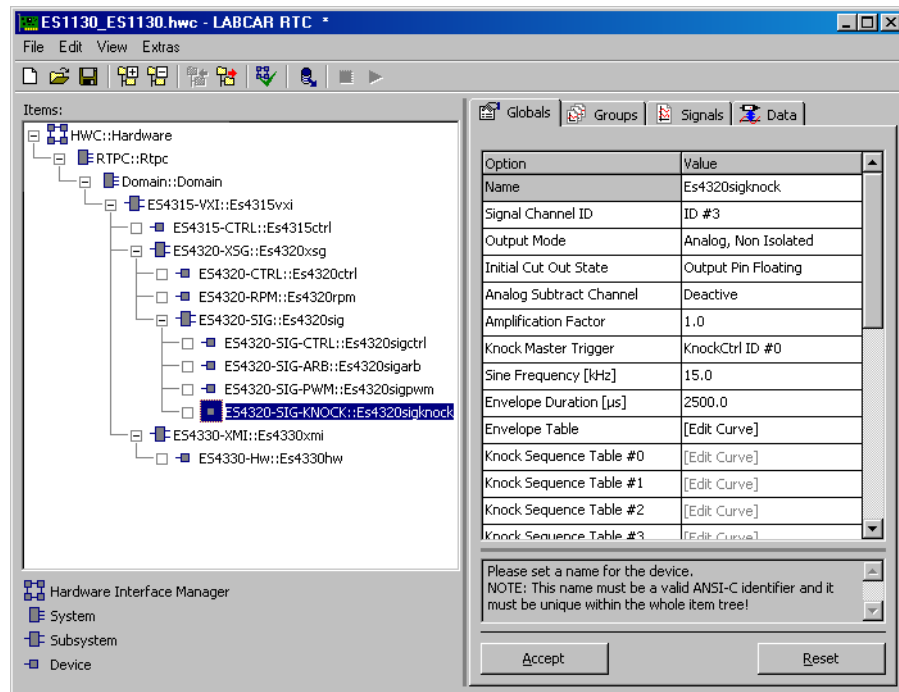
Abb. 17-21 Die Registerkarte „Globals“ des ES4320-SIG-KNOCK Devices
