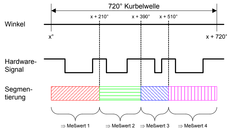
Abb. 29-30 Winkelsegmentierung mit TMIO-Karte
