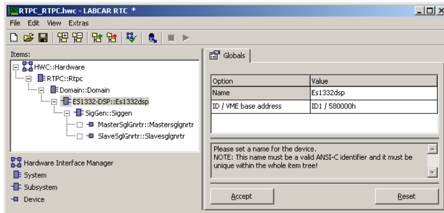
Abb. 7-2 Die Registerkarte „Globals“ des ES1332-DSP Subsystems
