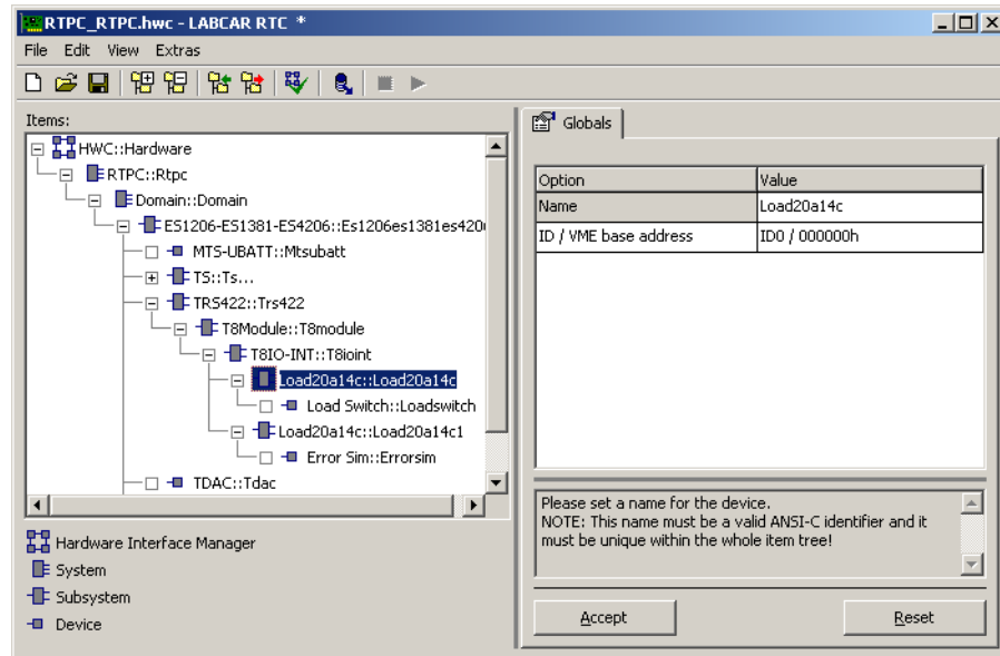
Abb. 29-40 Die Registerkarte „Globals“ des Load20A14C Subsystems ID / VME base address
