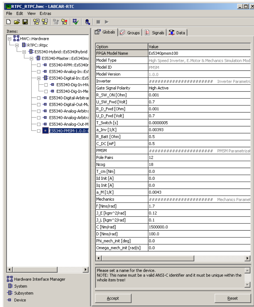
Abb. 22-54 Die Registerkarte „Globals“ des ES5340-PMSM-1.0.0 RTIO-Elements
