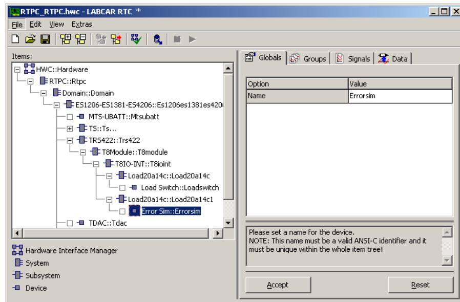
Abb. 29-41 Die Registerkarte „Globals“ des ErrorSim Devices
