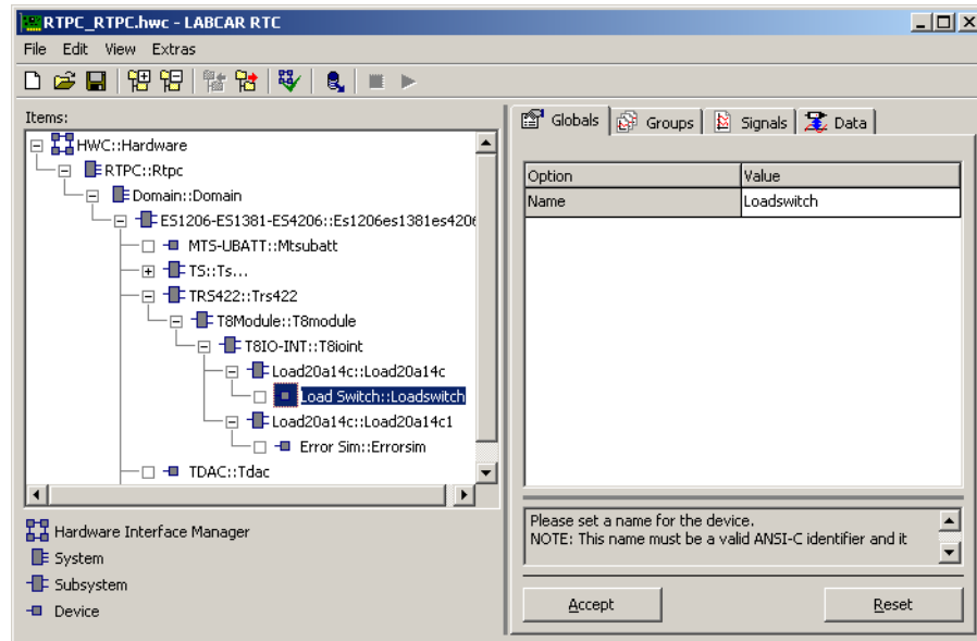
Abb. 29-44 Die Registerkarte „Globals“ des LoadSwitch Devices
