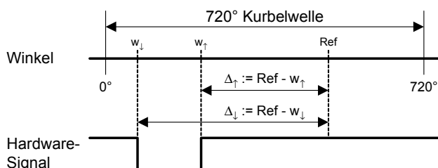
Abb. 29-23 Winkelmessungen mit der TMIO-Karte
