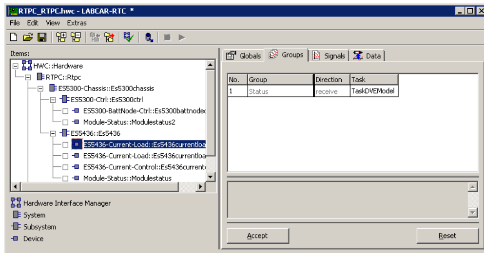
Abb. 27-5 Die Registerkarte "Groups" des ES5436-Current-Load Device Das ES5436-Current-Load-Device implementiert eine Receive-Signalgruppe für Pegel und Fehlerinformationen.
