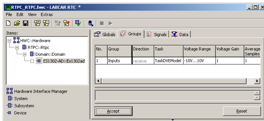
Abb. 3-2 Die Registerkarte „Groups“ des ES1302-AD Device
