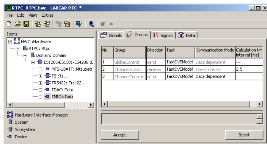
Abb. 29-32 Die Registerkarte „Groups“ des TMIO Devices
