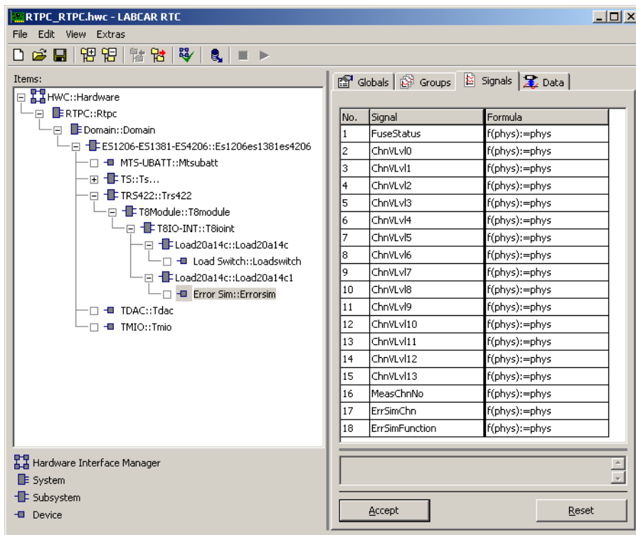
Abb. 29-43 Die Registerkarte „Signals“ des ErrorSim Devices
