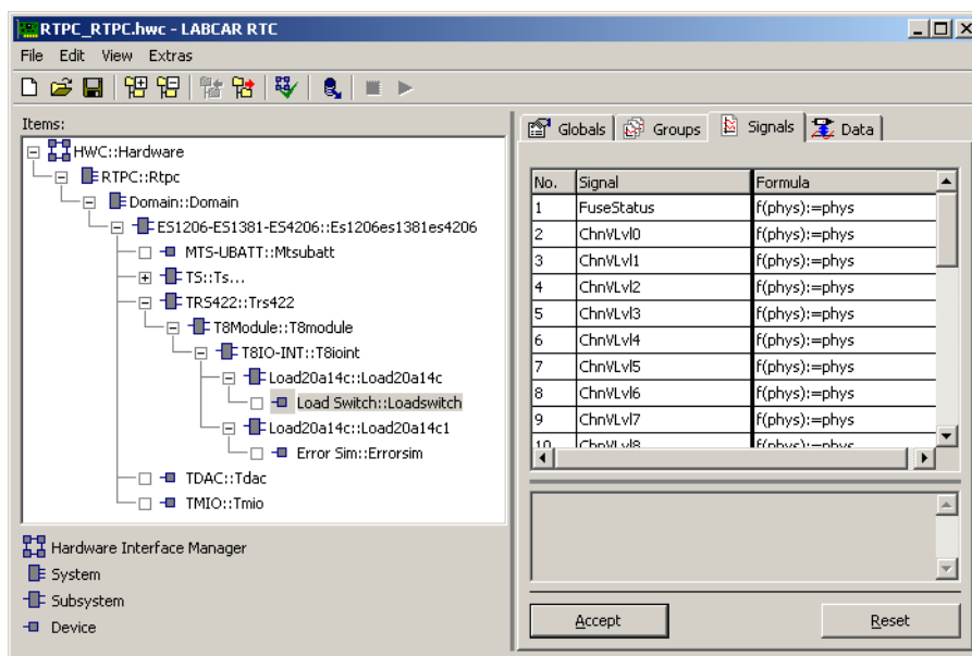
Abb. 29-46 Die Registerkarte „Signals“ des LoadSwitch Devices
