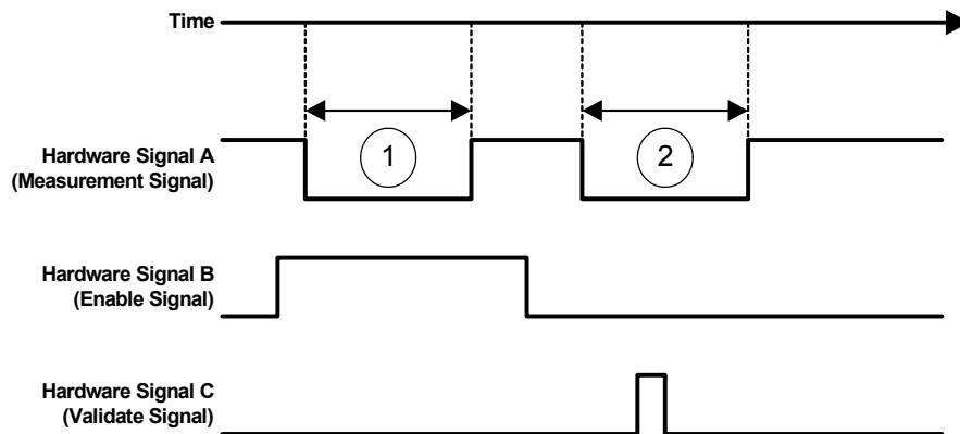
Abb. 11-21 Pulsweitenmessungen mit Enable- und Validierungssignal
