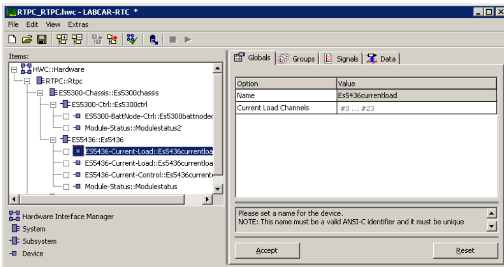
Abb. 27-4 Die Registerkarte "Globals" des ES5436-Current-Load-Device
