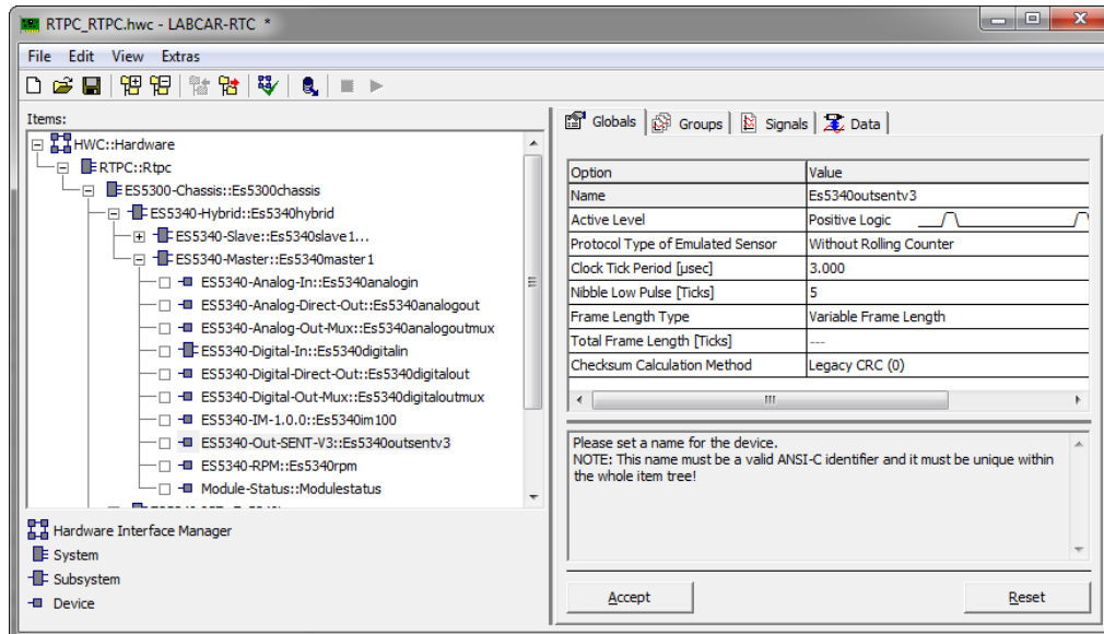
Abb. 22-51 Die Registerkarte „Globals“ des ES5340-Out-SENT Devices
