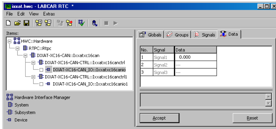
Abb. 28-12 Die Registerkarte „Data“ des IXXAT-XC16-CAN_IO Devices Man erkennt in der Registerkarte „Data“ (Abb. 28-12 - „offline“ Modus), dass das Signal „Signal1“ dazu verwendet wird, um eine CAN-Botschaft zu versenden. Im „Data“-Feld können im „online“ Modus die Nutzdaten belegt werden. Im „offline“ Modus sind die „Data“-Felder der Empfangsbotschaften „Signal2“ und „Signal3“ nicht aktiv, im „online“ Modus werden dort die empfangenen Nutzdaten der entsprechenden CAN-Botschaften dargestellt.
