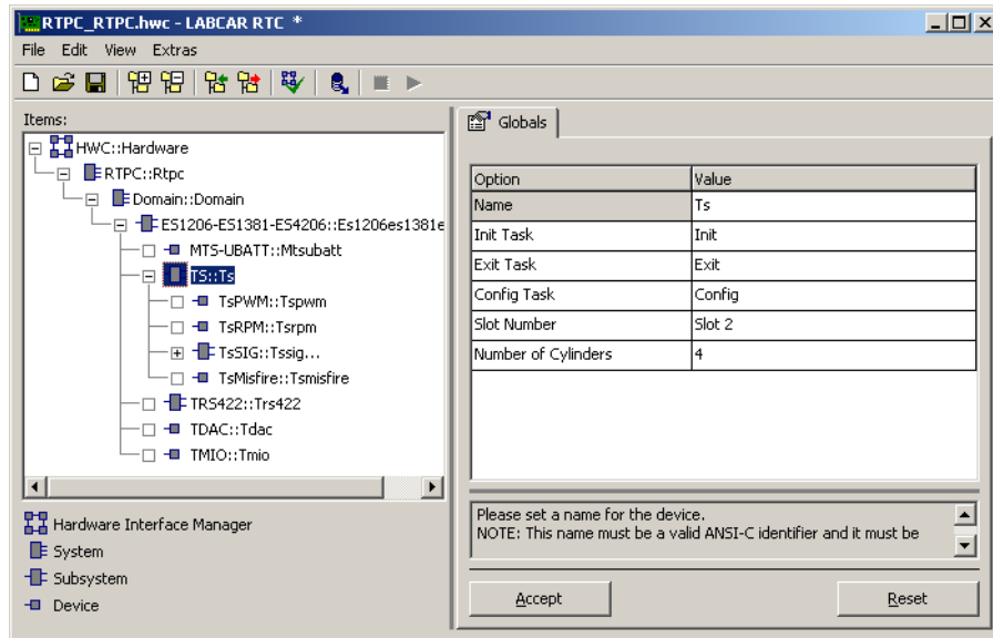
Abb. 29-5 Die Registerkarte „Globals“ des TS Subsystems
