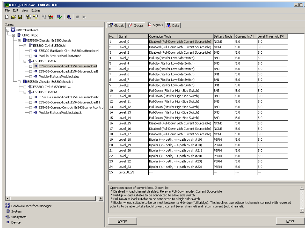
Abb. 27-6 Die Registerkarte "Signals" des ES5436-Current-Load-Device In diesem Register können für jeden der 24 Kanäle folgende Parameter eingestellt werden:
