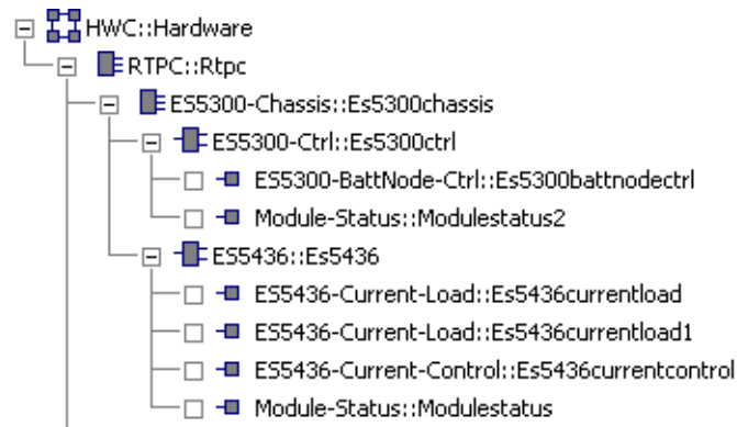
Abb. 27-1 RTIO Hierarchie mit ES5436.1 Current Source Load Board
