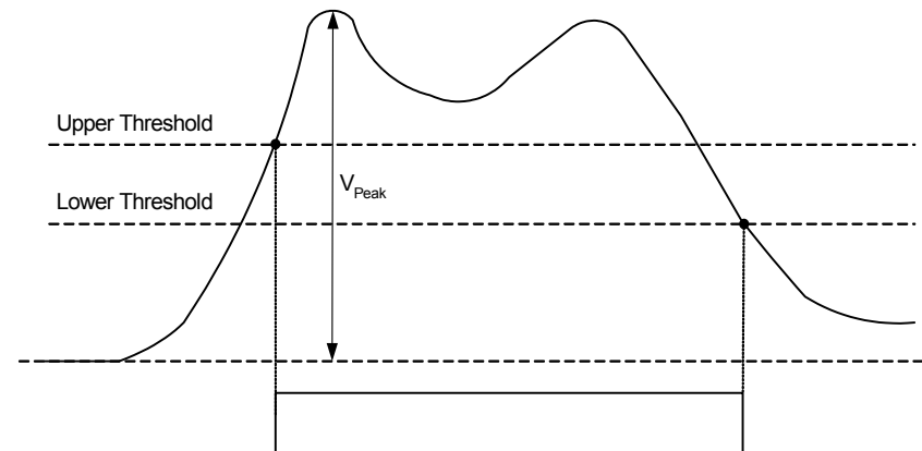
Abb. 11-6 Spitzenwertvermessung
