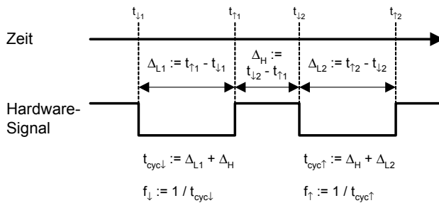
Abb. 29-27 Frequenzmessungen mit TMIO-Karte.
