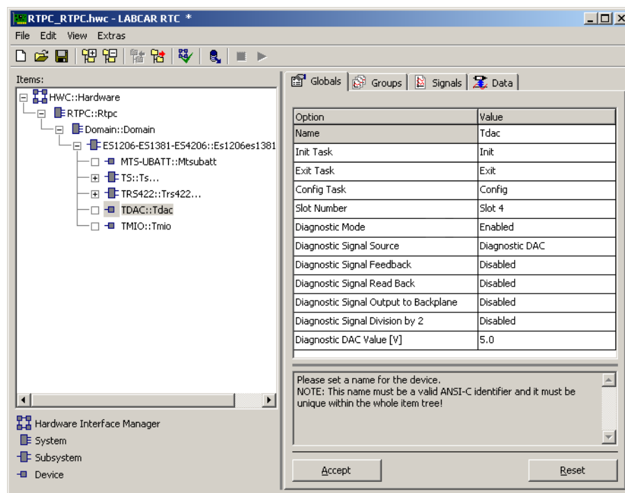
Abb. 29-34 Die Registerkarte „Globals“ des TDAC Devices
