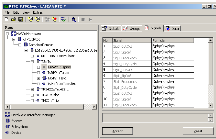
Abb. 29-8 Die Registerkarte „Signals“ des TsPWM Devices
