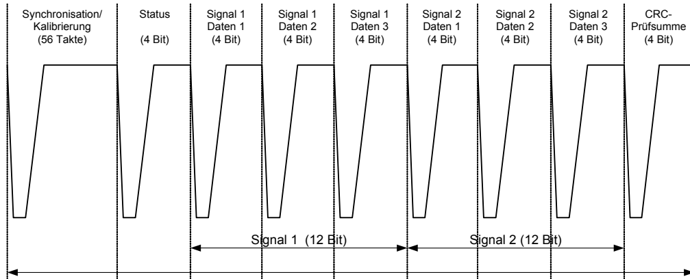
Abb. 20-15 Format eines Signals gemäß SENT-Datenprotokoll
