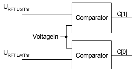
Abb. 11-3 Komparatorstufe für die Messung der Signalanstiegs- und -abfallzeiten
