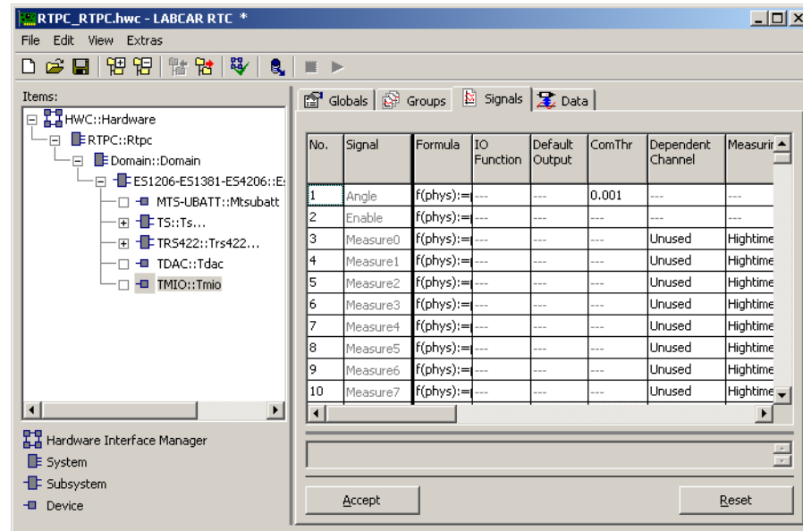
Abb. 29-33 Die Registerkarte „Signals“ des TMIO Devices
