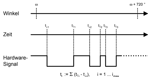
Abb. 29-25 Additive Zeitmessungen mit TMIO-Karte
