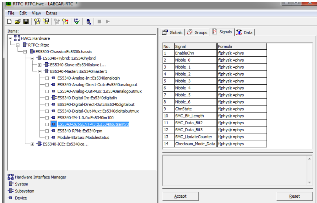
Abb. 22-52 Die Registerkarte „Signals“ des ES5340-Out-SENT Devices
