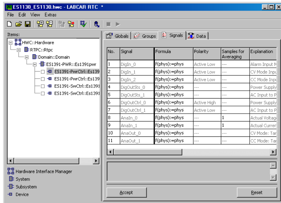
Abb. 14-6 Die Registerkarte „Signals“ des „ES1391-PwrCtrl“ Device (bei Fernsteuerung eines Takasago-Netzteils)
