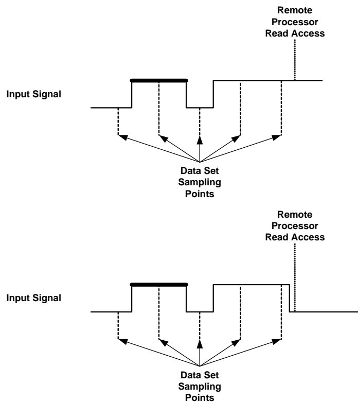
Abb. 16-41 High-Zeit-Messung (der gemessene Puls ist mit fester Strichstärke hervorgehoben)
