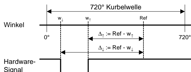
Abb. 28-23 Winkelmessungen mit der TMIO-Karte
