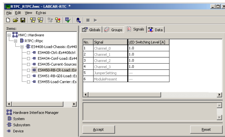
Abb. 18-11 Die Registerkarte „Signals“ des ES4450-RB-CR-Load Device
