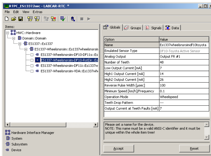
Abb. 12-11 Die Registerkarte „Globals“ des ES1337-Wheelsnsrsim-DF10-RotDir Device
