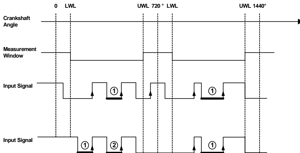
Abb. 11-20 Darstellung der Funktionsweise einer puls-qualifizierten, low-aktiven Pulsweitenmessung (Messverfahren Angular: L-Time n-th Pulse (Pu Qual.) [ \mu s]). Vermessene Pulse bzw. Pulse die gezählt werden sind mit erhöhter Linienstärke hervorgehoben.
