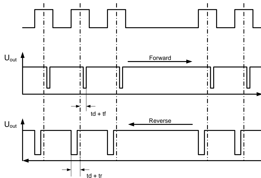
Abb. 23-42 Kurbelwellenzähne und Sensorsignale bei einem MSA-Sensor
