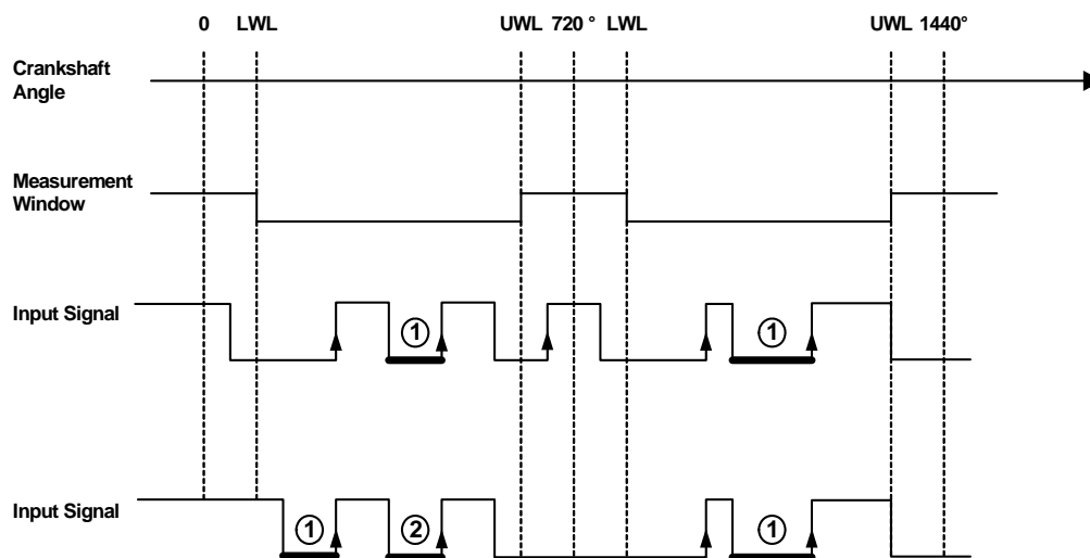
Abb. 23-23 Darstellung der Funktionsweise einer puls-qualifizierten, low-aktiven Pulsweitenmessung (Messverfahren Angular: L-Time n-th Pulse (Pu Qual.) [ \mu s]). Vermessene Pulse bzw. Pulse die gezählt werden sind mit erhöhter Linienstärke hervorgehoben.
