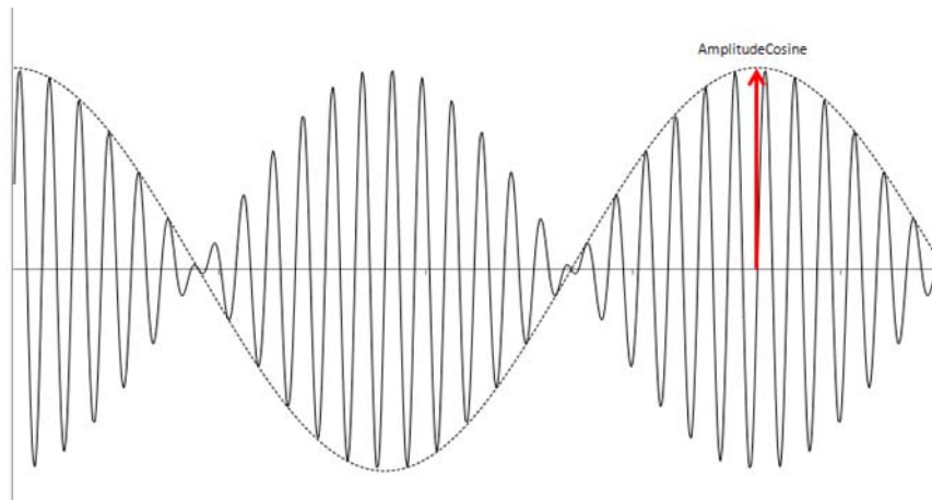
Abb. 22-44 Resolver: Kosinuskanal
