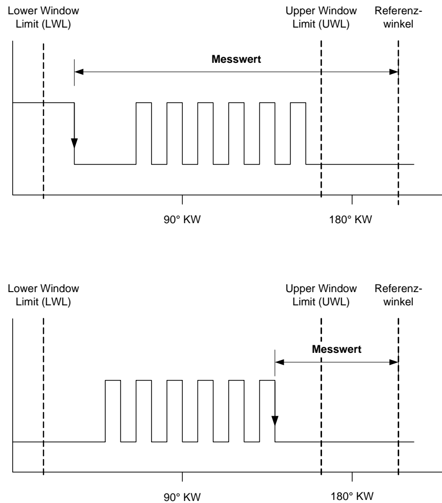
Abb. 23-30 Messwerte bei „Angle of First Falling Edge of Pulse Sequence“ (oben) und „Angle of Last Falling Edge of Pulse Sequence“ (unten)
