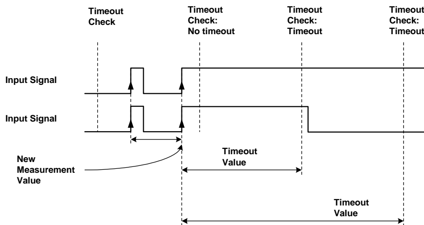
Abb. 17-50 Frequenz- und Zykluszeitmessung an ansteigenden Flanken: Darstellung der Messwertberechnung im Timeout-Fall (der Messwert ist in der Darstellung als „Timeout Value“ bezeichnet) bei den „... InpDep“-Verfahren zur Timeout-Überwachung
