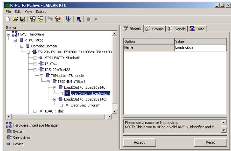
Abb. 28-44 Die Registerkarte „Globals“ des LoadSwitch Devices
