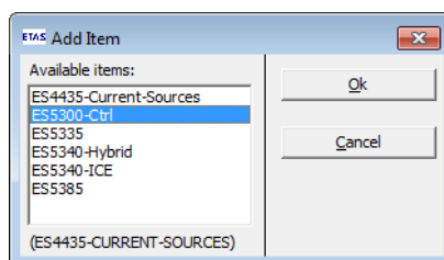
Abb. 19-1 Die unter einem ES5300-Chassis verfügbaren RTIO Elemente
