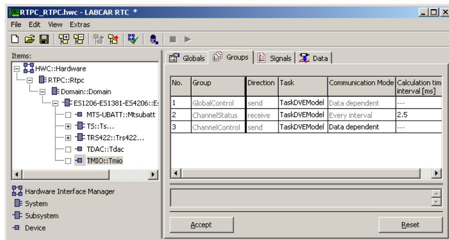
Abb. 28-32 Die Registerkarte „Groups“ des TMIO Devices
