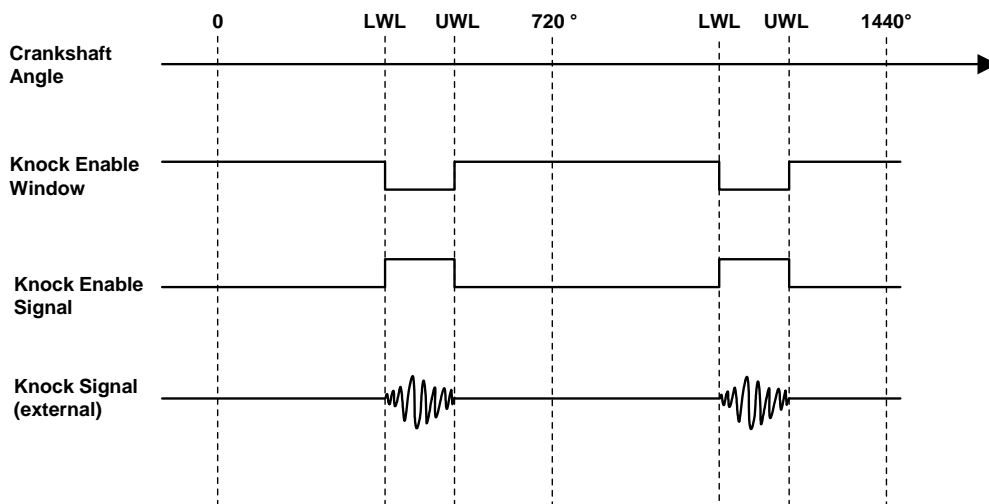
Abb. 8-4 High-aktives Klopf-Enable-Signal zur Aktivierung und Deaktivierung eines externen Klopfgenerators.
