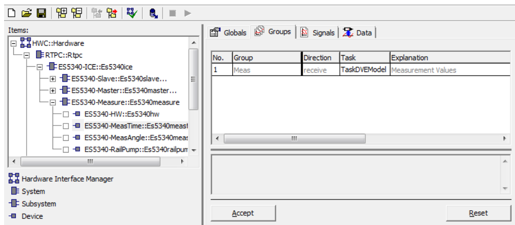
Abb. 23-21 Die Registerkarte „Groups“ des ES5340-MeasTime Device Die RTIO-Signale der Signalgruppe „Meas“
