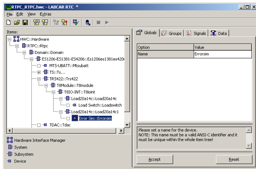
Abb. 28-41 Die Registerkarte „Globals“ des ErrorSim Devices
