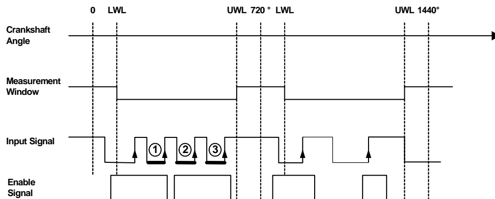
Abb. 11-22 Darstellung der Funktionsweise einer winkelsynchronen Pulsweitenmessung mit Enable-Signal (Messverfahren „Angular: L-Time n-th Pulse (H-Enable) [μs]“). Aktivierte Pulse sind mit erhöhter Linienstärke hervorgehoben.
