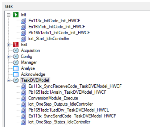
Abb. 3-43 Das Feld „Tasks“ des Registers „OS Configuration“
