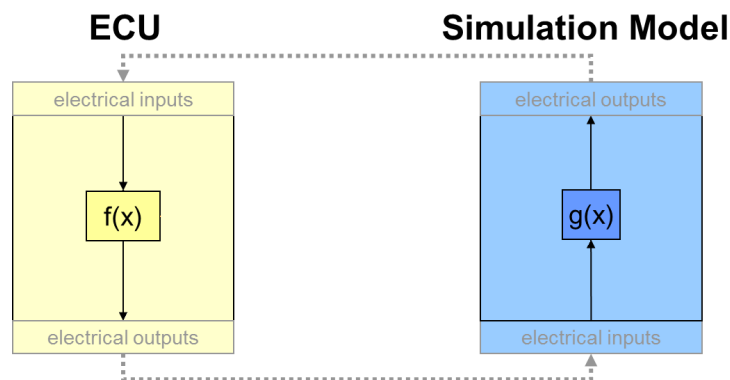
Abb. 3-23 Aufbau eines HiL-Systems
