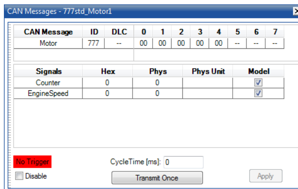
Abb. 3-15 Message-GUI für eine Send-Message
