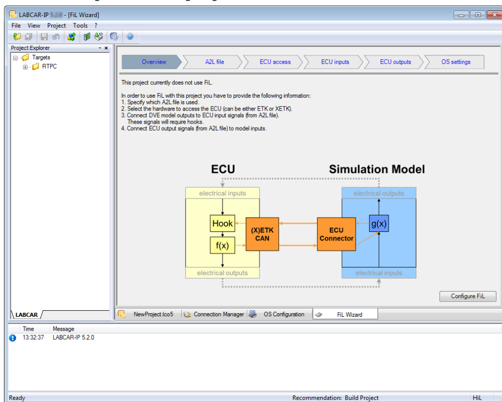
Abb. 3-25 Die Startseite des FiL Wizards
