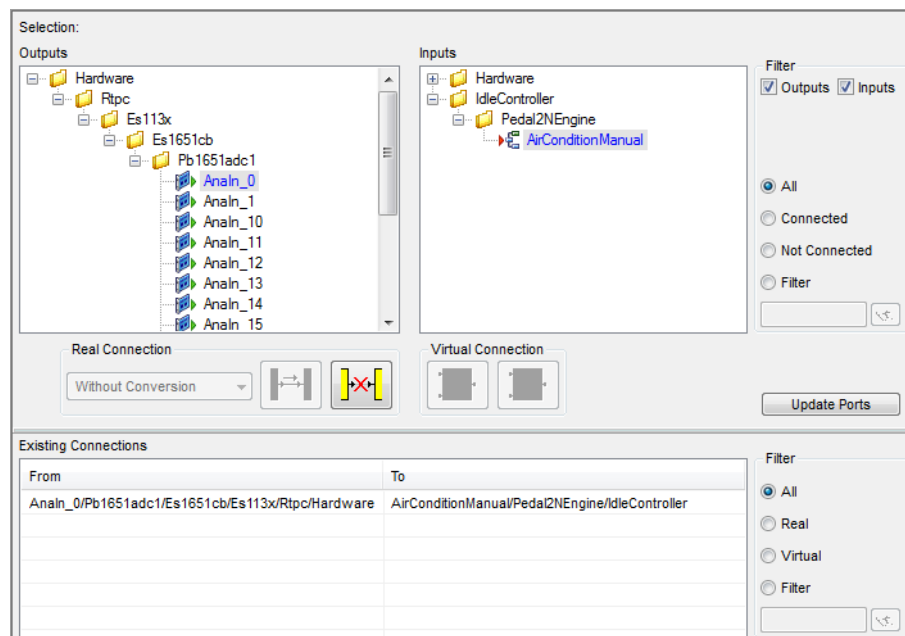
Abb. 3-37 Das Bedienfenster des Connection Manager
