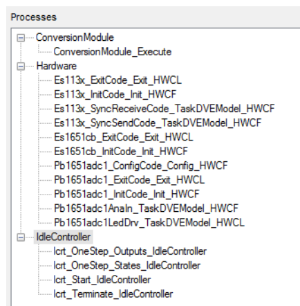
Abb. 3-42 Das Feld „Processes“ des Registers „OS Configuration“
