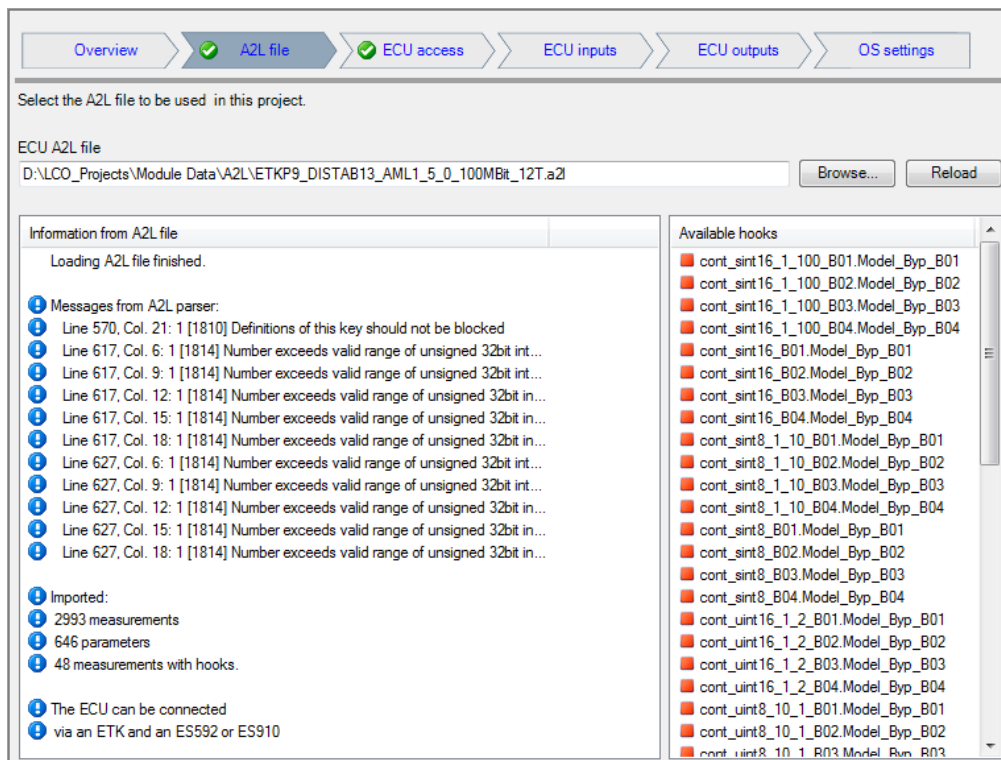
Abb. 3-26 Auswahl der A2L-Datei
