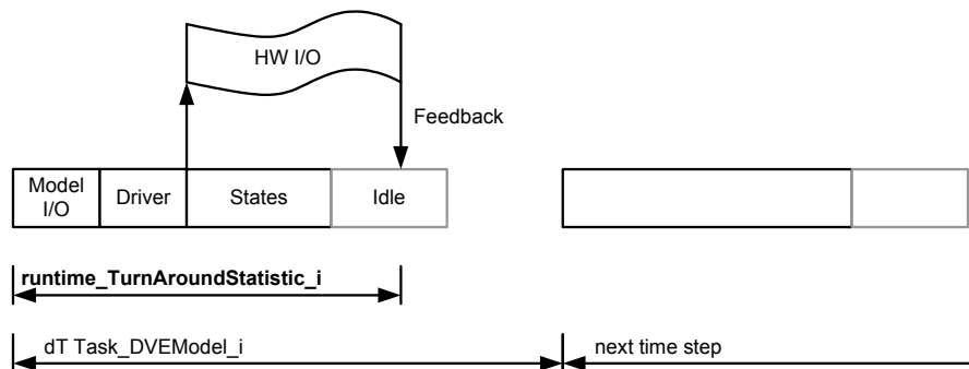
Abb. 3-40 Berechnung der Größe „runtime_TurnaroundStatistic“
