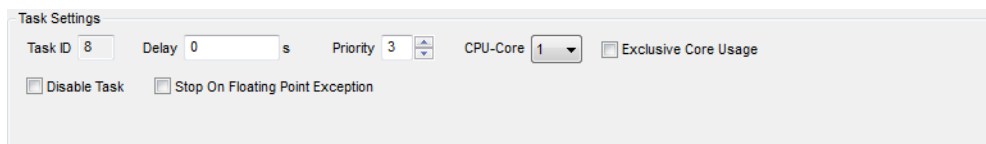
Abb. 3-41 Task-Einstellungen
