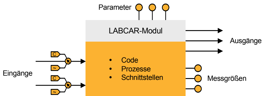
Abb. 3-1 Ein LABCAR-Modul
