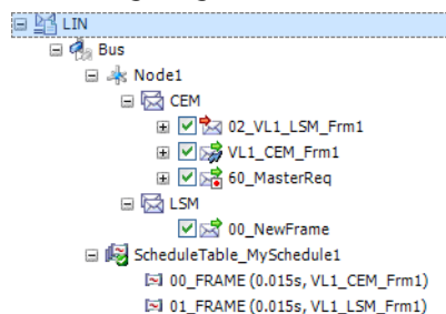
Abb. 3-18 Das LIN-Netzwerk
