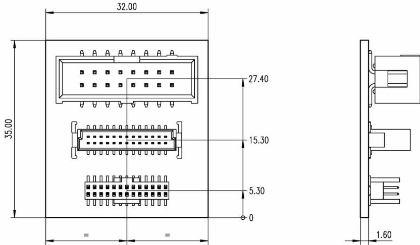
Fig. 2-2 ETAF5 PCB
