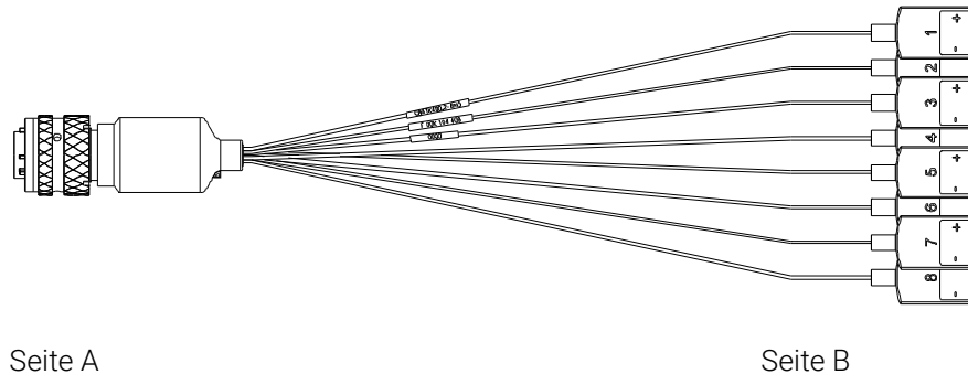
Abb. 8-17 Kabel CBATx400.x
