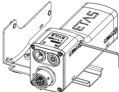
Abb. 5-9 Befestigung an einem ES4xx-Haltewinkel (links) mit den integrierten Montageelementen
