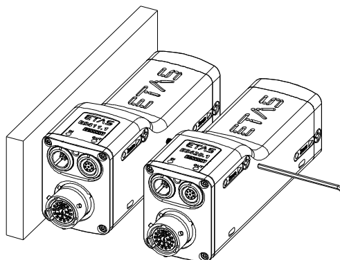
Abb. 5-8 Verbinden mit weiteren Modulen
