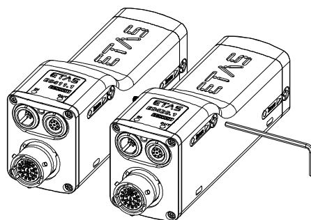
Abb. 5-5 ES400-Module mit den integrierten Montageelementen verbinden
