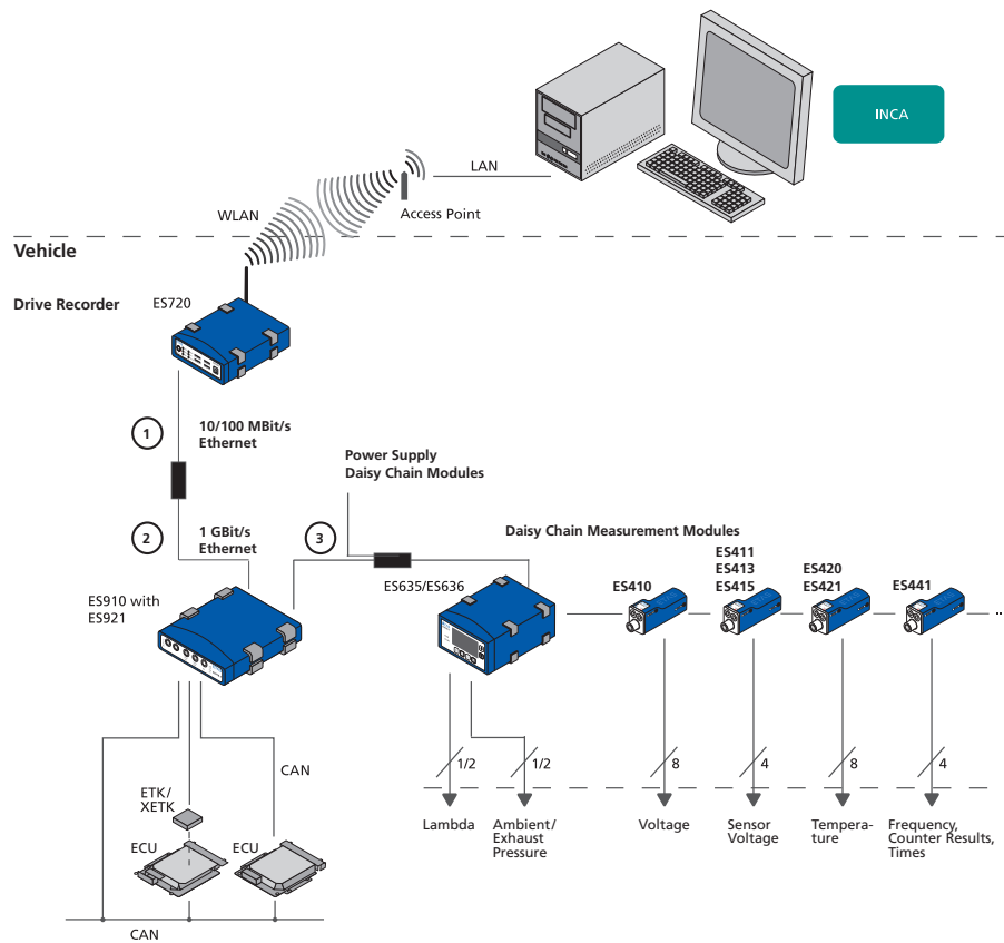
Abb. 5-19 ES400 Module mit ES910.3 und Drive Recorder (Rapid Prototyping)
