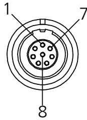
Abb. 7-3 Anschluss „OUT“
