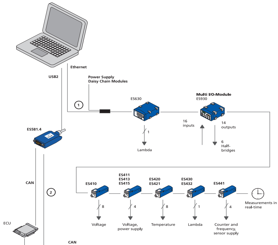
Abb. 5-20 ES400 Module mit ETAS RTPRO-PC (Rapid Prototyping)
