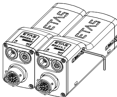
Abb. 5-6 Miteinander verbundene ES400-Module
