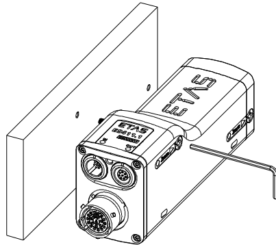
Abb. 5-7 Befestigung an anderen Bauteilen mit den integrierten Montageelementen
