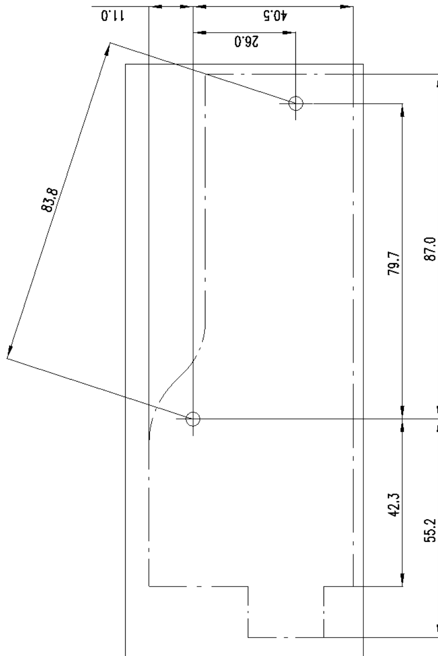
Abb. 5-13 Bohrschablone
