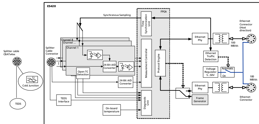
Abb. 4-2 Blockdiagramm
