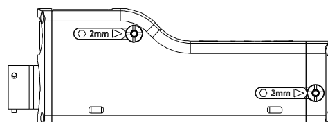
Abb. 5-3 Zugang zu den integrierten Montageelementen
