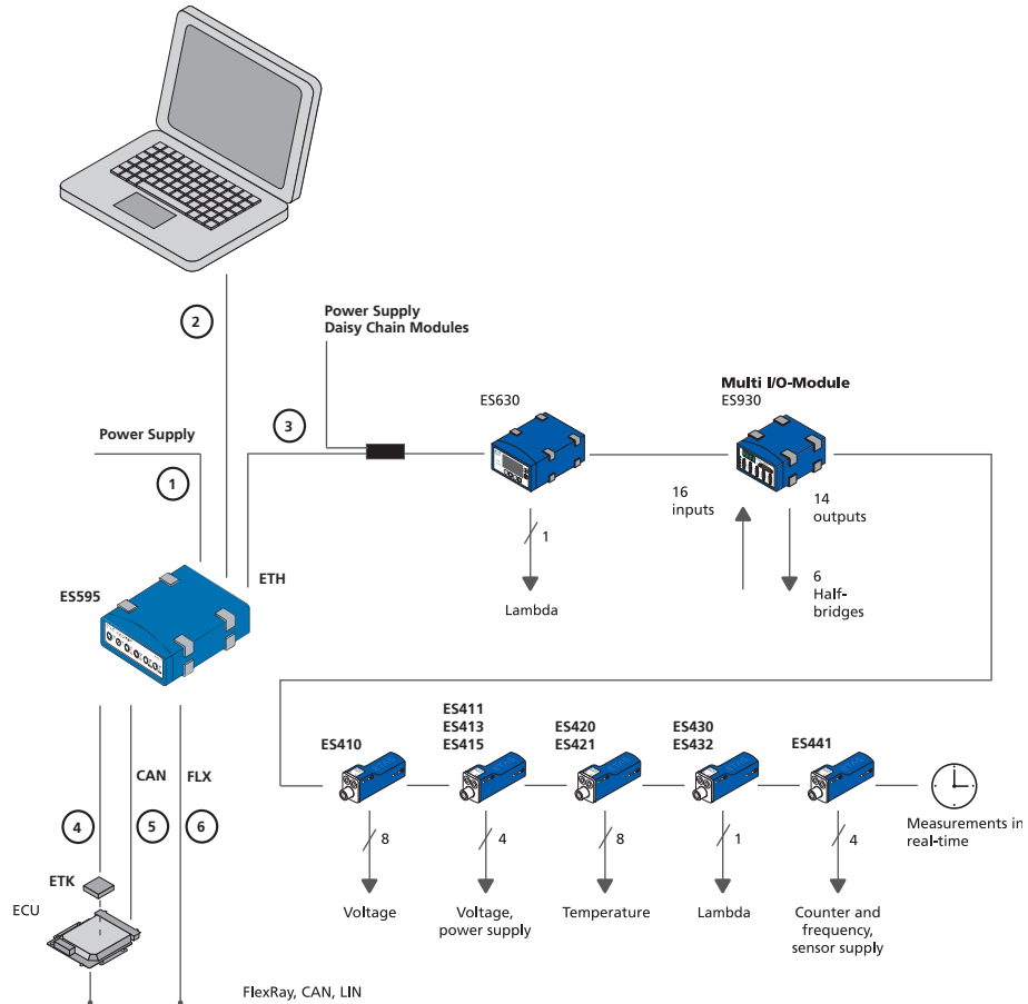
Abb. 5-16 ES400 Module mit weiteren ETAS Modulen (Measurement and Calibration)
