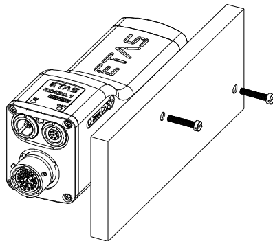
Abb. 5-10 Befestigung an anderen Bauteilen mit zusätzlichen Schrauben
