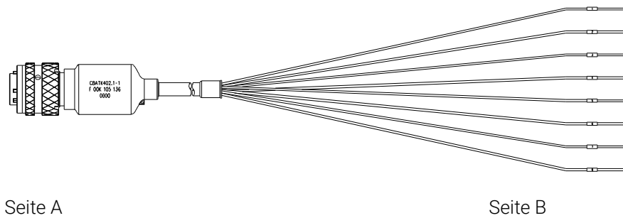
Abb. 8-19 Kabel AS_CBATK402.1
