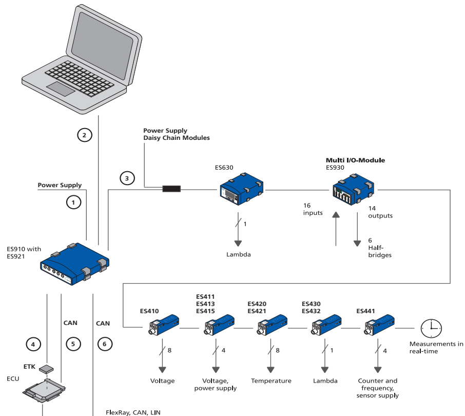
Abb. 5-18 ES400 Module mit ES910.3 (Rapid Prototyping)
