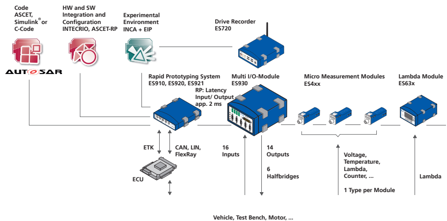
Abb. 5-15 ES400 Module mit ES910 und weiteren ETAS Modulen für Rapid Prototyping-Applikationen
