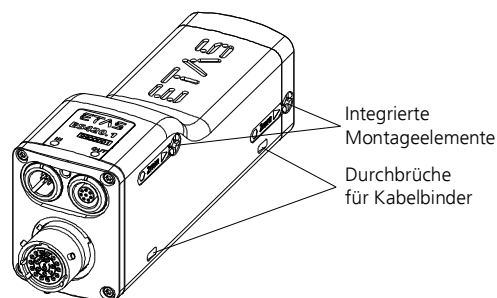
Abb. 5-2 Befestigungsmöglichkeiten an den ES400-Modulen
