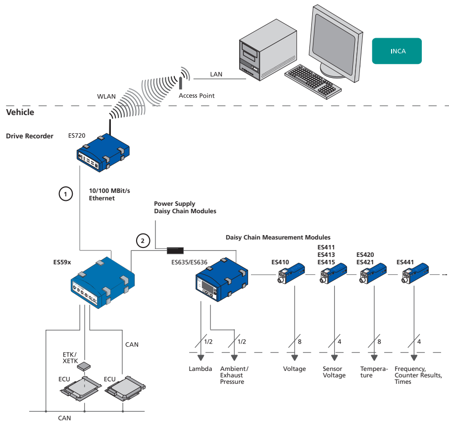
Abb. 5-17 ES400 Module mit weiteren ETAS Modulen und Drive Recorder (Measurement and Calibration)
