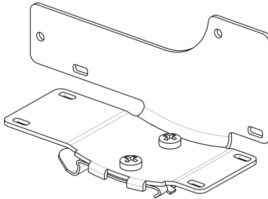
Abb. 8-24 ES4xx-Haltewinkel rechts
