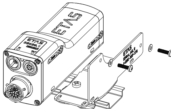
Abb. 5-11 Befestigung an Hutschienen mit zusätzlichen Schrauben
