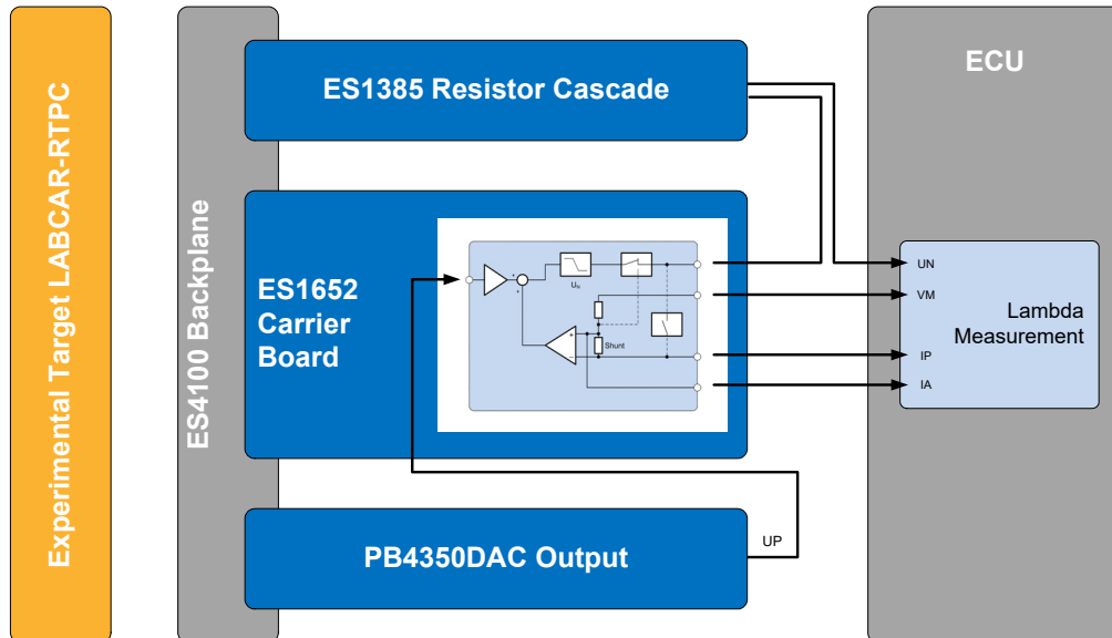
Abb. 1-1 Lambdasondensimulation im HIL-System
