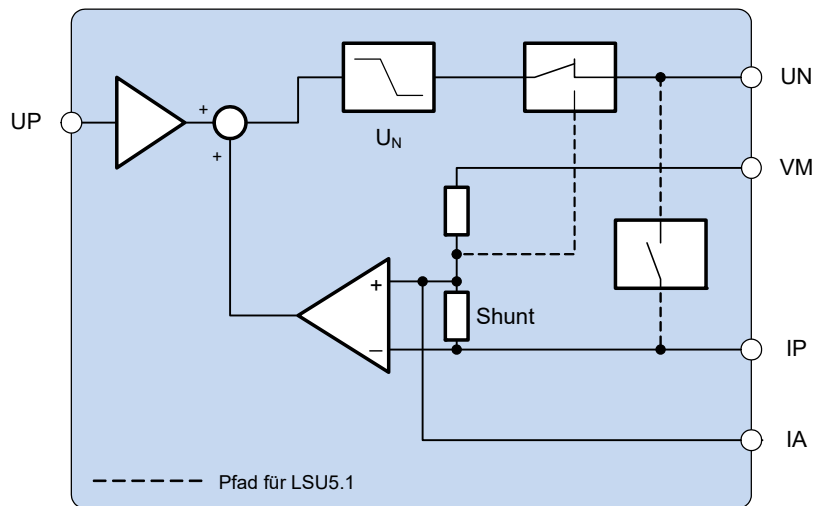
Abb. 1-2 Blockdiagramm des PB1652LAMBDA.1-B
